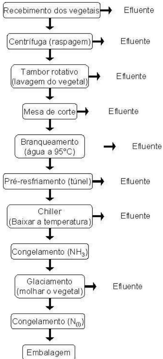
Figura 2: Fluxograma processamento de cenoura com geração de efluentes em cada etapa
