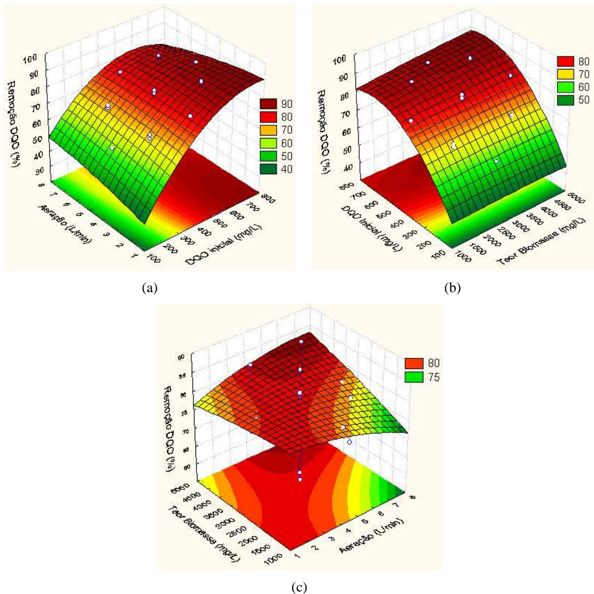
Figura 10: Superfície de resposta para remoção de DQO, utilizando as variáveis: (a) aeração e DQO inicial, (b) DQO inicial e teor de biomassa e (c) teor de biomassa e aeração.
