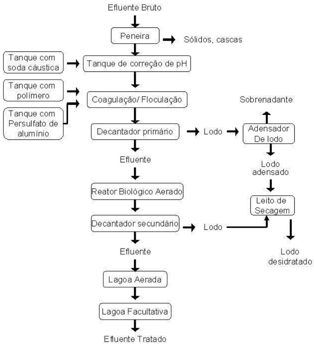
Figura 7: Fluxograma da ETE
