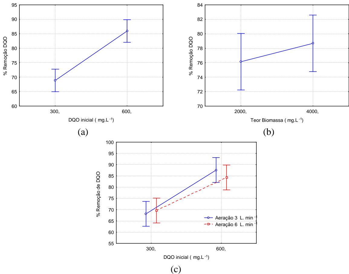
Figura 9: Gráfico das médias para remoção de DQO, utilizando as variáveis: (a) DQO inicial, (b) Teor de biomassa e (c) Interação entre DQO inicial e aeração.
