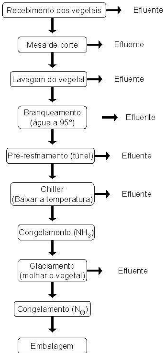
Figura 1: Fluxograma processamento de brócolis e couve-flor com geração de efluentes em cada etapa FONTE: Adaptado de GIL et al., 2009
