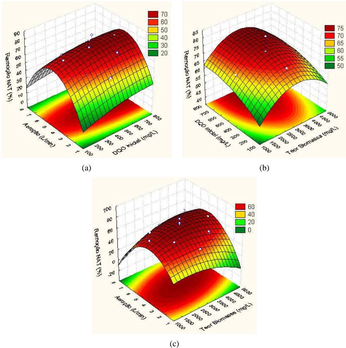
Figura 11: Superfície de resposta para remoção de NAT, utilizando as variáveis: (a) aeração e DQO inicial, (b) DQO inicial e teor de biomassa e (c) aeração e teor de biomassa.
