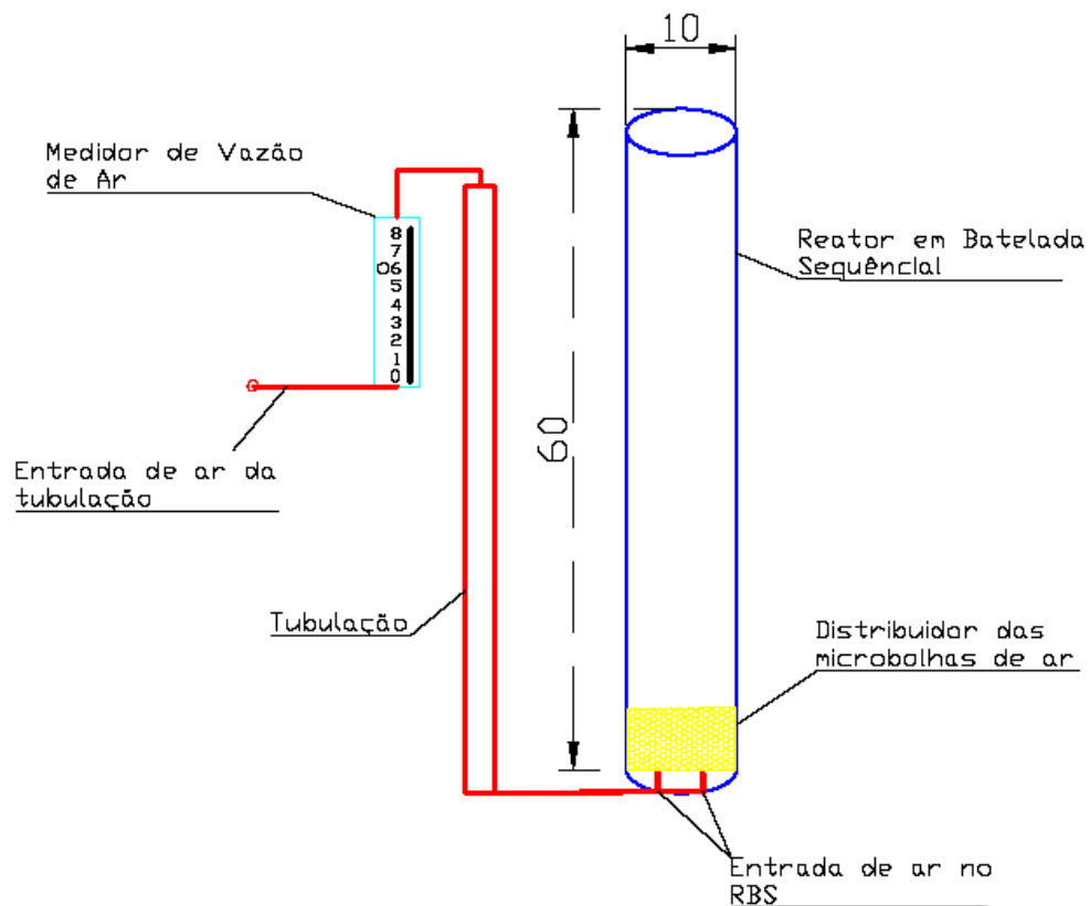
Figura 4: Esquema de montagem do reator RBS.
