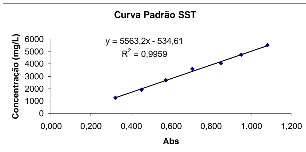
Figura 12: Curva Padrão de SST do lodo utilizado no reator
