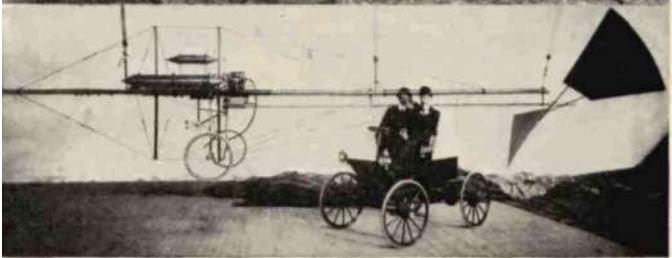
Motor of "No. 4"
