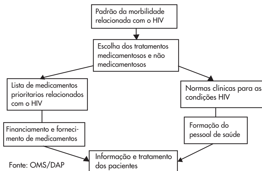
Figura 1. O padrão da morbilidade relacionada com o HIV que deve guiar a selecção, a formação, o fornecimento e uso de medicamentos a nível local.
