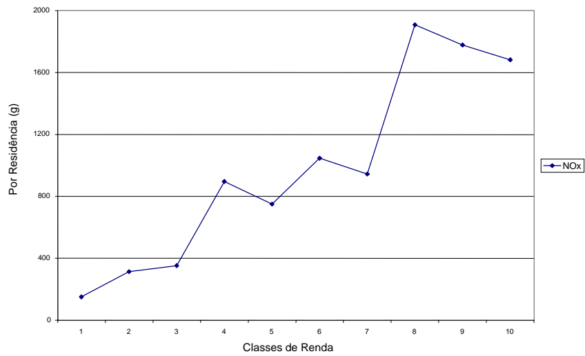
Gráfico 16 Transporte Urbano (NOx)
