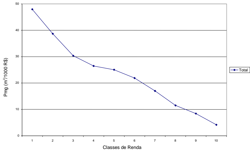
Gráfico 27 Geração de Esgoto (Total)
