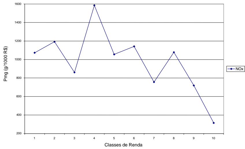
Gráfico 15 Transporte Urbano (NOx)
