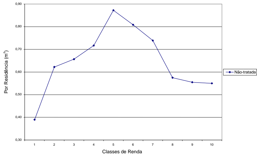
Gráfico 26 Consumo de Água (Não-tratada)
