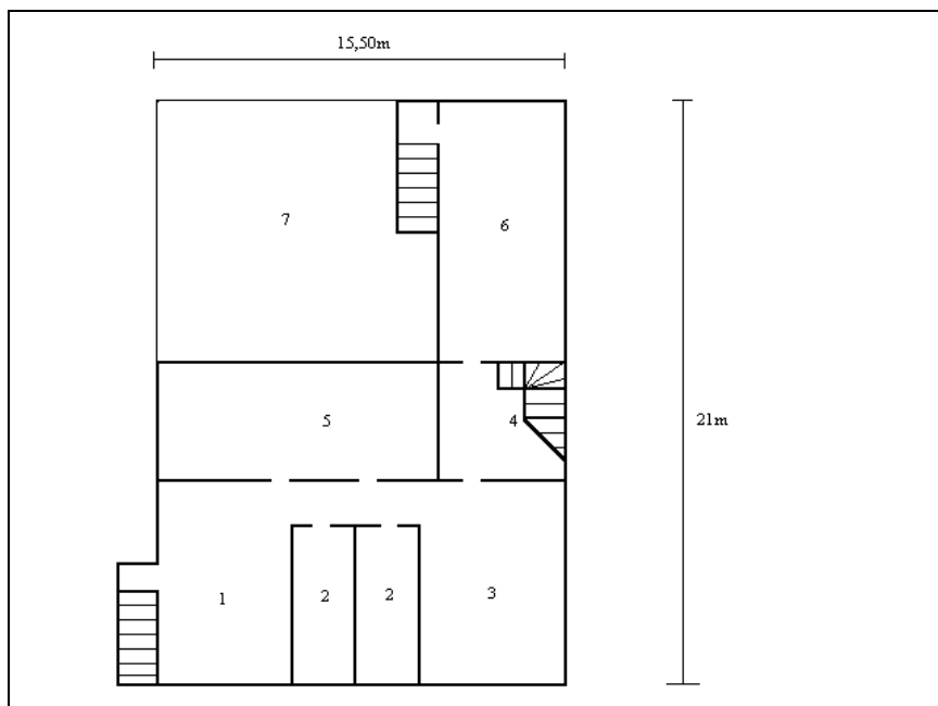
Planta 1. - Compartmentação do Solar Lopo Gonçalves e suas etapas de ampliação: 1- sala de visitas, 2- alcovas, 3- sala de jantar (construção original); 4- recinto que dá acesso ao torreão (primeira etapa de ampliação); 5- varanda (segunda etapa de ampliação); 6- recinto transversal (terceira etapa de ampliação); 7- pátio interno.
