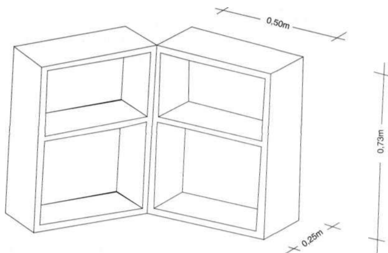
Figura 2 - Caixa-estante aberta
