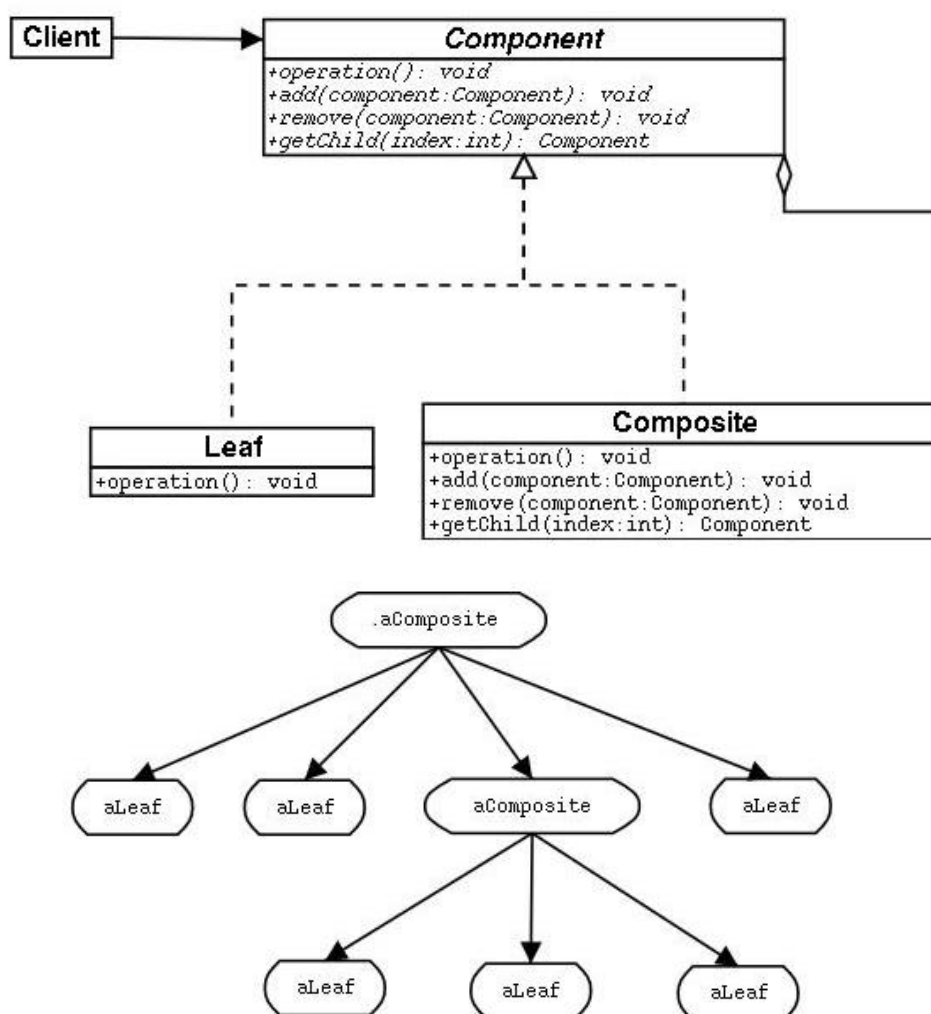
Figura 3.4 O padrão Composite pode representar a estrutura utilizada no GRS
