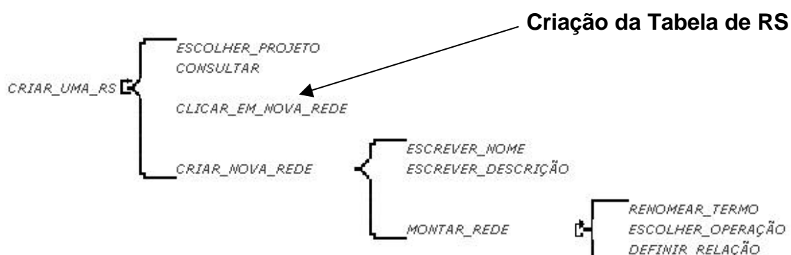
Figura 3.1 Processo de criação de redes sistêmicas no GRS
