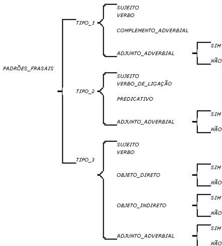
Figura 2.10 Rede Sistemática baseada em padrões frasais
