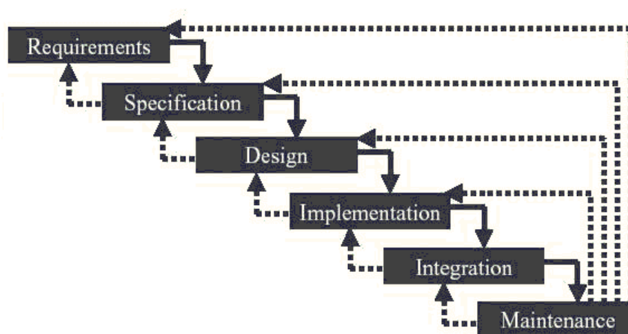
Figura 3.3 Modelo Cascata Modificada
