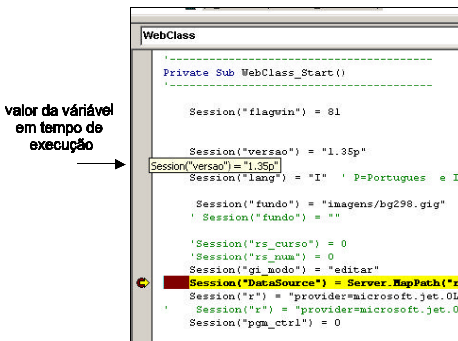
Figura 3.5 Break point e valor da variável em tempo de execução
