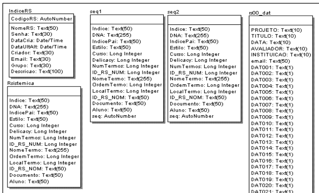
Figura 3.6 Tabelas do Projeto GRS
