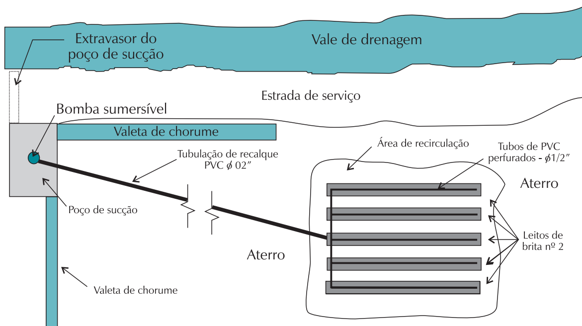
Figura 42 – Recirculação por leito de infiltração
