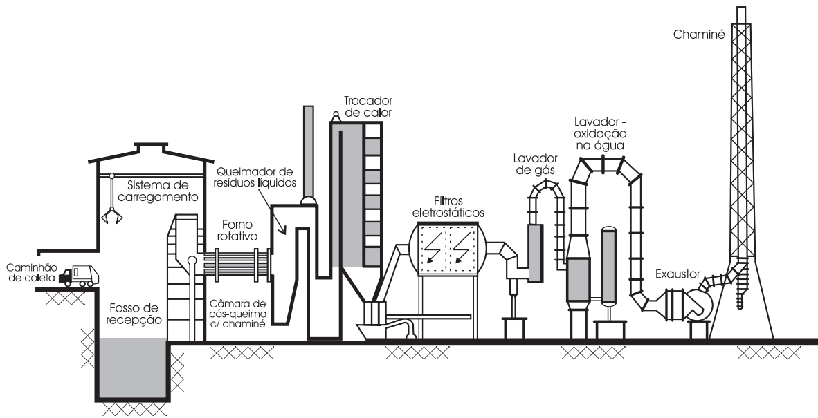
Figura 30 – Incinerador rotativo
