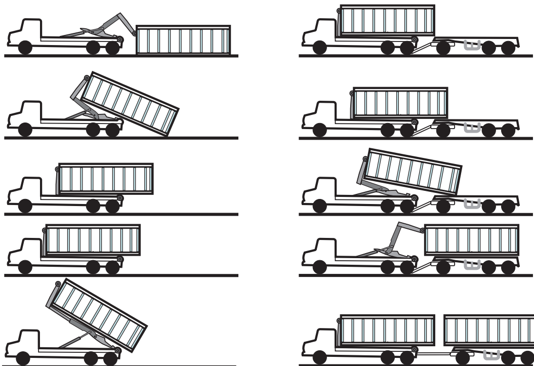
Figura 10 – Caminhão coletor tipo Roll-On/Roll-Off
