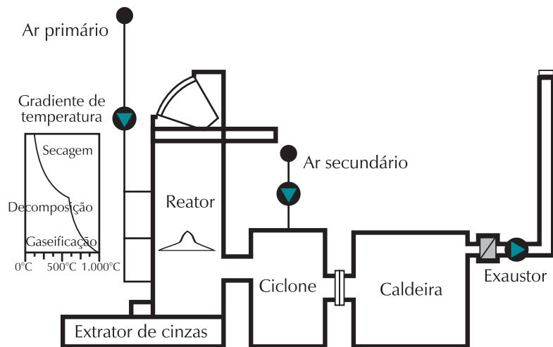
Figura 31 – Pirolisador
