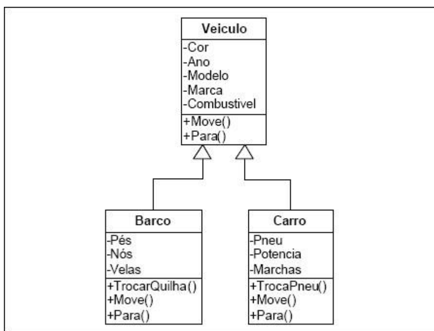
Figura 3.3.1 – Generalização das classes Barco e Carro em superclasse Veículo. Fonte: BOSCARIOLI, 2006.
