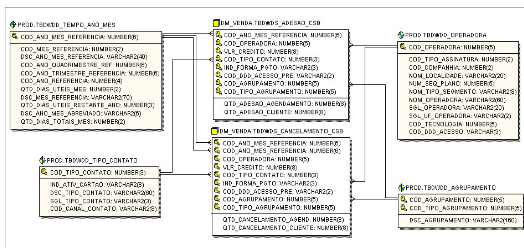
Figura 4.2.1 – Modelo dimensional CSB. Fonte: Adaptado de Core Synesis, 2008.
