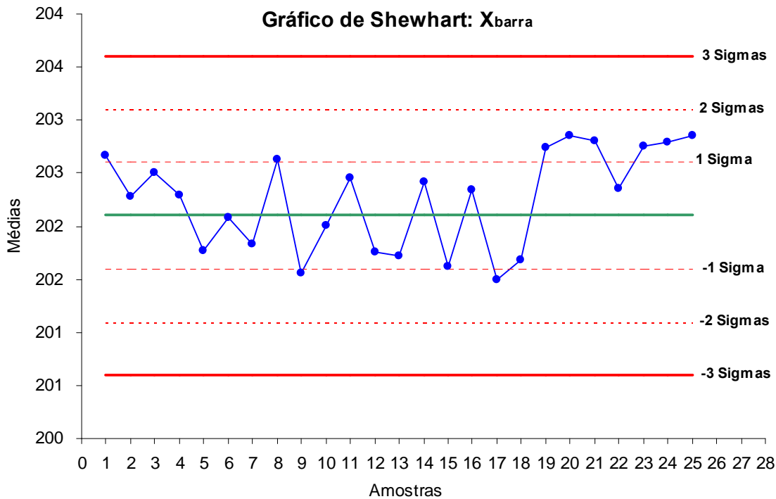
Figura 4.5 Gráfico \bar{X} de Shewhart da semana 3 (Processo: PA)
