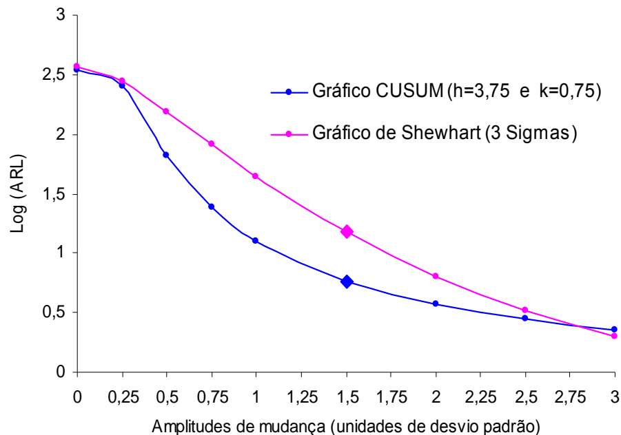
Figura 4.22 Desempenho de ARL dos Gráficos CUSUM e de Shewhart ( X_i ) do Processo PB (Semana 5-2)
