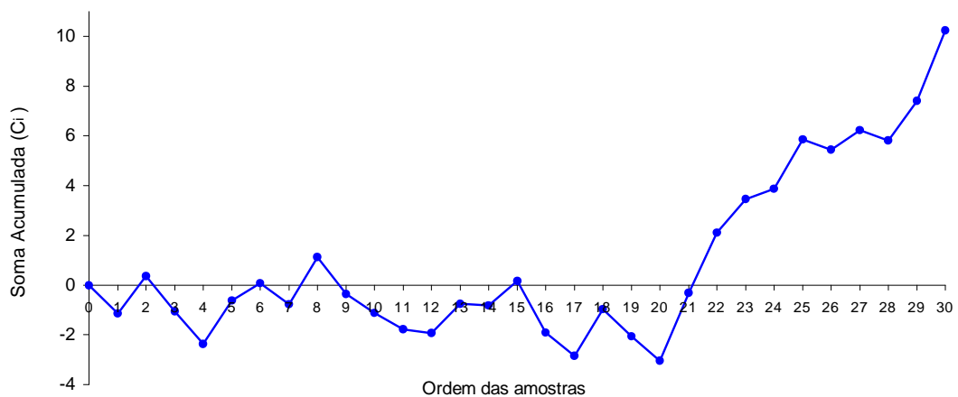
Figura 3.11 Gráfico de Controle Cusum para os dados da tabela 3.12
