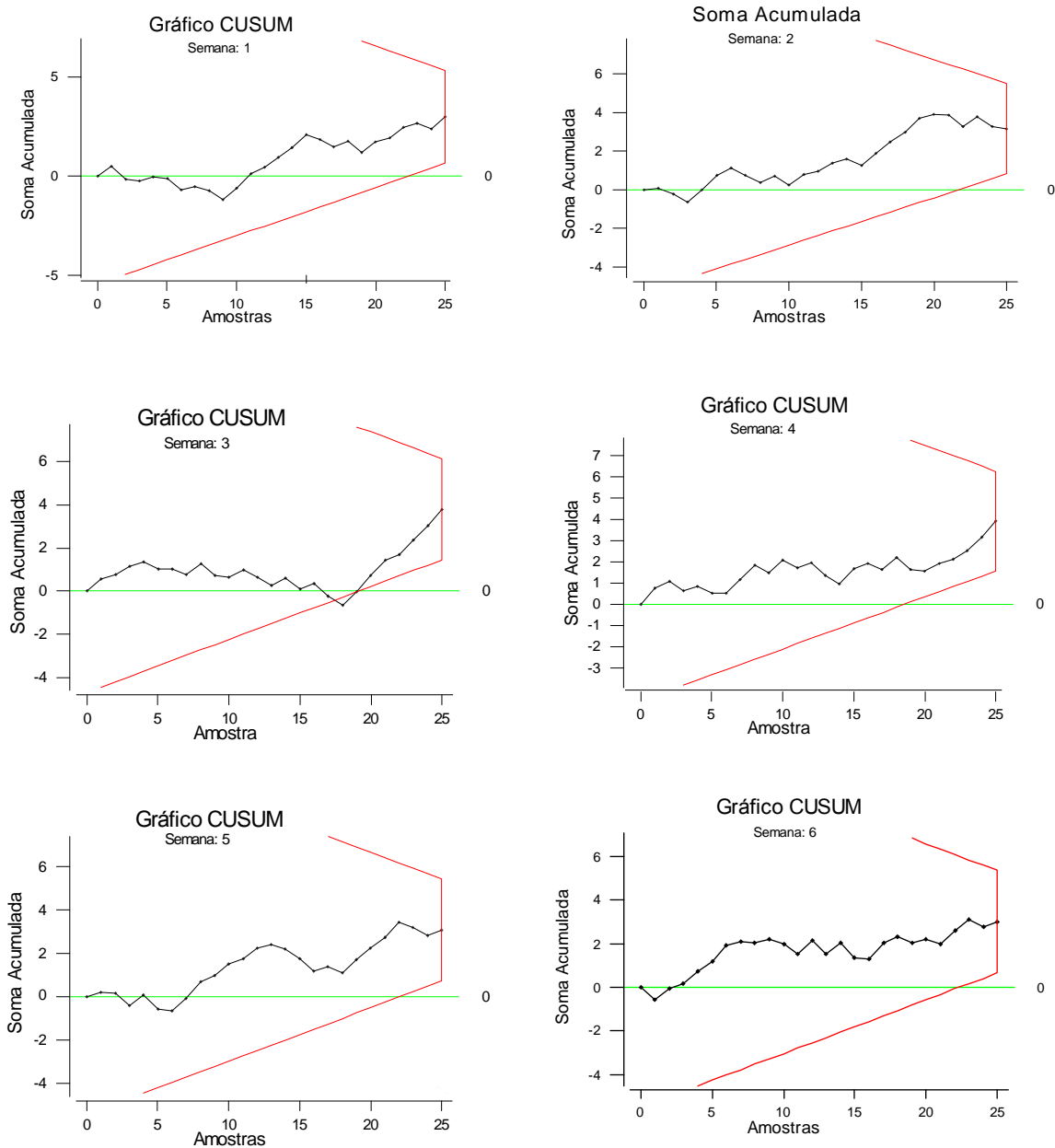
Figura 4.4 Gráficos CUSUM de todas as semanas de análise do processo PA
