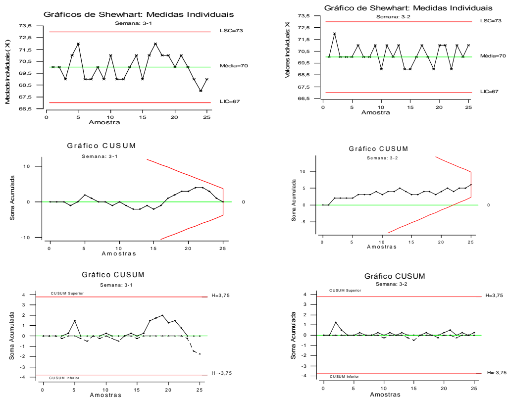
Figura 4.12 Gráficos de Shewhart ( X_i ) e CUSUM do Processo PB (Semana 3)
