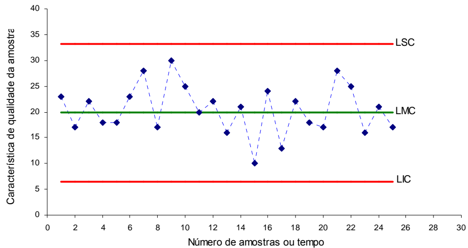
Figura 2.3 Gráfico de controle típico
