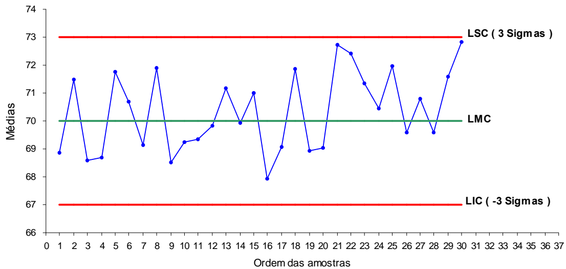
Figura 3.10 Gráfico de Controle de Shewhart para a média: \bar{X}
