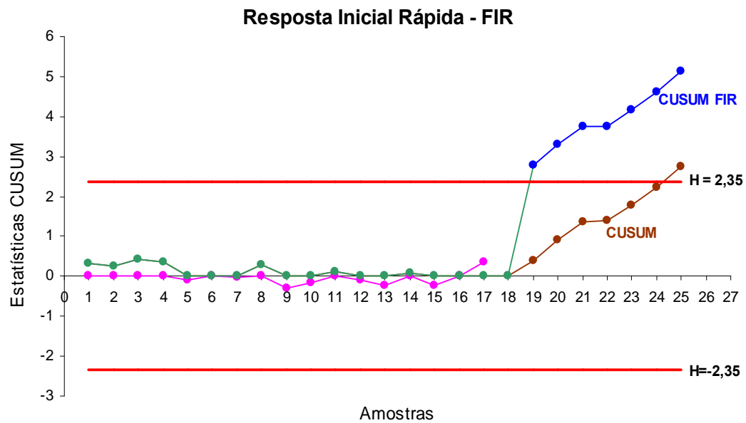
Figura 4.8 Planos de Decisão CUSUM e CUSUM FIR do Processo PA (Semana 3 )
