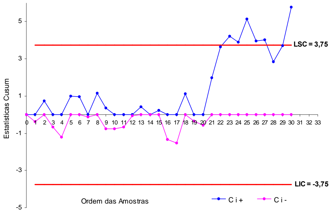
Figura 3.13 Gráfico CUSUM Tabular das estatísticas ( C_i^+ e C_i^- )
