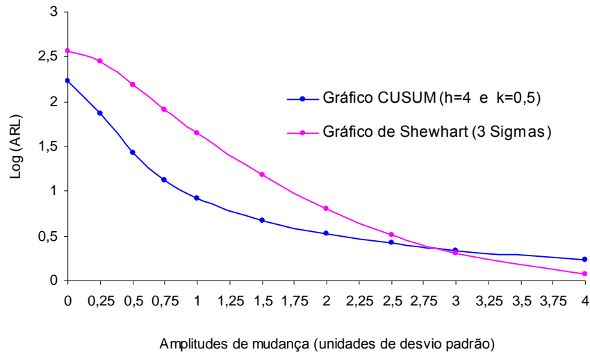
Figura 3.4 Desempenho de ARL dos gráficos: CUSUM (Máscara V) e Shewhart ( 3\sigma )
