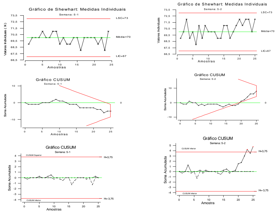
Figura 4.14 Gráficos de Shewhart ( X_i ) e CUSUM do Processo PB (Semana 5)
