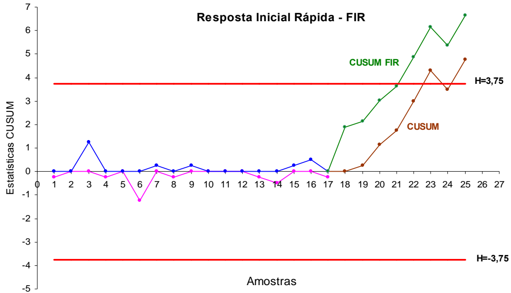
Figura 4.19 Planos de Decisão CUSUM e CUSUM FIR do Processo PB (Semana 5-2)
