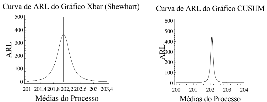
Figura 4.9 Curvas de ARL dos Gráficos \bar{X} (Shewhart) e CUSUM do Processo PA (Semana3)
