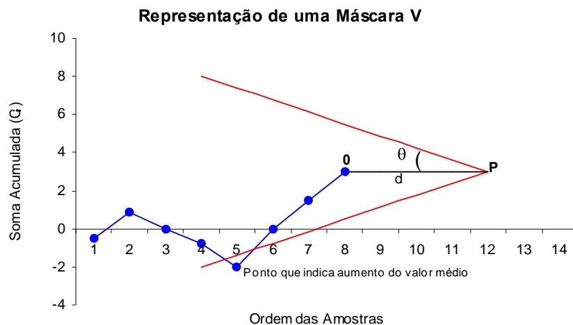
Figura 3.2 Exemplo de Máscara V
