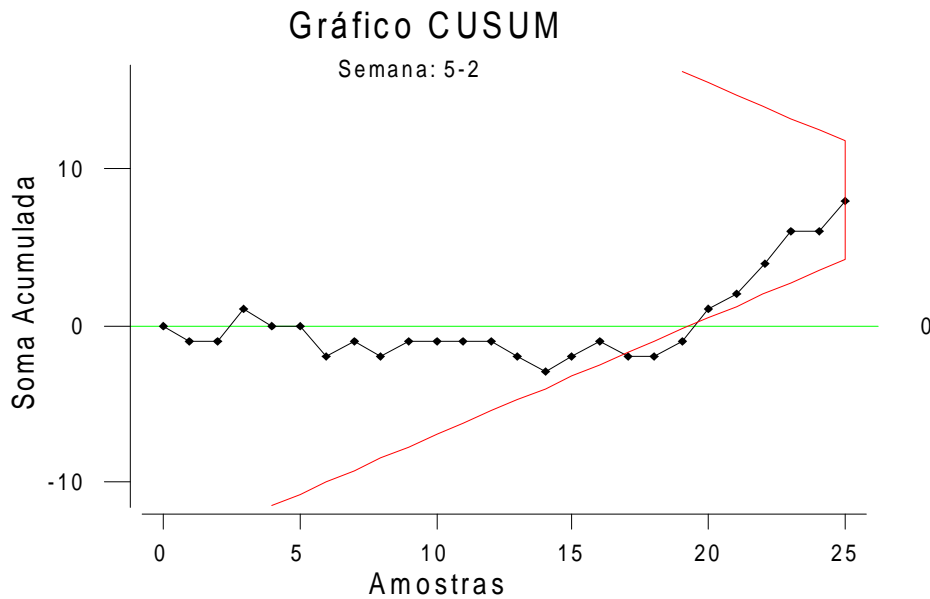
Figura 4.17 Gráfico CUSUM do Processo PB (Semana 5-2 )
