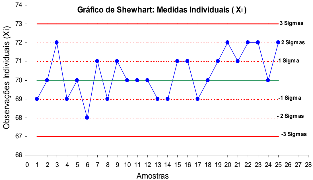
Figura 4.16 Gráfico X_i (Medidas Individuais) de Shewhart do Processo PB (Semana 5-2)
