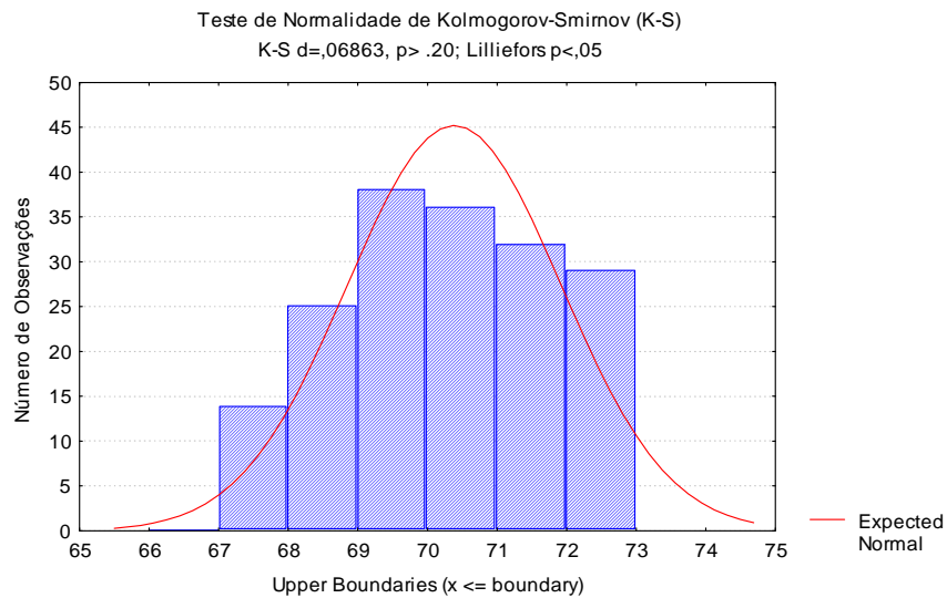
Figura 3.9 Teste de Kolmogorov-Smirnov para os dados da tabela 3.11
