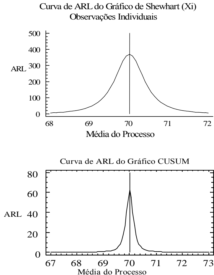
Figura 4.21 Curvas de ARL dos Gráficos de Shewhart ( X_i ) e CUSUM do Processo PB (Semana 5-2)
