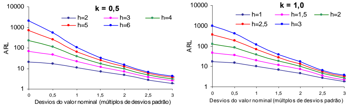
Figura 3.3 Comparativo dos valores de ARL para projetos de Soma Acumulada com valores de referência k (0,5 e 1,0 ) e alguns intervalos de decisão h
