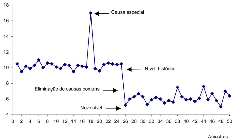
Figura 2.1 Causas comuns e causas especiais de variação
