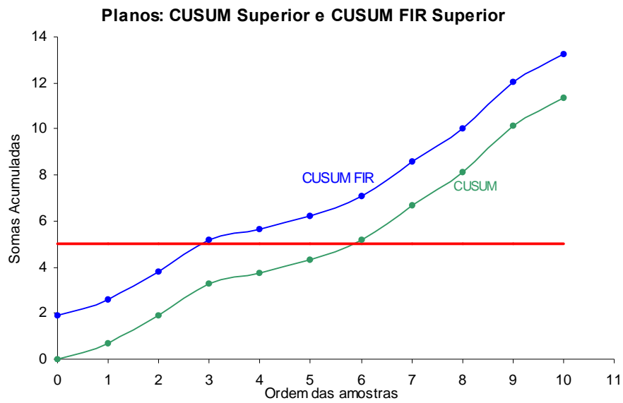
Figura 3.7 Exemplo dos projetos CUSUM e CUSUM FIR
