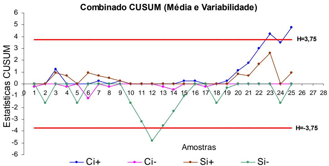
Figura 4.20 Gráfico CUSUM das Estatísticas C_i e S_i do Processo PB (Semana 5-2)
