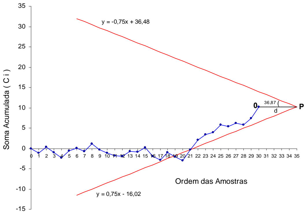
Figura 3.12 Gráfico CUSUM com a utilização da Máscara V para os dados da tabela 3.12
