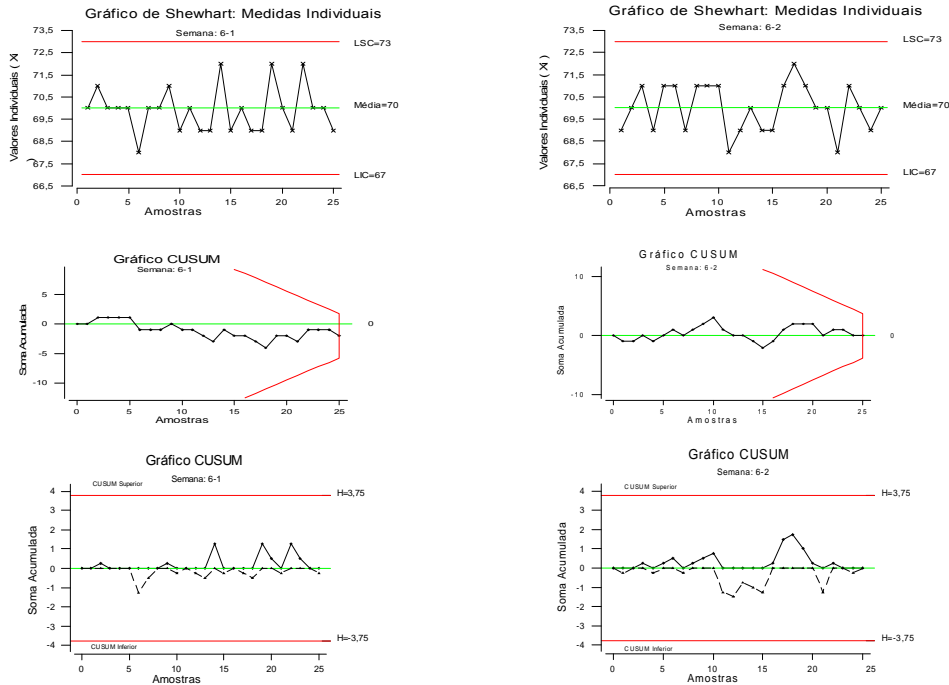
Figura 4.15 Gráficos de Shewhart ( X_i ) e CUSUM do Processo PB (Semana 6)
