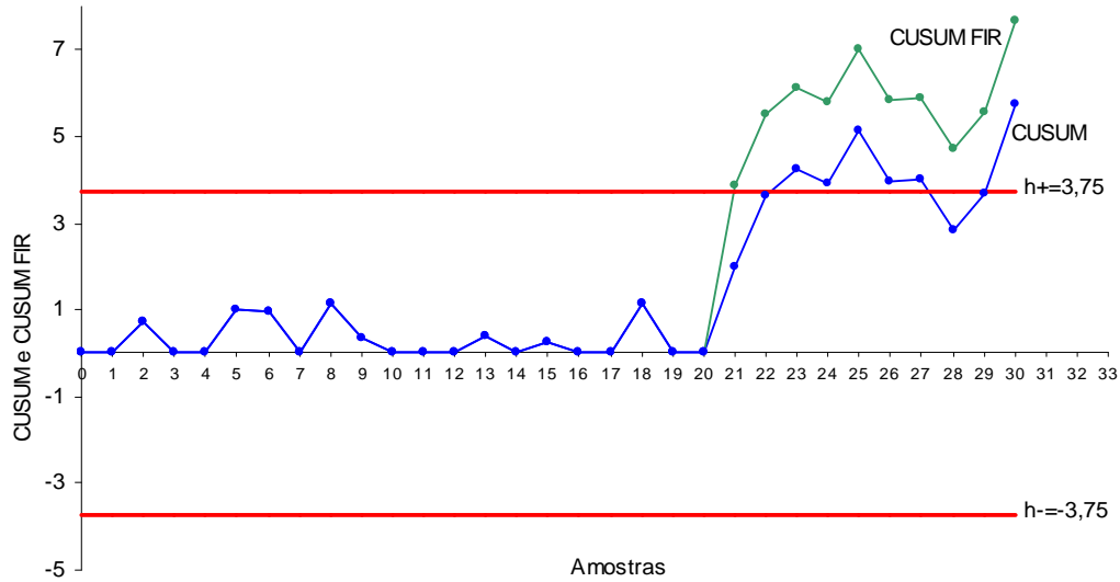
Figura 3.14 Gráfico CUSUM Tabular (CUSUM Superior e CUSUM FIR Superior)
