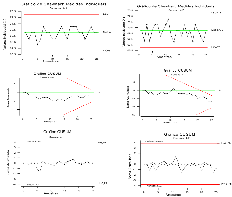
Figura 4.13 Gráficos de Shewhart ( X_i ) e CUSUM do Processo PB (Semana 4)
