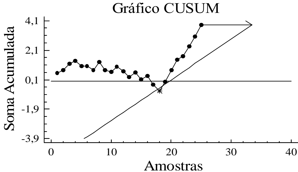
Figura 4.6 Gráfico CUSUM do Processo PA ( Semana 3 )
