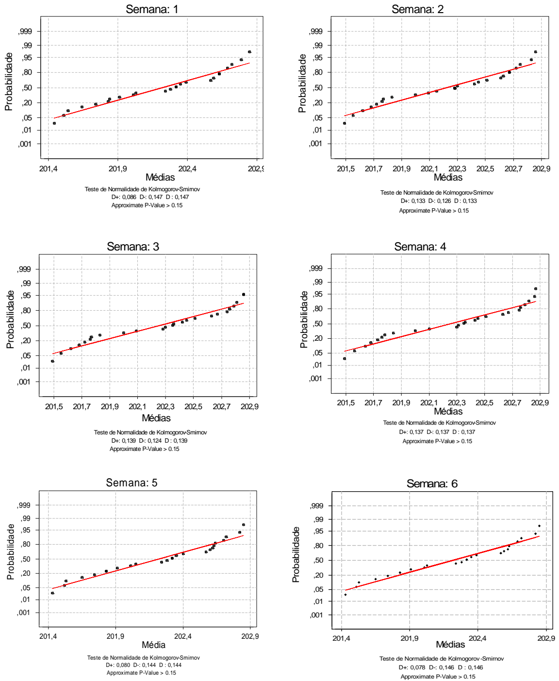
Figura 4.3 Teste Normalidade de todas as semanas de análise do processo PA
