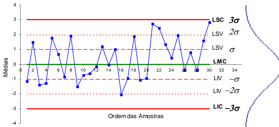
Figura 2.4 Gráfico de controle 3\sigma (três sigmas)
