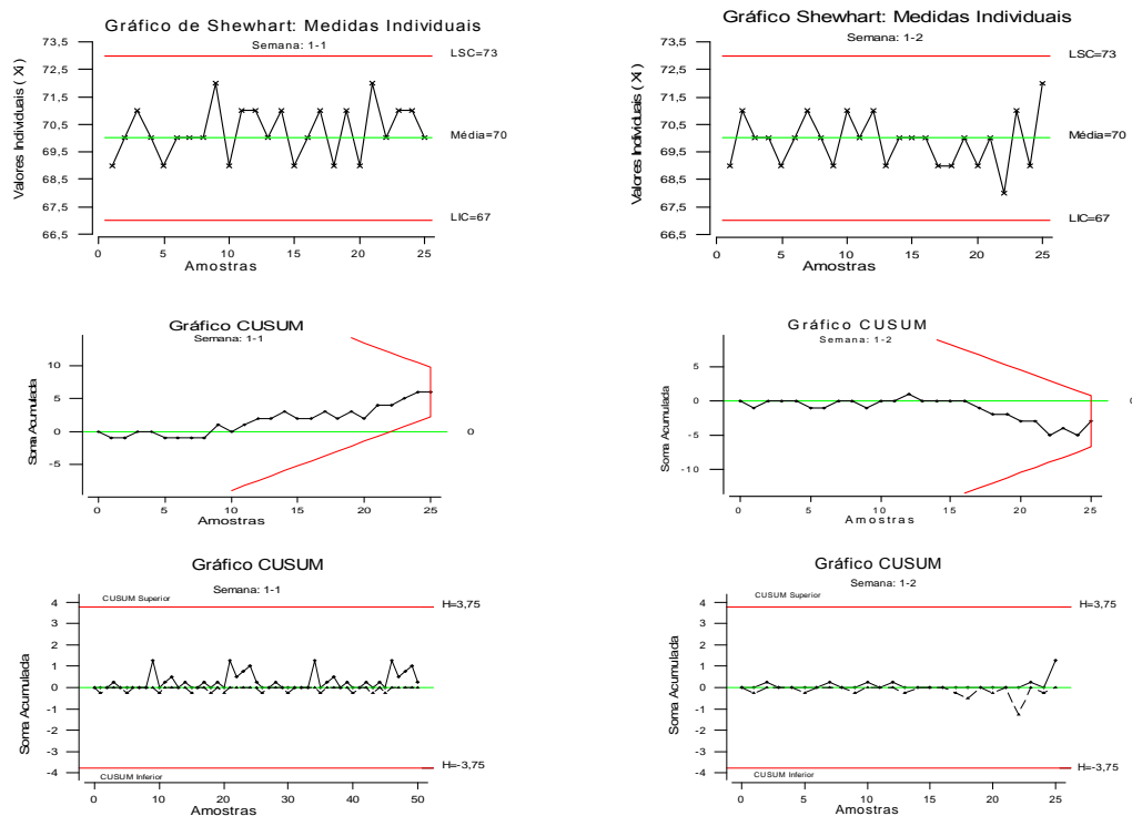
Figura 4.10 Gráficos de Shewhart ( X_i ) e CUSUM do Processo PB (Semana 1)
