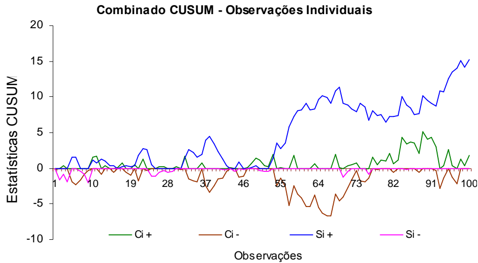
Figura 3.6 Exemplo de gráfico CUSUM com combinado das estatísticas C_i e S_i
