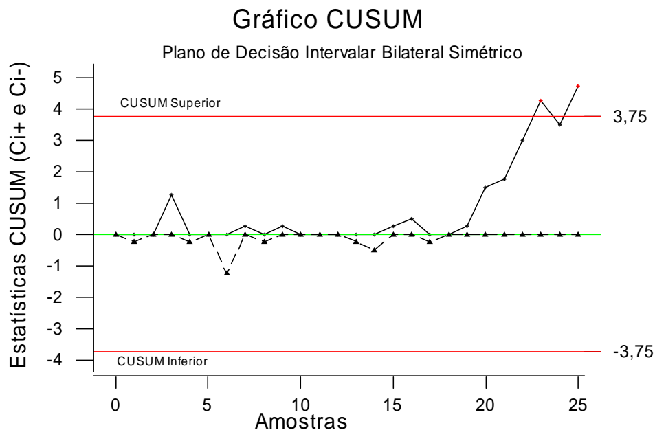
Figura 4.18 Gráfico CUSUM Tabular do Processo PB (Semana 5-2)
