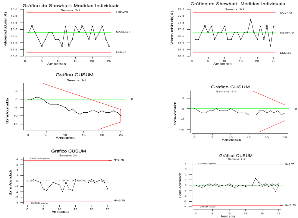
Figura 4.11 Gráficos de Shewhart ( X_i ) e CUSUM do Processo PB (Semana 2)
