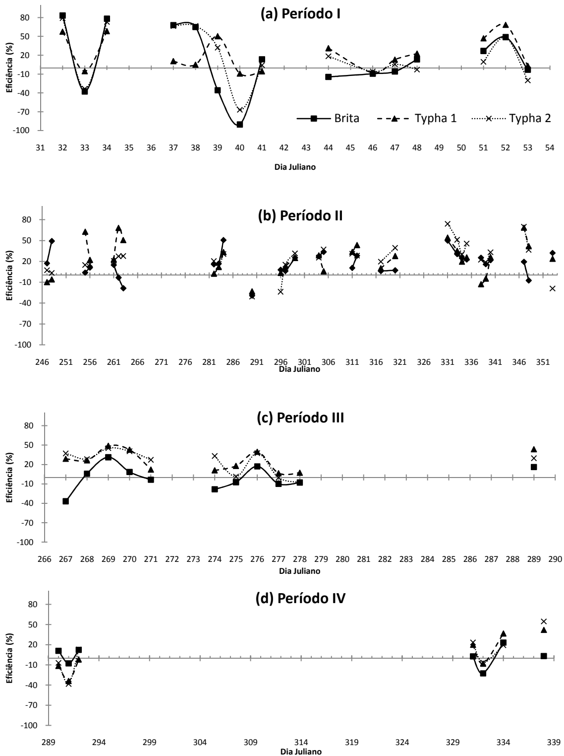
Figura 47. Valor médio da eficiência de retenção de fósforo nos quatro períodos monitorados. Período I (a), Período II (b), Período III (c) e Período IV (d). FEAGRI/UNICAMP, 2006 - 2007. Período I (01 a 22/02/2006), Período II (04/09 a 20/12/2006), Período III (24/09 a 16/10/2007) e Período IV (17/10 a 04/12/2007).
