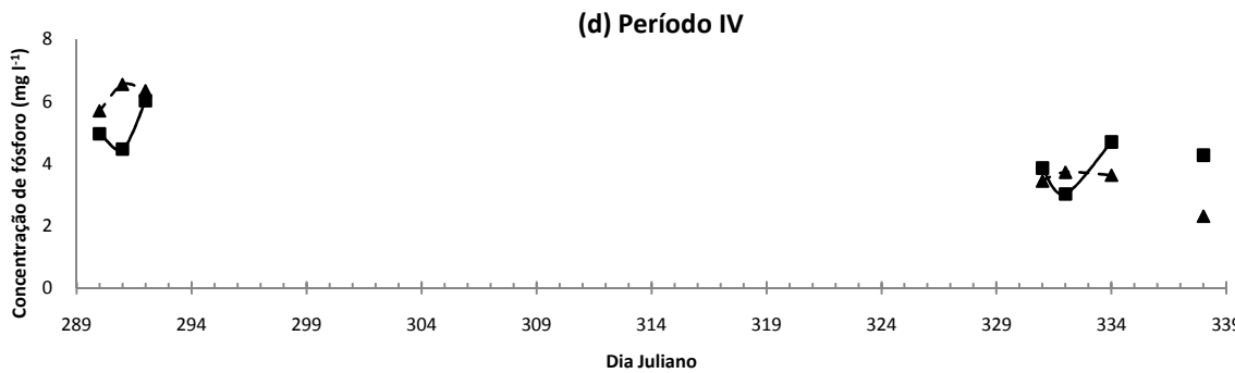
Figura 40. Valor médio de PT_{ed} e PT_{sd} nos quatro períodos monitorados no leito Typha 1. Período I (a), Período II (b), Período III (c) e Período IV (d). FEAGRI/UNICAMP, 2006 - 2007. Período I (01 a 22/02/2006), Período II (04/09 a 20/12/2006), Período III (24/09 a 16/10/2007) e Período IV (17/10 a 04/12/2007).
