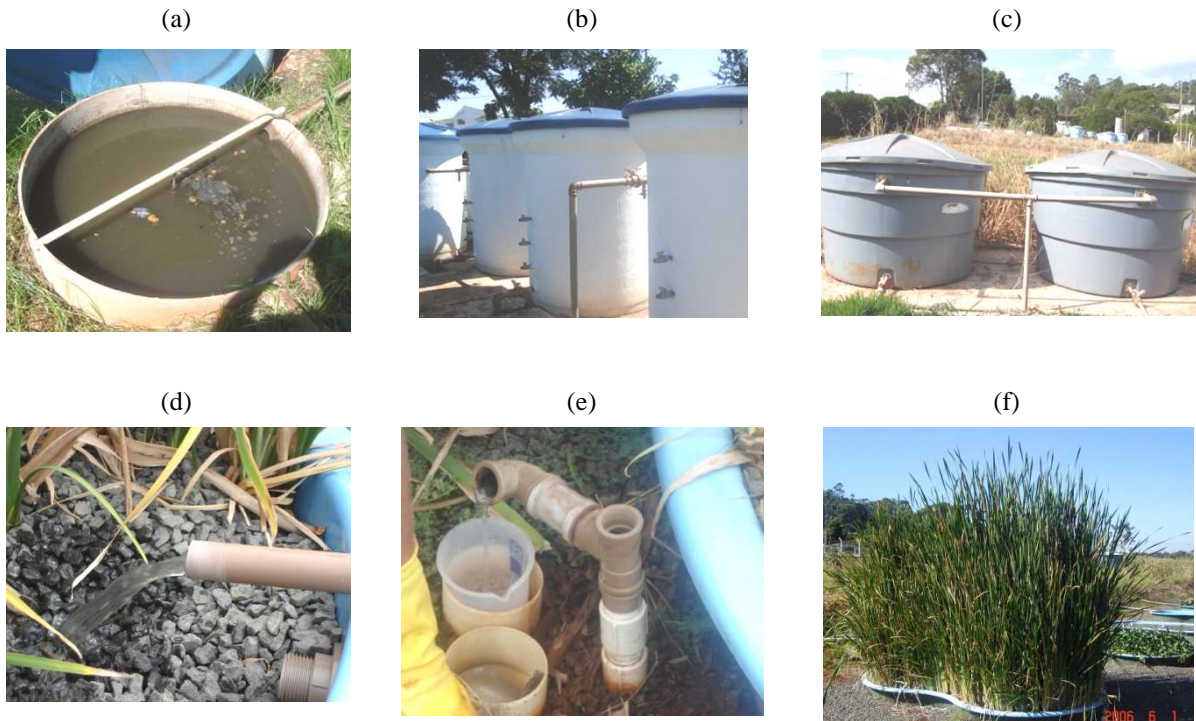
Figura 10. Seqüência percorrida pelo efluente produzido na FEAGRI até a chegada nos leitos cultivados. (a) Efluente bruto; (b) Passagem do efluente pelos RACs; (c) Armazenamento e distribuição do efluente nos reservatórios; (d) Detalhe do dispositivo de entrada do afluente nos leitos cultivados; (e) Detalhe do dispositivo de saída e retirada de amostra do efluente; e (f) Leito cultivado com Typha sp. (FEAGRI/UNICAMP, 2006).
