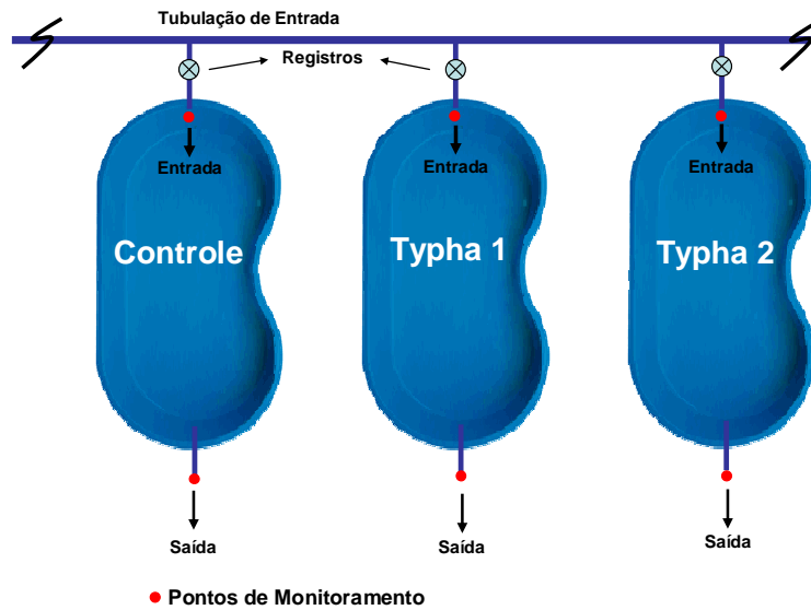
Figura 11. Formato e pontos de monitoramento dos leitos cultivados implantados no Campo Experimental da FEAGRI.
