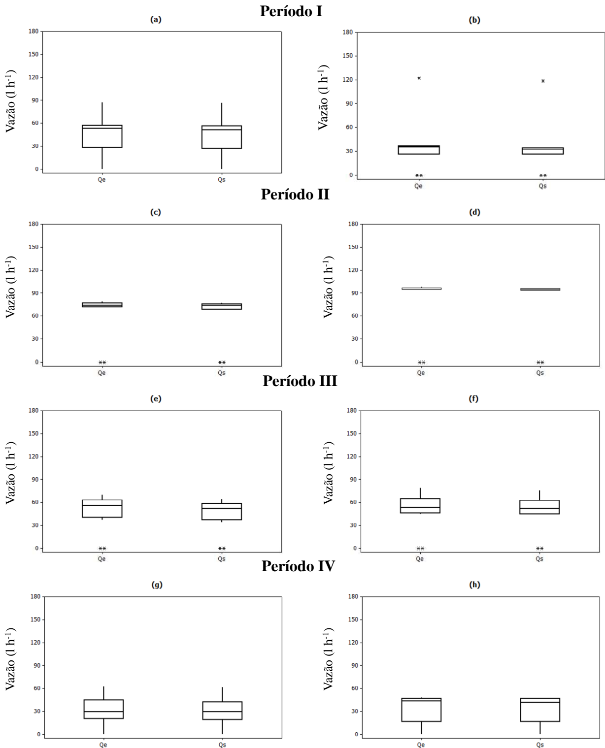
Figura 14. Gráficos “Box Plot” da Q_{eh} e Q_{sh} de dias característicos nos quatro períodos monitorados no leito Brita. Período I: 02/02/2006 (a) e 03/02/2006 (b); Período II: 19/09/2006 (c) e 20/09/2006 (d); Período III: 02/10/2007 (e) e 03/10/2007 (f) e; Período IV: 27/11/2007 (g) e 28/11/2007 (h). FEAGRI/UNICAMP, 2006 - 2007.
