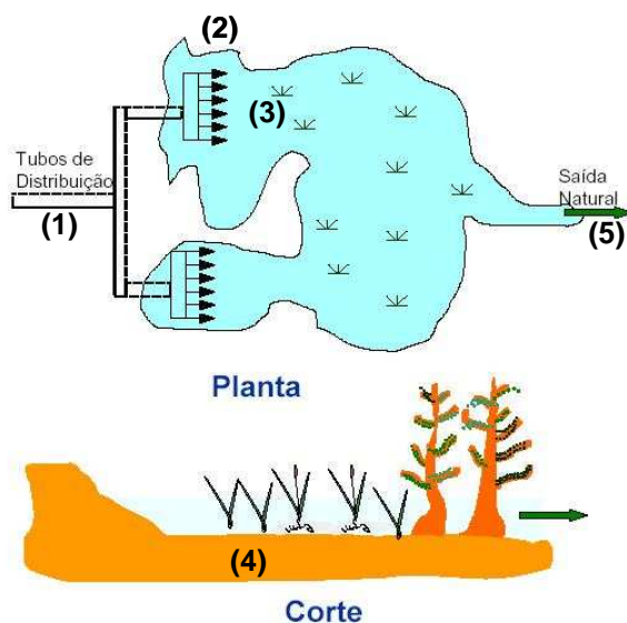
Figura 3. Configuração típica de um wetland natural. Modificado de Kadlec & Knight (1996).
