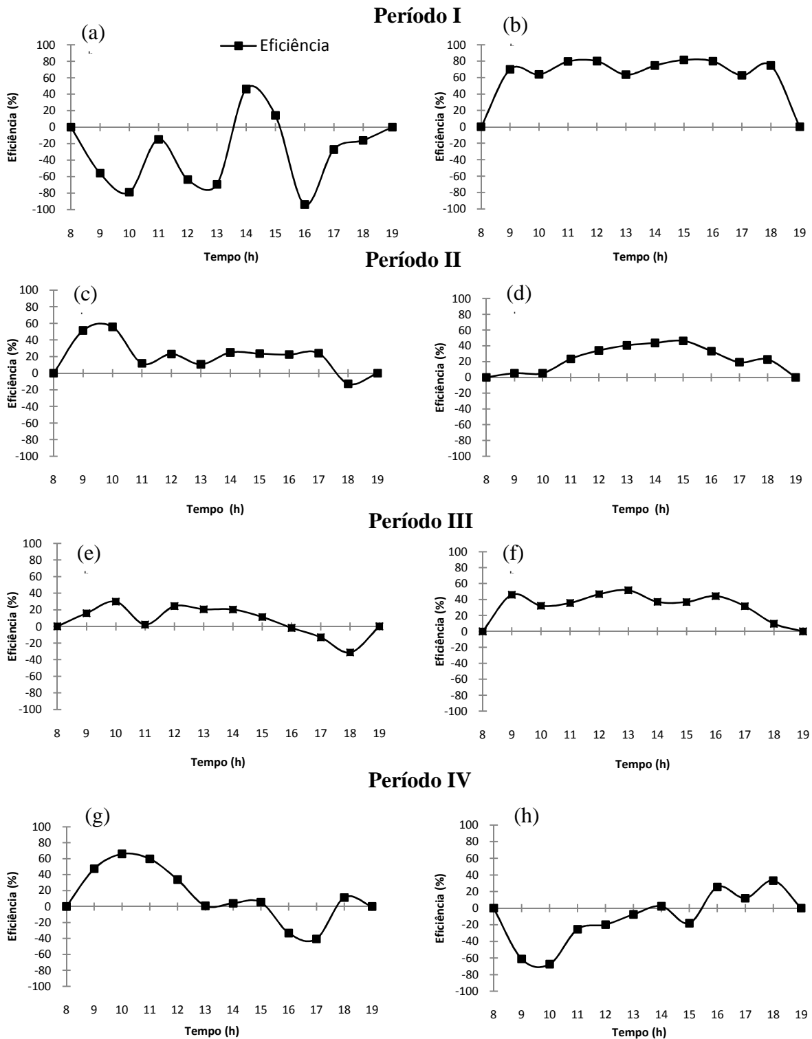
Figura 33. Valor horário da eficiência de retenção de fósforo de dias característicos nos quatro períodos monitorados no leito Typha 2. Período I: 02/02/2006 (a) e 03/02/2006 (b); Período II: 19/09/2006 (c) e 20/09/2006 (d); Período III: 02/10/2007 (e) e 03/10/2007 (f) e; Período IV: 27/11/2007 (g) e 28/11/2007 (h). FEAGRI/UNICAMP, 2006 - 2007.
