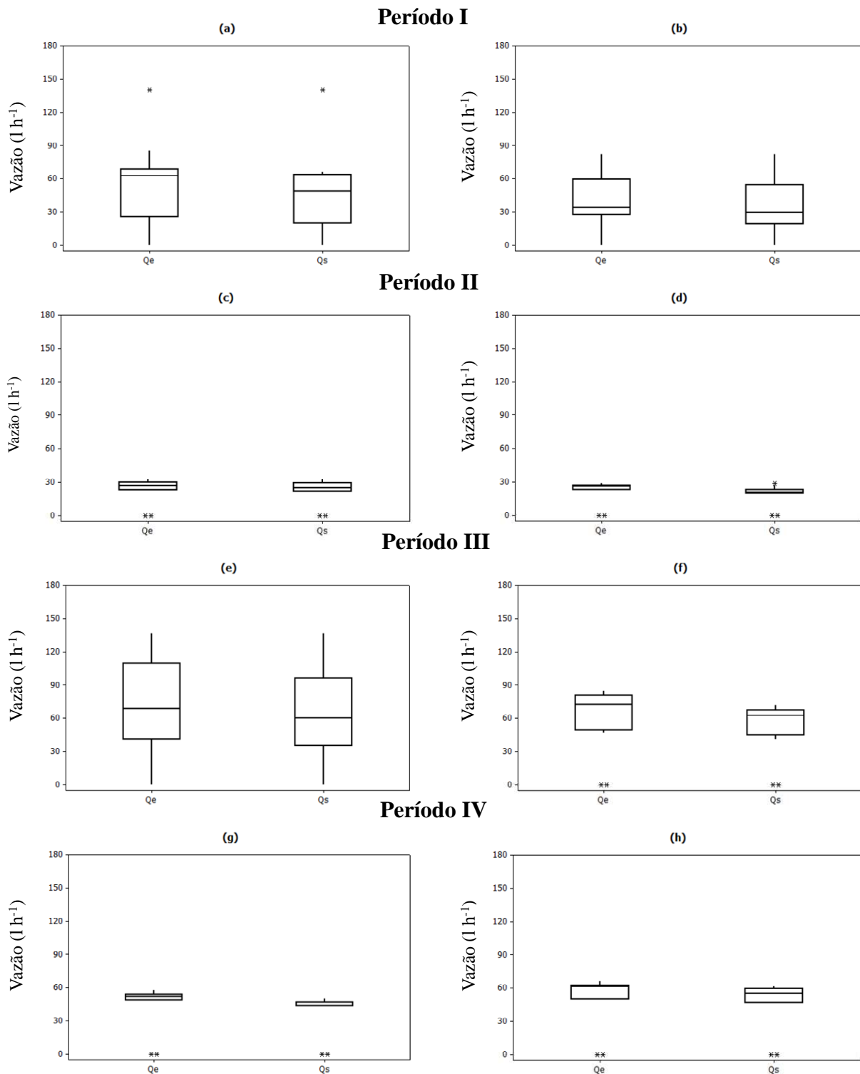
Figura 18. Gráficos “Box Plot” de Q_{eh} e Q_{sh} de dias característicos nos quatro períodos monitorados no leito Typha 2. Período I: 02/02/2006 (a) e 03/02/2006 (b); Período II: 19/09/2006 (c) e 20/09/2006 (d); Período III: 02/10/2007 (e) e 03/10/2007 (f) e; Período IV: 27/11/2007 (g) e 28/11/2007 (h). FEAGRI/UNICAMP, 2006 - 2007.
