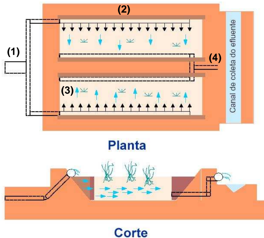
Figura 2. Configuração típica de um leito cultivado de fluxo subsuperficial. Modificado de Kadlec & Knight (1996).
