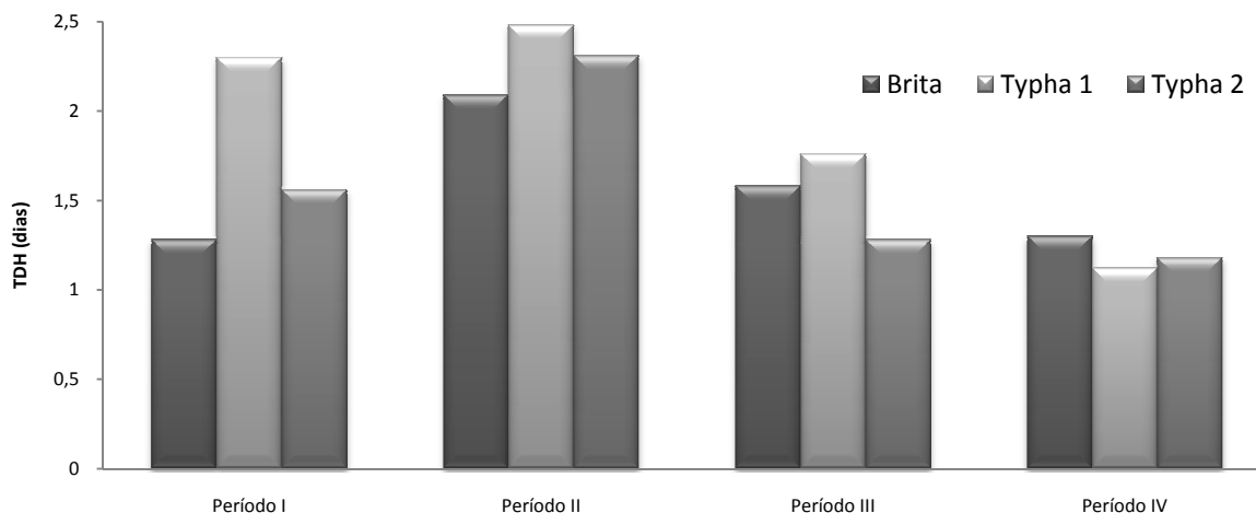
Figura 52. Valor médio do TDH nos quatro períodos monitorados. Período I (01 a 22/02/2006), Período II (04/09 a 20/12/2006), Período III (24/09 a 16/10/2007) e Período IV (17/10 a 04/12/2007). FEAGRI/UNICAMP, 2006 – 2007
