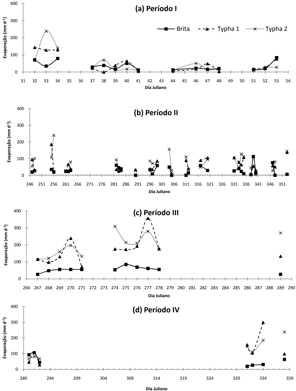
Figura 38. Valor médio do volume evaporado nos quatro períodos monitorados. Período I (a), Período II (b), Período III (c) e Período IV (d). FEAGRI/UNICAMP, 2006 - 2007. Período I (01 a 22/02/2006), Período II (04/09 a 20/12/2006), Período III (24/09 a 16/10/2007) e Período IV (17/10 a 04/12/2007).
