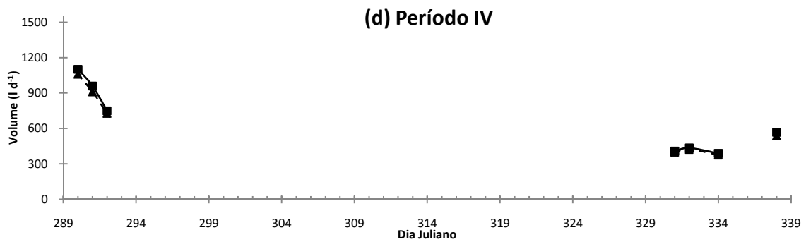
Figura 34. Valor médio diário de V_{ed} e V_{sd} nos quatro períodos monitorados no leito Brita. Período I (a), Período II (b), Período III (c) e Período IV (d). FEAGRI/UNICAMP, 2006 - 2007. Período I (01 a 22/02/2006), Período II (04/09 a 20/12/2006), Período III (24/09 a 16/10/2007) e Período IV (17/10 a 04/12/2007).
