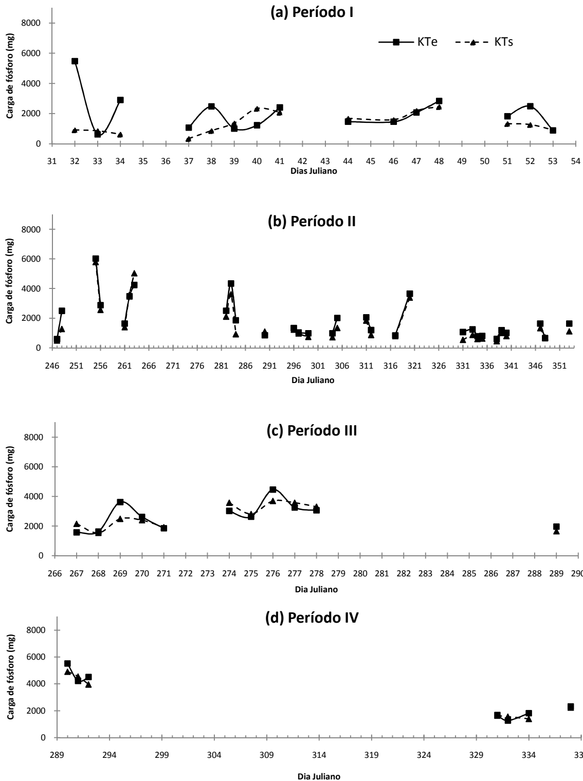
Figura 43. Valor médio de KT_{ed} e KT_{sd} nos quatro períodos monitorados no leito Brita. Período I (a), Período II (b), Período III (c) e Período IV (d). FEAGRI/UNICAMP, 2006 - 2007. Período I (01 a 22/02/2006), Período II (04/09 a 20/12/2006), Período III (24/09 a 16/10/2007) e Período IV (17/10 a 04/12/2007).
