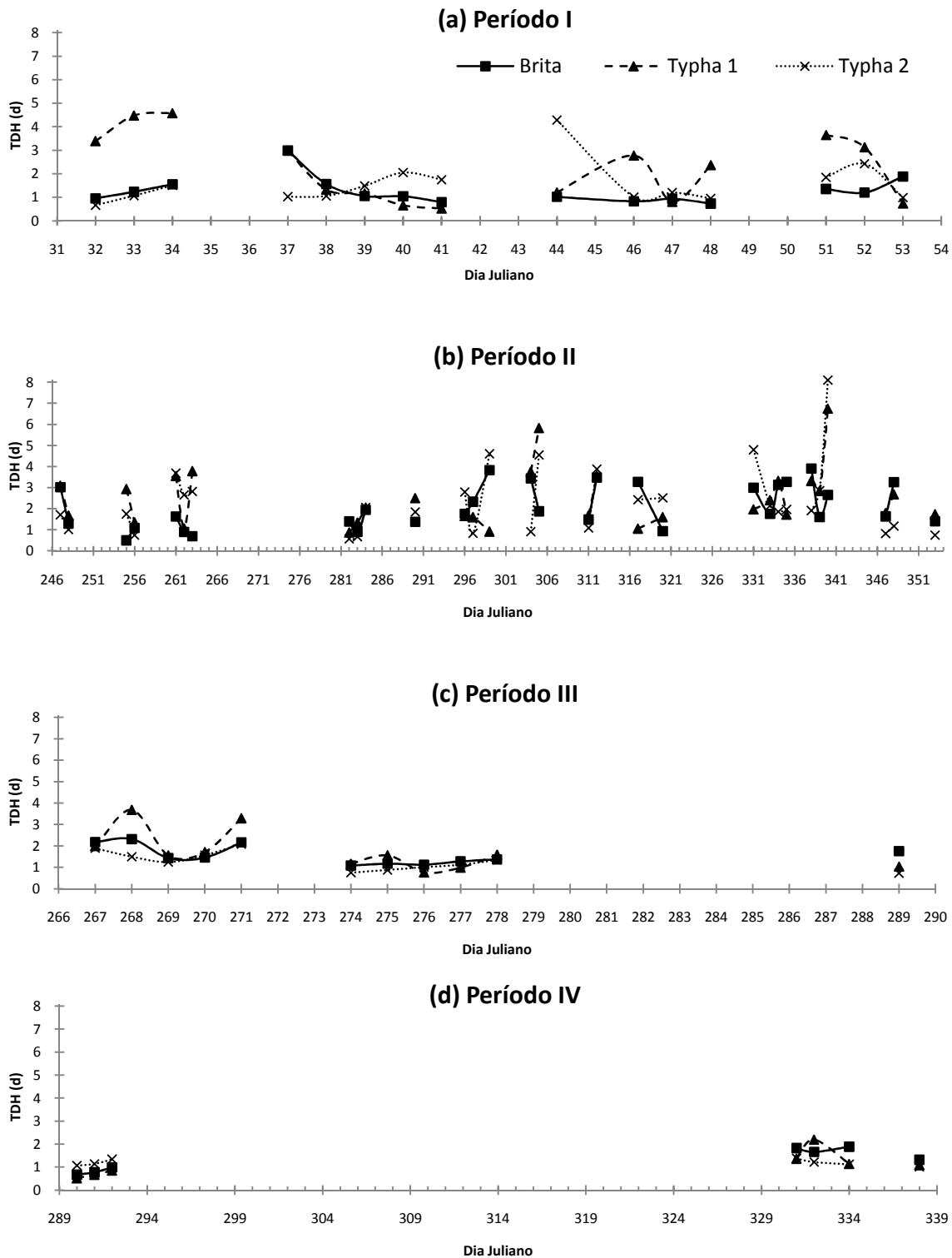
Figura 37. Valor médio do TDH nos quatro períodos monitorados. Período I (a), Período II (b), Período III (c) e Período IV (d). FEAGRI/UNICAMP, 2006 - 2007. Período I (01 a 22/02/2006), Período II (04/09 a 20/12/2006), Período III (24/09 a 16/10/2007) e Período IV (17/10 a 04/12/2007).
