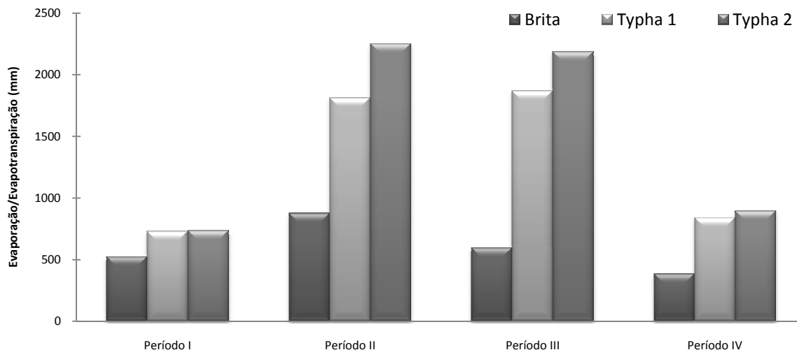
Figura 51. Volume total evaporado/evapotranspirado nos quatro períodos monitorados. Período I (01 a 22/02/2006), Período II (04/09 a 20/12/2006), Período III (24/09 a 16/10/2007) e Período IV (17/10 a 04/12/2007). FEAGRI/UNICAMP, 2006 - 2007.
