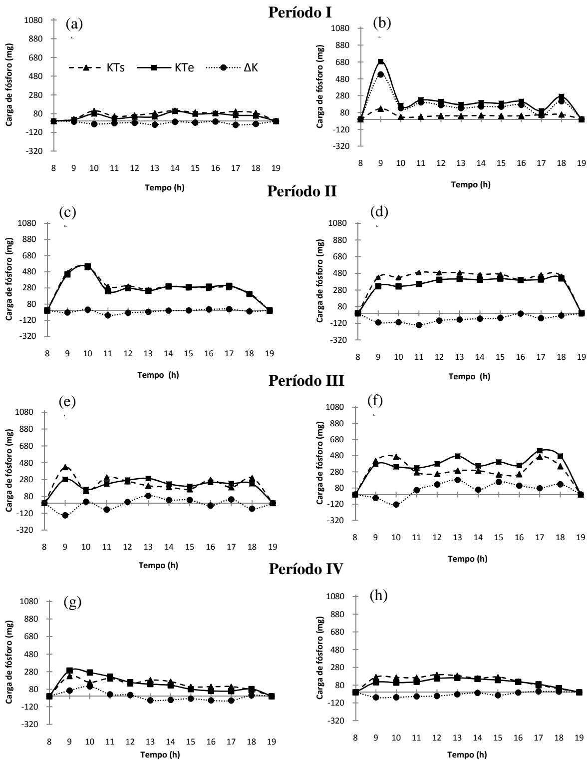
Figura 25. Valor horário de carga de KT_{ch} , KT_{sh} e \Delta KT_h de dias característicos nos quatro períodos monitorados no leito Brita. Período I: 02/02/2006 (a) e 03/02/2006 (b); Período II: 19/09/2006 (c) e 20/09/2006 (d); Período III: 02/10/2007 (e); 03/10/2007 (f) e; Período IV: 27/11/2007 (g) e 28/11/2007 (h). FEAGRI/UNICAMP, 2006 - 2007.
