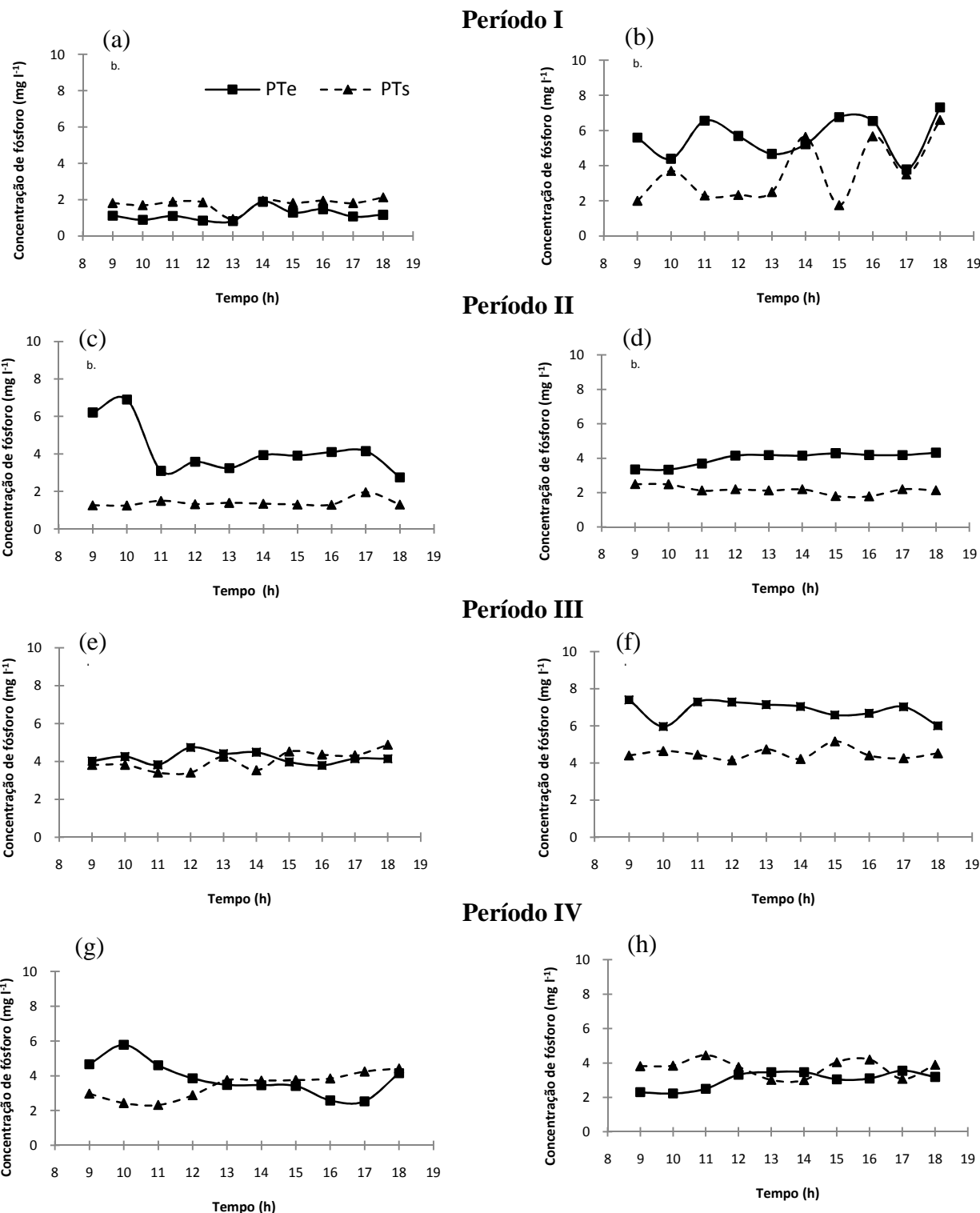
Figura 21. Valor horário de concentração de PT_{eh} e PT_{sh} de dias característicos nos quatro períodos monitorados no leito Typha 1. Período I: 02/02/2006 (a) e 03/02/2006 (b); Período II: 19/09/2006 (c) e 20/09/2006 (d); Período III: 02/10/2007 (e) e 03/10/2007 (f) e; Período IV: 27/11/2007 (g) e 28/11/2007 (h). FEAGRI/UNICAMP, 2006 - 2007.
