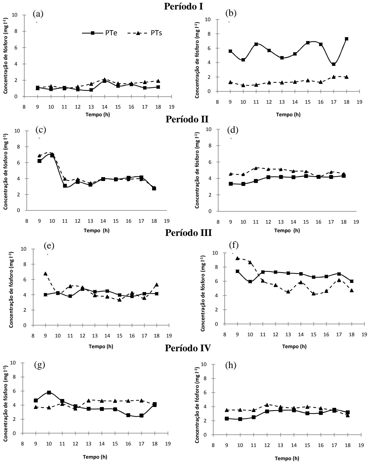
Figura 19. Valor horário de concentração de PT_{ch} e PT_{sh} de dias característicos nos quatro períodos monitorados no leito Brita. Período I: 02/02/2006 (a) e 03/02/2006 (b); Período II: 19/09/2006 (c) e 20/09/2006 (d); Período III: 02/10/2007 (e) e 03/10/2007 (f) e; Período IV: 27/11/2007 (g) e 28/11/2007 (h). FEAGRI/UNICAMP, 2006 - 2007.
