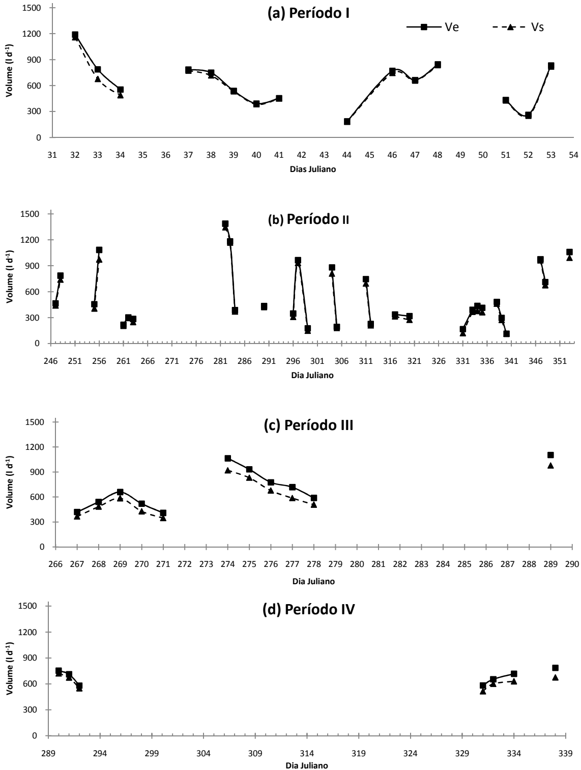
Figura 36. Valor médio diário de V_{ed} e V_{sd} nos quatro períodos monitorados no leito Typha 2. Período I (a), Período II (b), Período III (c) e Período IV (d). FEAGRI/UNICAMP, 2006 - 2007. Período I (01 a 22/02/2006), Período II (04/09 a 20/12/2006), Período III (24/09 a 16/10/2007) e Período IV (17/10 a 04/12/2007).
