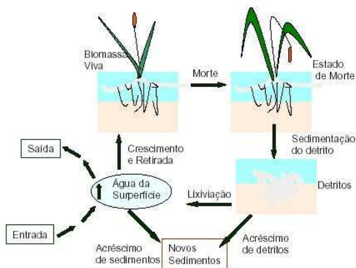
Figura 6. Ciclo do fósforo na biomassa em wetlands (Kadlec & Knight, 1996).
