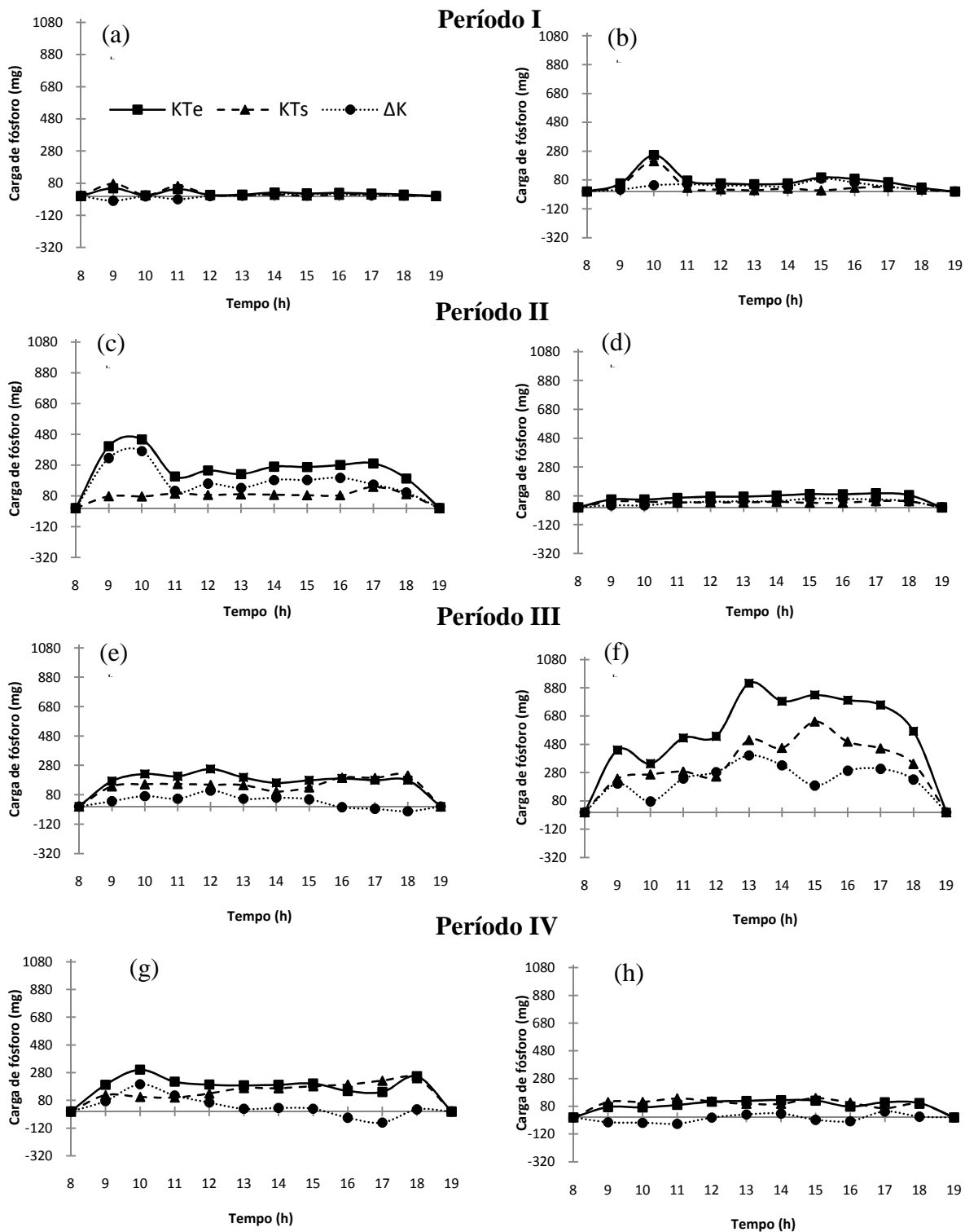
Figura 27. Valor horário de carga de KT_{ch} , KT_{sh} e \Delta KT_h de dias característicos nos quatro períodos monitorados no leito Typha 1. Período I: 02/02/2006 (a) e 03/02/2006 (b); Período II: 19/09/2006 (c) e 20/09/2006 (d); Período III: 02/10/2007 (e) e 03/10/2007 (f) e; Período IV: 27/11/2007 (g) e 28/11/2007 (h). FEAGRI/UNICAMP, 2006 - 2007.
