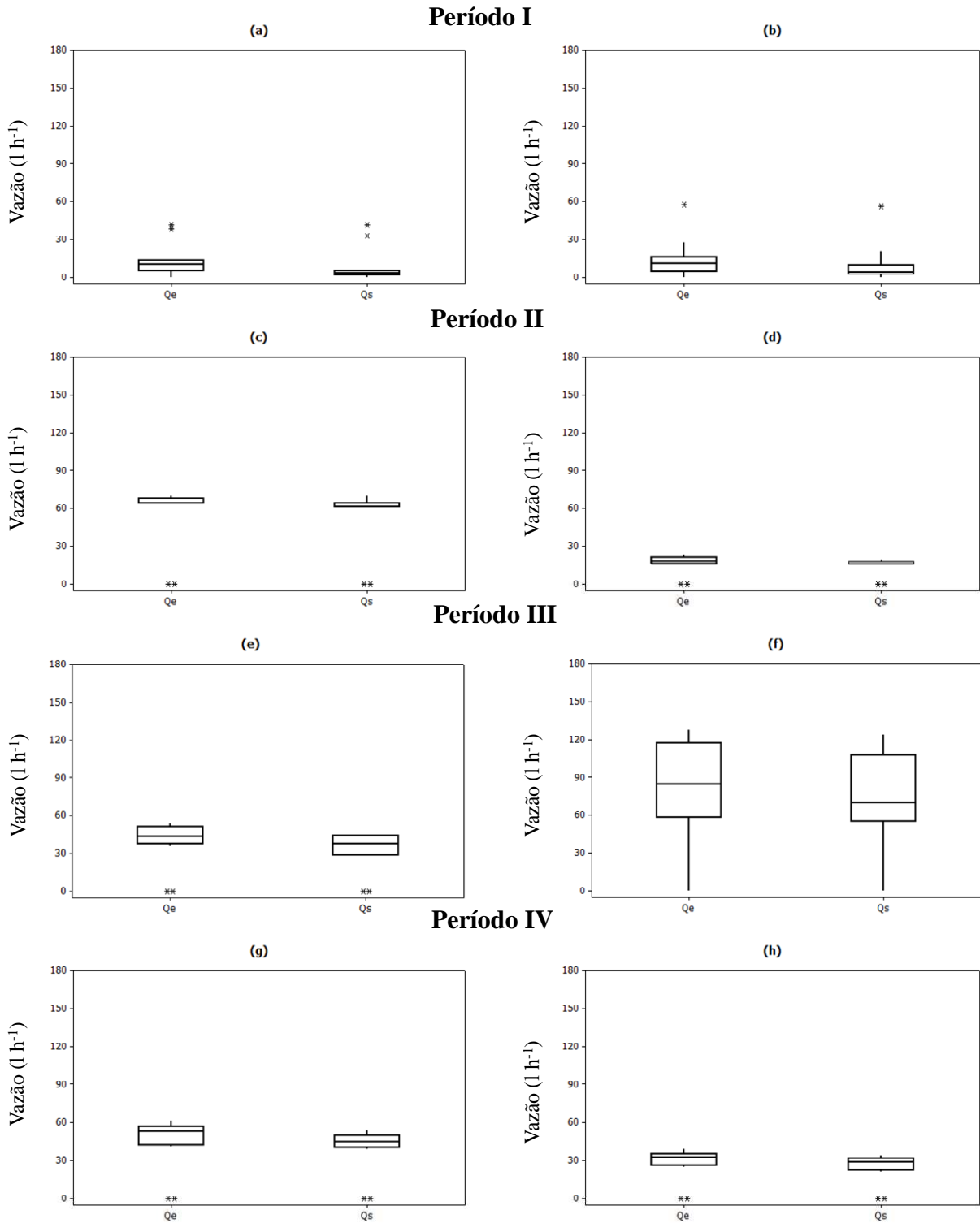
Figura 16. Gráficos “Box Plot” de Q_{ch} e Q_{sh} de dias característicos nos quatro períodos monitorados no leito Typha 1. Período I: 02/02/2006 (a) e 03/02/2006 (b); Período II: 19/09/2006 (c) e 20/09/2006 (d); Período III: 02/10/2007 (e) e 03/10/2007 (f) e; Período IV: 27/11/2007 (g) e 28/11/2007 (h). FEAGRI/UNICAMP, 2006 - 2007.
