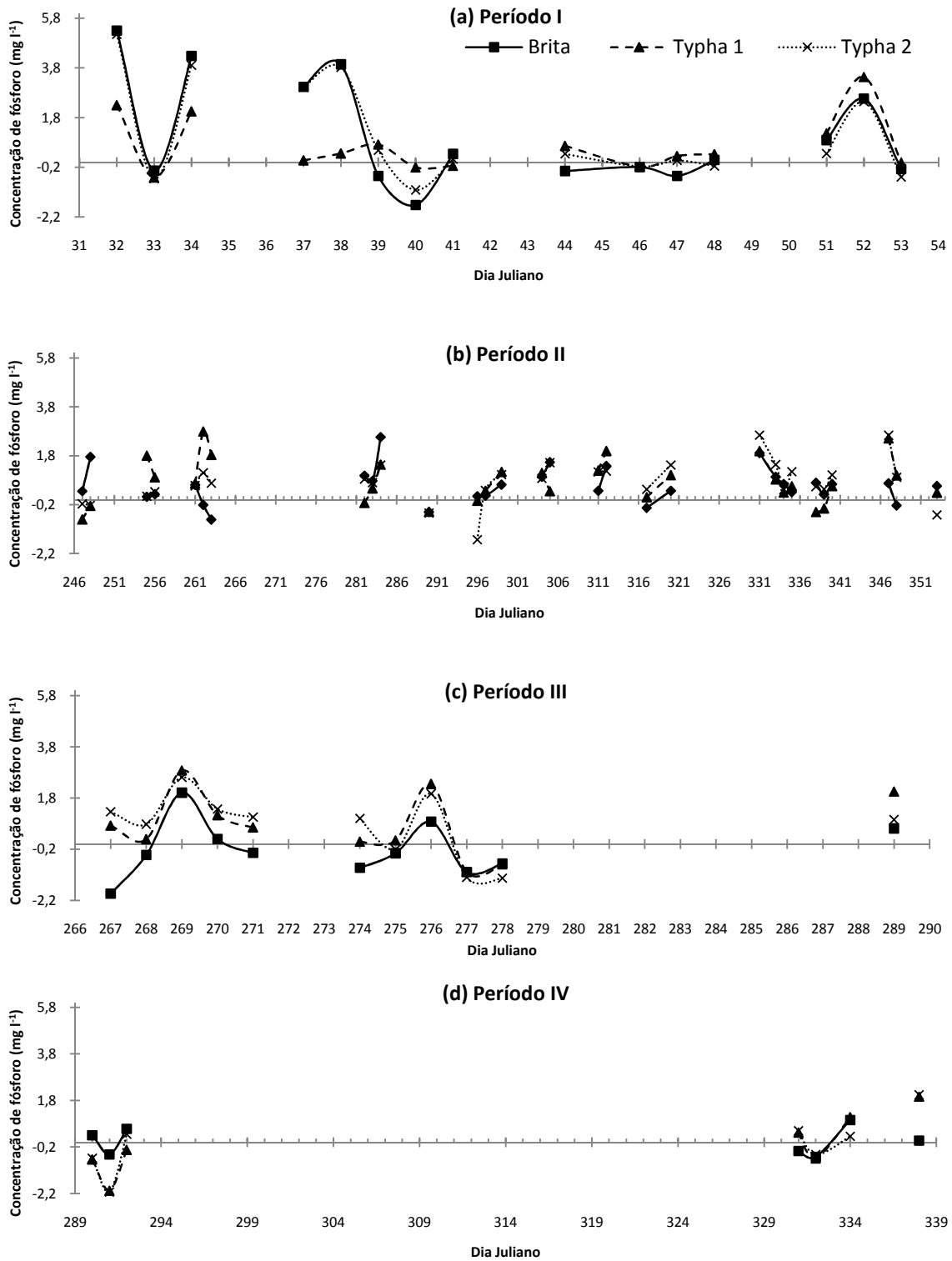
Figura 42. Valor médio do \Delta\text{PPT}_d nos quatro períodos monitorados. Período I (a), Período II (b), Período III (c) e Período IV (d). FEAGRI/UNICAMP, 2006 - 2007. Período I (01 a 22/02/2006), Período II (04/09 a 20/12/2006), Período III (24/09 a 16/10/2007) e Período IV (17/10 a 04/12/2007).
