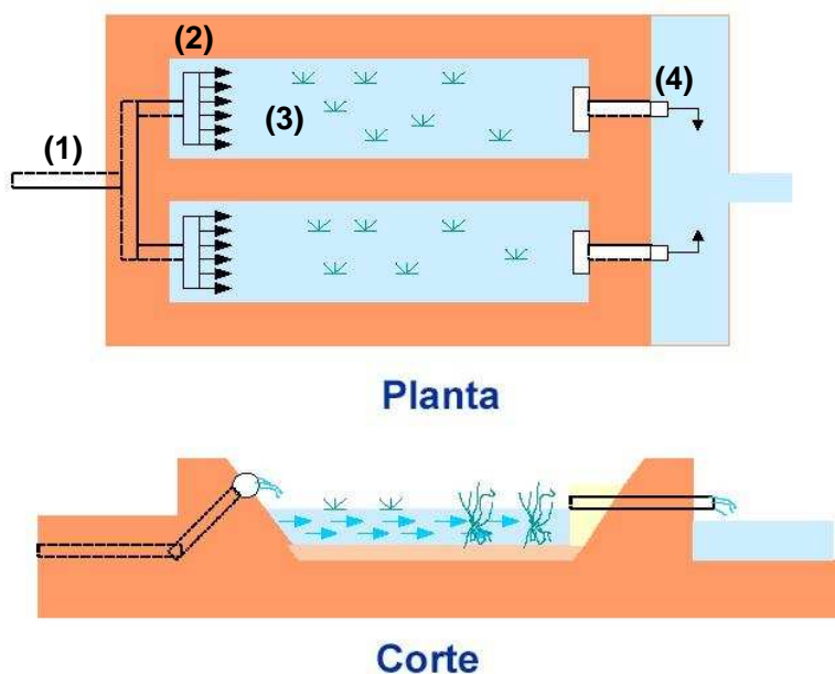
Figura 1. Configuração típica de um leito cultivado de fluxo superficial. Modificado de Kadlec & Knight (1996).
