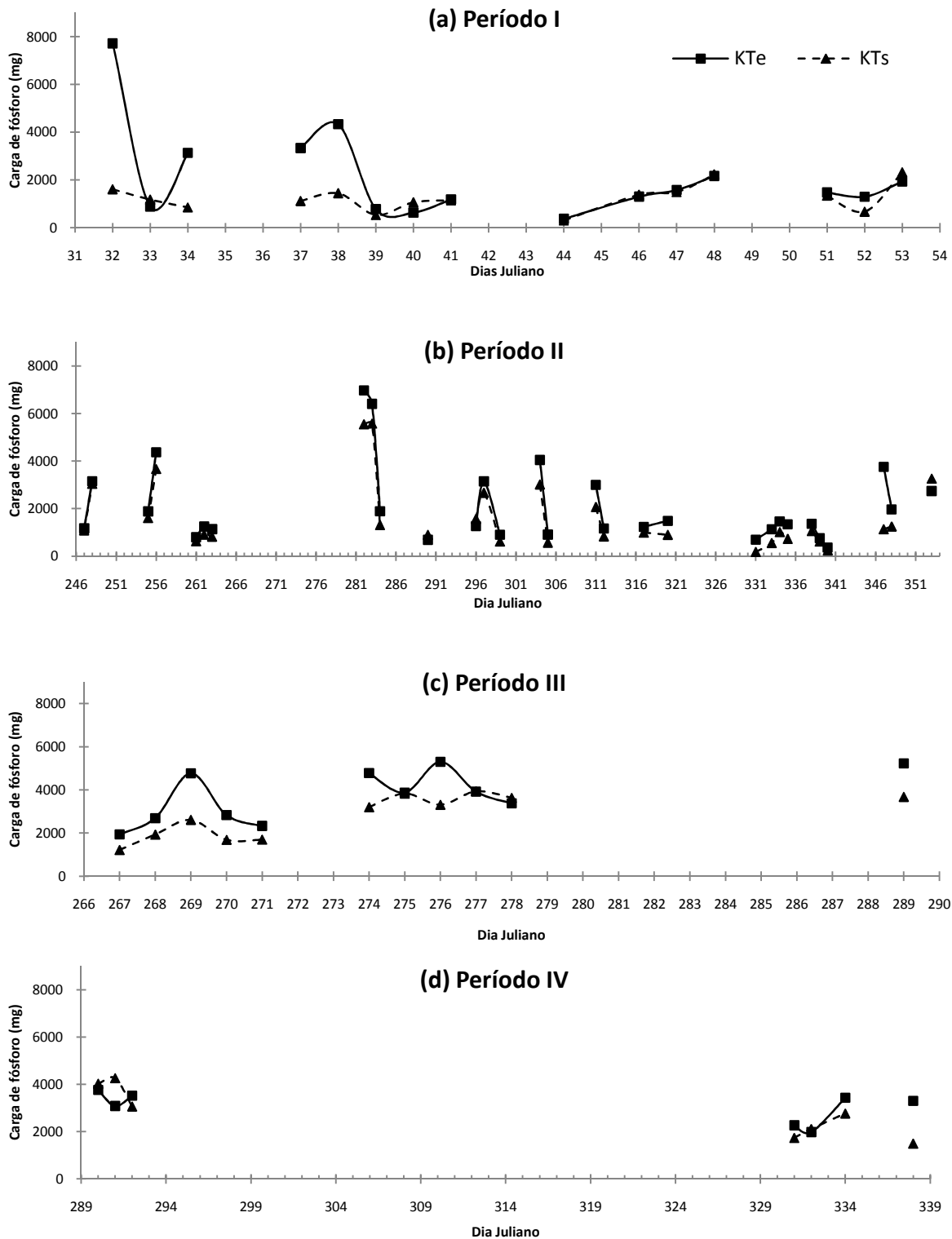
Figura 45. Valor médio de KT_{ed} e KT_{sd} nos quatro períodos monitorados no leito Typha 2. Período I (a), Período II (b), Período III (c) e Período IV (d). FEAGRI/UNICAMP, 2006 - 2007. Período I (01 a 22/02/2006), Período II (04/09 a 20/12/2006), Período III (24/09 a 16/10/2007) e Período IV (17/10 a 04/12/2007).
