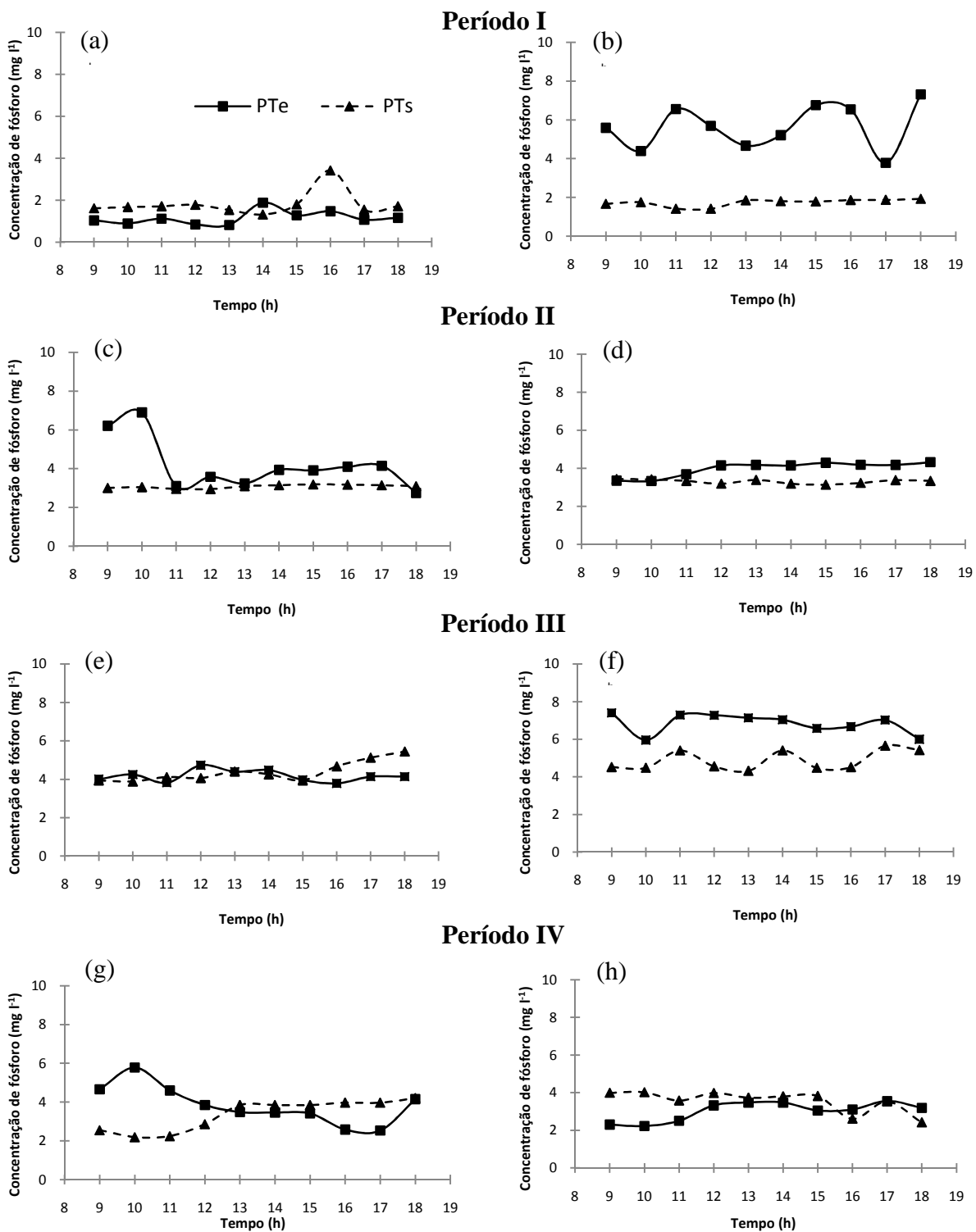
Figura 23. Valor horário de concentração de PT_{eh} e PT_{sh} de dias característicos nos quatro períodos monitorados no leito Typha 2. Período I: 02/02/2006 (a) e 03/02/2006 (b); Período II: 19/09/2006 (c) e 20/09/2006 (d); Período III: 02/10/2007 (e) e 03/10/2007 (f) e; Período IV: 27/11/2007 (g) e 28/11/2007 (h). FEAGRI/UNICAMP, 2006 - 2007.
