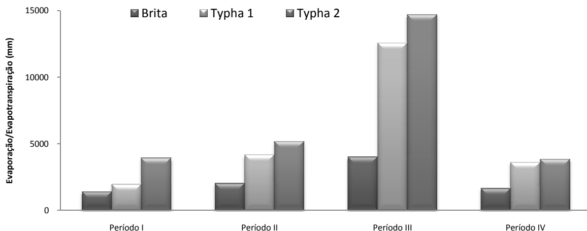
Figura 58. Volume total evaporado/evapotranspirado no período estendido. Período I (01/02 a 02/06/2006), Período II (04/09 a 20/12/2006), Período III (03/07 a 16/10/2007) e Período IV (17/10 a 04/12/2007). FEAGRI/UNICAMP, 2006 - 2007.
