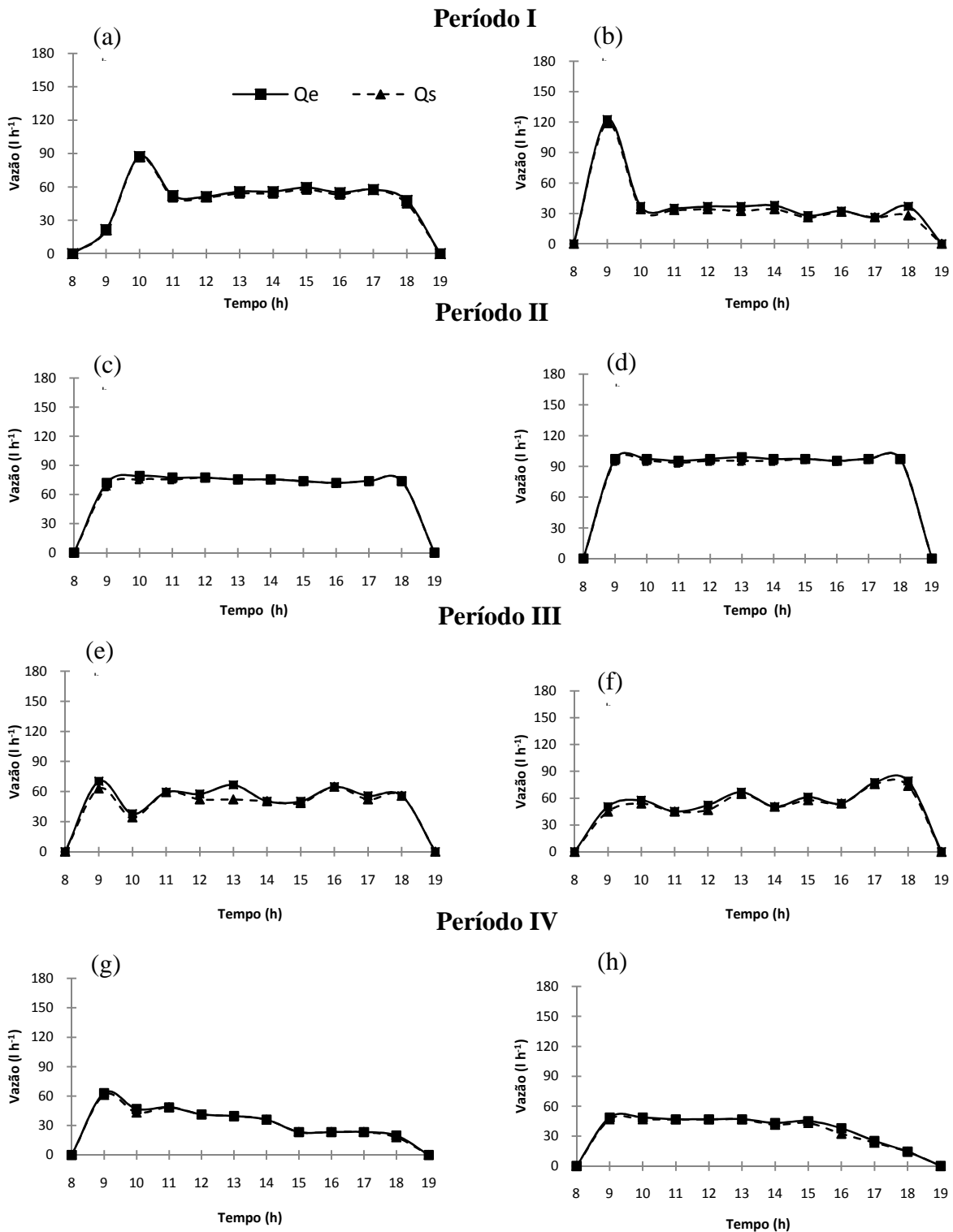
Figura 13. Valor horário medido de Q_{eh} e Q_{sh} de dias característicos nos quatro períodos monitorados no leito Brita. Período I: 02/02/2006 (a) e 03/02/2006 (b); Período II: 19/09/2006 (c) e 20/09/2006 (d); Período III: 02/10/2007 (e) e 03/10/2007 (f) e; Período IV: 27/11/2007 (g) e 28/11/2007 (h). FEAGRI/UNICAMP, 2006 - 2007.
