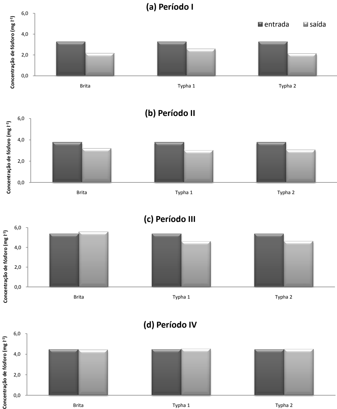
Figura 53. Valor médio diário de PT_{epm} e PT_{spm} dos leitos cultivados (leito Brita, leito Typha 1 e leito Typha 2). Período I (a), Período II (b), Período III (c) e Período IV (d). FEAGRI/UNICAMP, 2006 - 2007. Período I (01 a 22/02/2006), Período II (04/09 a 20/12/2006), Período III (24/09 a 16/10/2007) e Período IV (17/10 a 04/12/2007).
