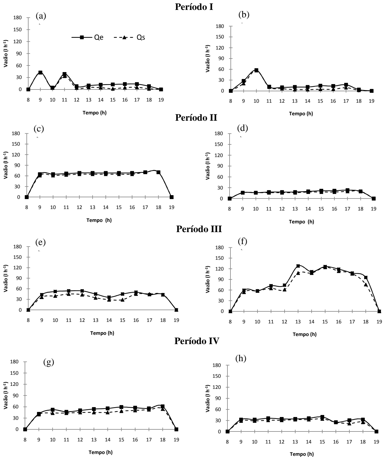
Figura 15. Valor horário medido de Q_{eh} e Q_{sh} de dias característicos nos quatro períodos monitorados no leito Typha 1. Período I: 02/02/2006 (a) e 03/02/2006 (b); Período II: 19/09/2006 (c) e 20/09/2006 (d); Período III: 02/10/2007 (e) e 03/10/2007 (f) e; Período IV: 27/11/2007 (g) e 28/11/2007 (h). FEAGRI/UNICAMP, 2006 - 2007.
