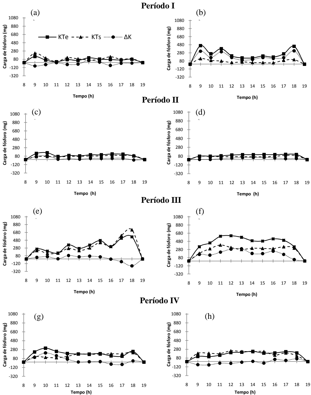
Figura 29. Valor horário de carga de KT_{ch} , KT_{sh} e \Delta KT_{sh} de dias característicos nos quatro períodos monitorados no leito Typha 2. Período I: 02/02/2006 (a.) e 03/02/2006 (b.); Período II: 19/09/2006 (c.) e 20/09/2006 (d.); Período III: 02/10/2007 (e.) e 03/10/2007 (f.) e; Período IV: 27/11/2007 (g) e 28/11/2007 (h). FEAGRI/UNICAMP, 2006 - 2007.
