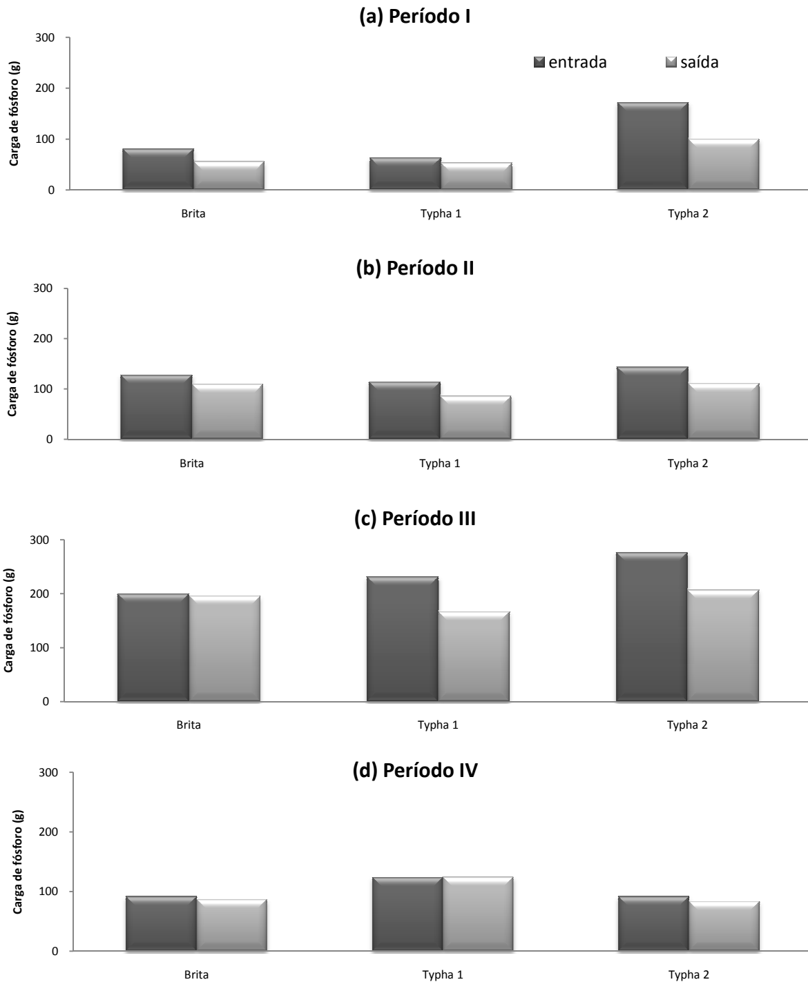
Figura 59. Valor total do período estendido de KT_{epe} e KT_{spe} dos leitos cultivados (leito Brita, leito Typha 1 e leito Typha 2). Período I (a), Período II (b), Período III (c) e Período IV (d). FEAGRI/UNICAMP, 2006 - 2007. Período I (01/02 a 02/06/2006), Período II (04/09 a 20/12/2006), Período III (03/07 a 16/10/2007) e Período IV (17/10 a 04/12/2007).
