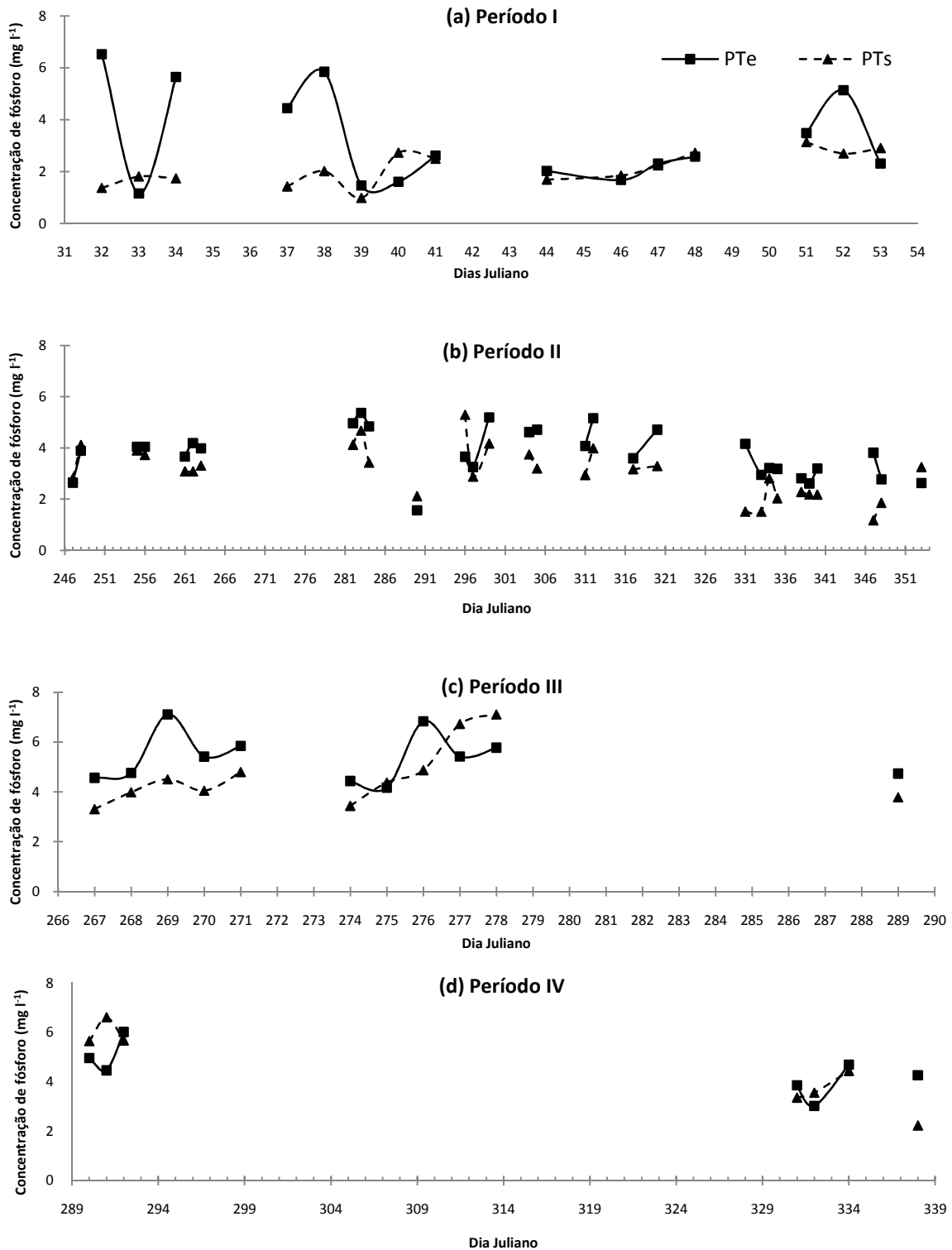
Figura 41. Valor médio de PT_{ed} e PT_{sd} nos quatro períodos monitorados no leito Typha 2. Período I (a), Período II (b), Período III (c) e Período IV (d). FEAGRI/UNICAMP, 2006 - 2007. Período I (01 a 22/02/2006), Período II (04/09 a 20/12/2006), Período III (24/09 a 16/10/2007) e Período IV (17/10 a 04/12/2007).
