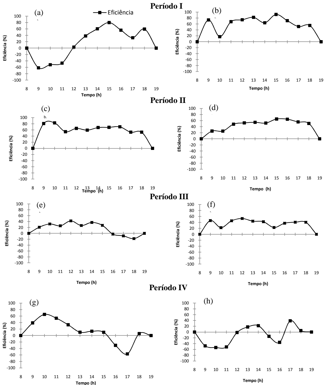
Figura 32. Valor horário da eficiência de retenção de fósforo de dias característicos nos quatro períodos monitorados no leito Typha 1. Período I: 02/02/2006 (a) e 03/02/2006 (b); Período II: 19/09/2006 (c) e 20/09/2006 (d); Período III: 02/10/2007 (e) e 03/10/2007 (f) e; Período IV: 27/11/2007 (g) e 28/11/2007 (h). FEAGRI/UNICAMP, 2006 - 2007.
