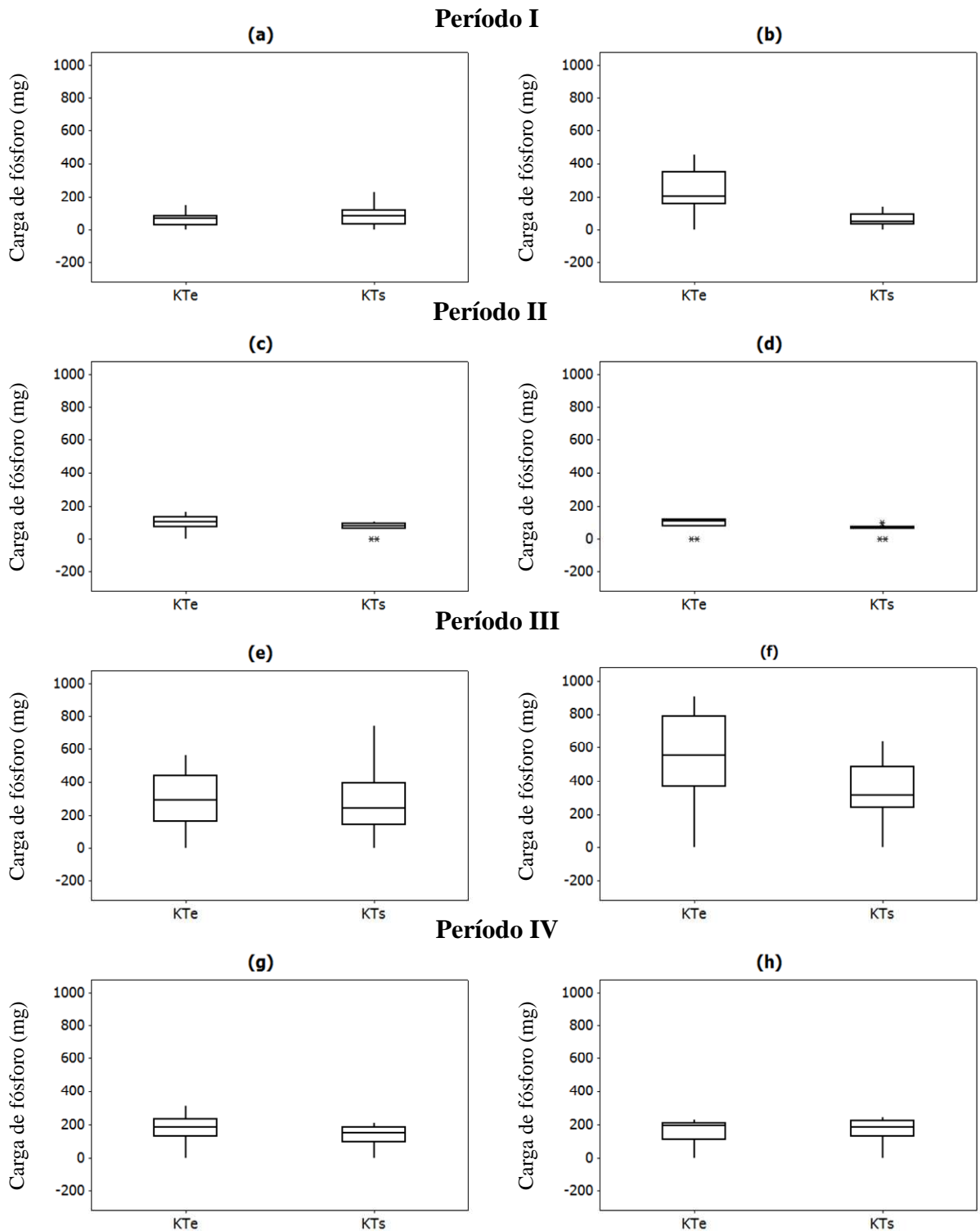
Figura 30. Gráficos “Box Plot” de KT_{ch} e KT_{sh} de dias característicos nos quatro períodos monitorados no leito Typha 2. Período I: 02/02/2006 (a) e 03/02/2006 (b); Período II: 19/09/2006 (c) e 20/09/2006 (d); Período III: 02/10/2007 (e); 03/10/2007 (f) e; Período IV: 27/11/2007 (g) e 28/11/2007 (h). FEAGRI/UNICAMP, 2006 - 2007.
