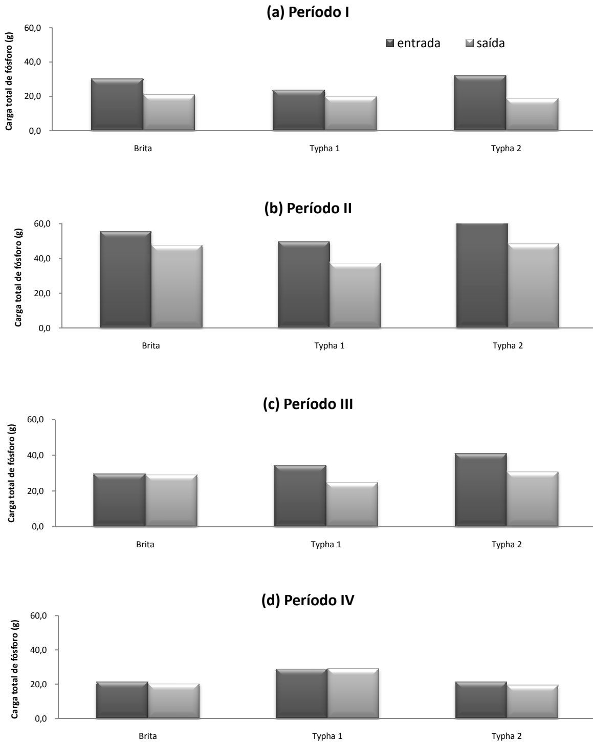
Figura 55. Valor total de KT_{epm} e KT_{spm} dos leitos cultivados (leito Brita, leito Typha 1 e leito Typha 2). Período I (a), Período II (b), Período III (c) e Período IV (d). FEAGRI/UNICAMP, 2006 - 2007. Período I (01 a 22/02/2006), Período II (04/09 a 20/12/2006), Período III (24/09 a 16/10/2007) e Período IV (17/10 a 04/12/2007).
