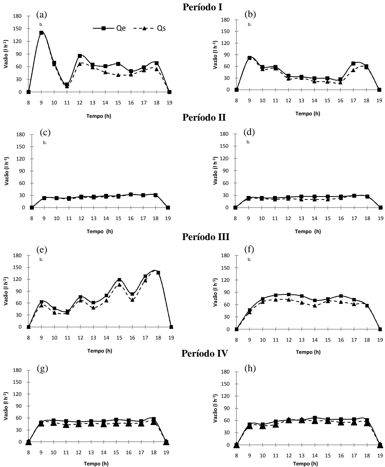
Figura 17. Valor horário medido de Q_{eh} e Q_{sh} de dias característicos nos quatro períodos monitorados no leito Typha 2. Período I: 02/02/2006 (a) e 03/02/2006 (b); Período II: 19/09/2006 (c) e 20/09/2006 (d); Período III: 02/10/2007 (e) e 03/10/2007 (f) e; Período IV: 27/11/2007 (g) e 28/11/2007 (h). FEAGRI/UNICAMP, 2006 - 2007.
