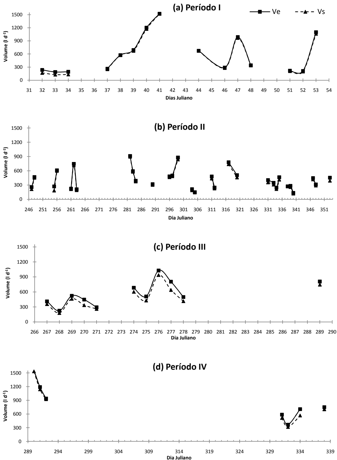
Figura 35. Valor médio diário de V_{ed} e V_{sd} nos quatro períodos monitorados no leito Typha 1. Período I (a), Período II (b), Período III (c) e Período IV (d). FEAGRI/UNICAMP, 2006 - 2007. Período I (01 a 22/02/2006), Período II (04/09 a 20/12/2006), Período III (24/09 a 16/10/2007) e Período IV (17/10 a 04/12/2007).
