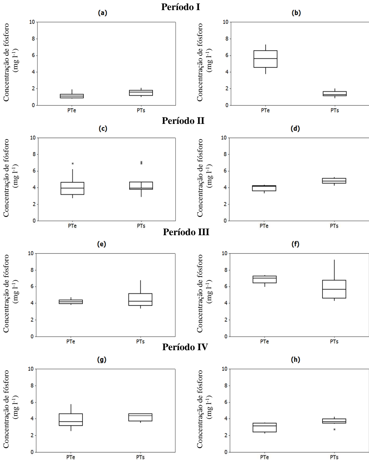
Figura 20. Gráficos “Box Plot” de PT_{ch} e PT_{sh} de dias característicos nos quatro períodos monitorados no leito Brita. Período I: 02/02/2006 (a) e 03/02/2006 (b); Período II: 19/09/2006 (c) e 20/09/2006 (d); Período III: 02/10/2007 (e) e 03/10/2007 (f) e; Período IV: 27/11/2007 (g) e 28/11/2007 (h). FEAGRI/UNICAMP, 2006 - 2007.
