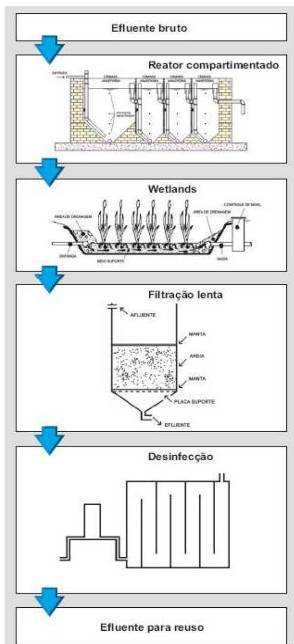
Figura 9. Fluxograma do tratamento dos efluentes gerado na Faculdade de Engenharia Agrícola da UNICAMP e financiado pelo PROSAB.
