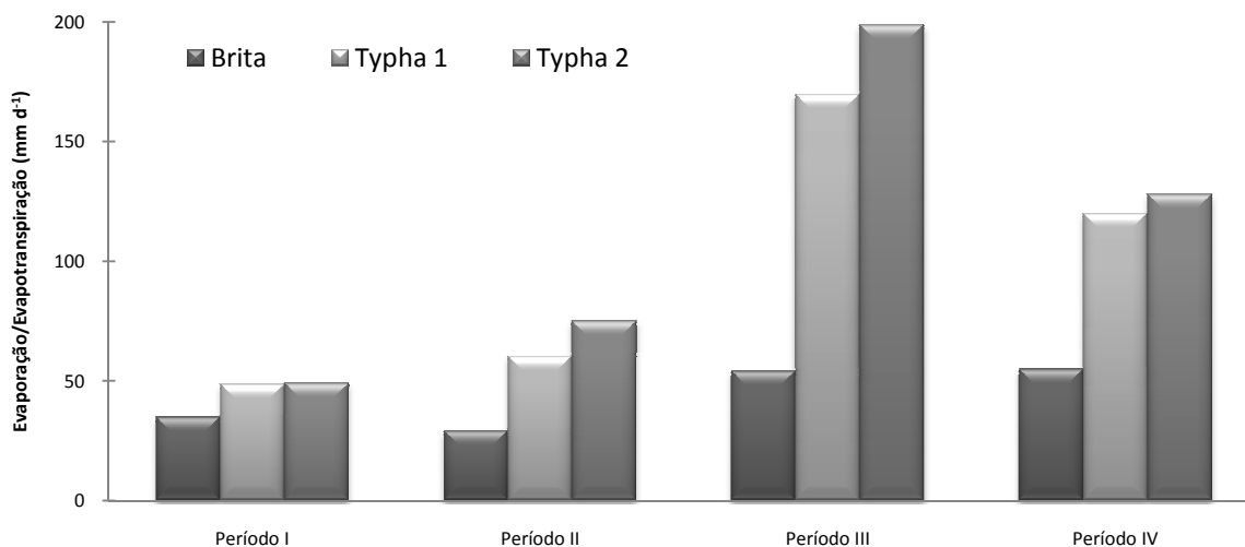
Figura 50. Volume médio diário da evaporação/evapotranspiração nos quatro períodos monitorados. Período I (01 a 22/02/2006), Período II (04/09 a 20/12/2006), Período III (24/09 a 16/10/2007) e Período IV (17/10 a 04/12/2007). FEAGRI/UNICAMP, 2006 - 2007.
