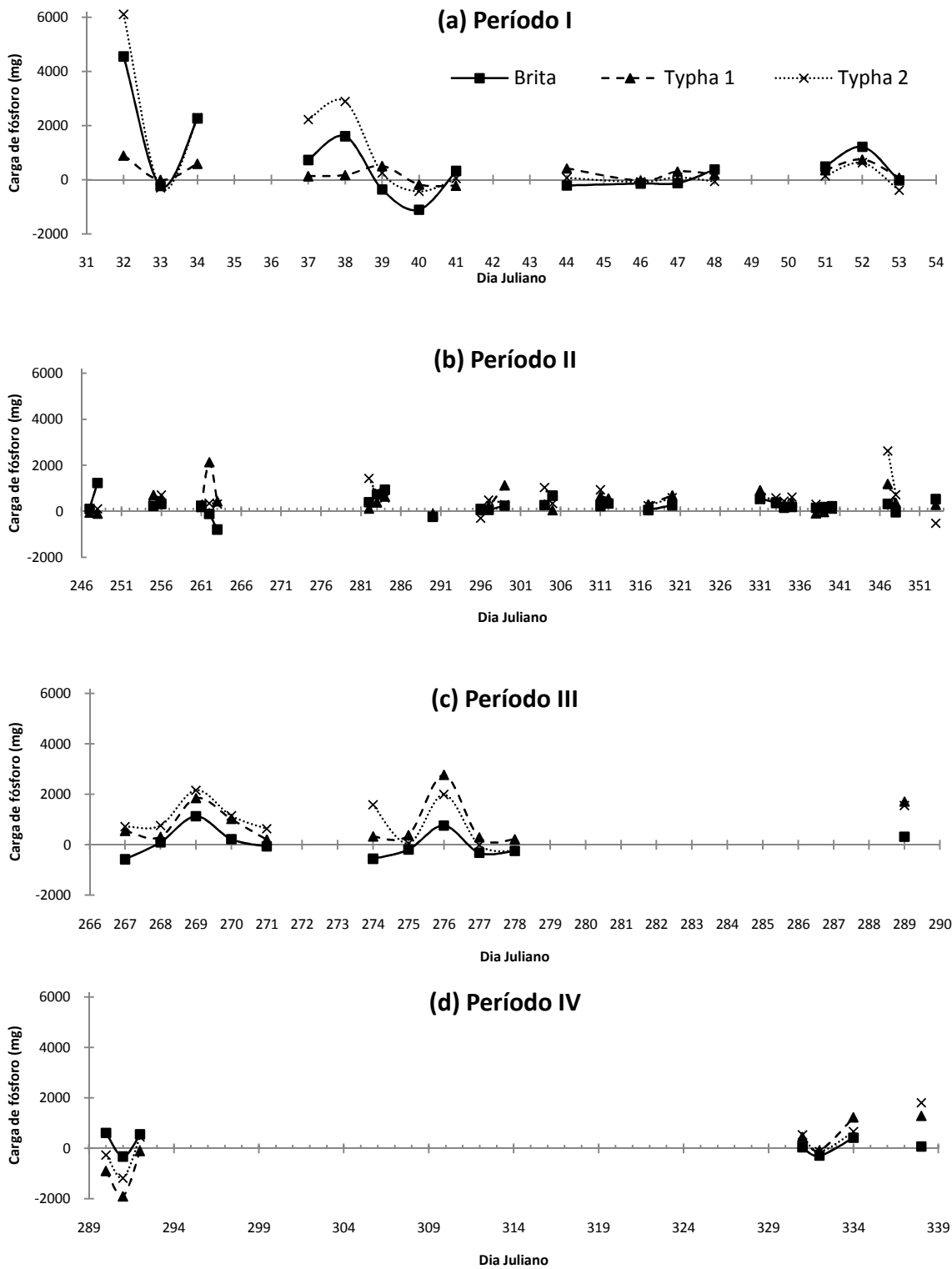
Figura 46. Valor médio de \Delta KT_d nos quatro períodos monitorados. Período I (a), Período II (b), Período III (c) e Período IV (d). FEAGRI/UNICAMP, 2006 - 2007. Período I (01 a 22/02/2006), Período II (04/09 a 20/12/2006), Período III (24/09 a 16/10/2007) e Período IV (17/10 a 04/12/2007).
