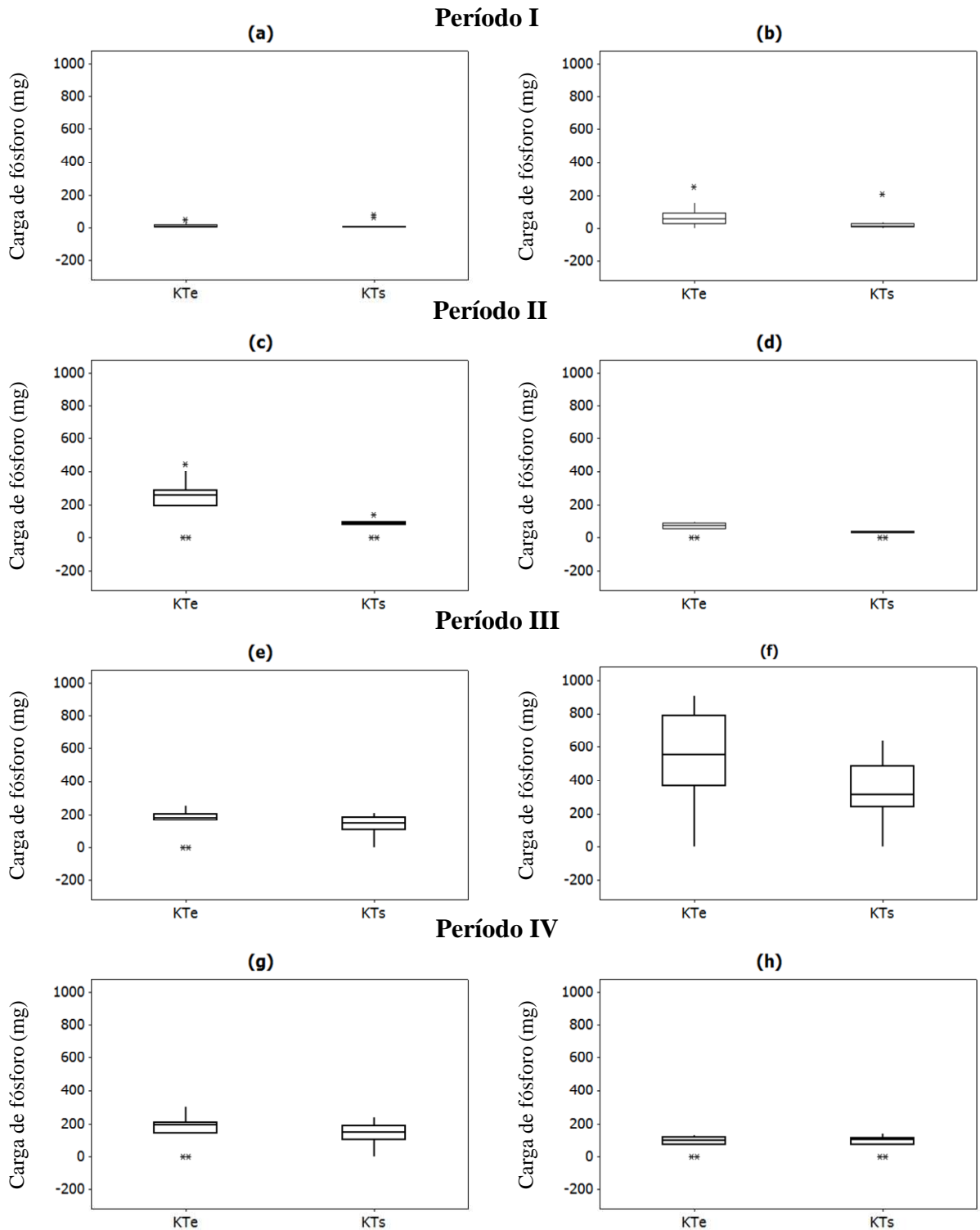
Figura 28. Gráficos “Box Plot” de KT_{eh} e KT_{sh} de dias característicos nos quatro períodos monitorados no leito Typha1. Período I: 02/02/2006 (a) e 03/02/2006 (b); Período II: 19/09/2006 (c) e 20/09/2006 (d); Período III: 02/10/2007 (e); 03/10/2007 (f) e; Período IV: 27/11/2007 (g) e 28/11/2007 (h). FEAGRI/UNICAMP, 2006 - 2007.
