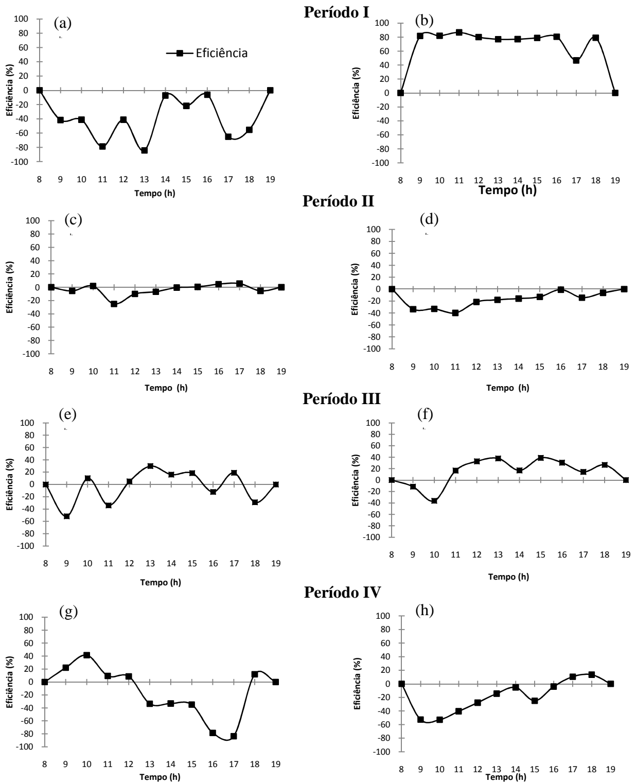
Figura 31. Valor horário da eficiência de retenção de fósforo de dias característicos nos quatro períodos monitorados no leito Brita. Período I: 02/02/2006 (a) e 03/02/2006 (b); Período II: 19/09/2006 (c) e 20/09/2006 (d); Período III: 02/10/2007 (e) e 03/10/2007 (f) e; Período IV: 27/11/2007 (g) e 28/11/2007 (h). FEAGRI/UNICAMP, 2006 - 2007.
