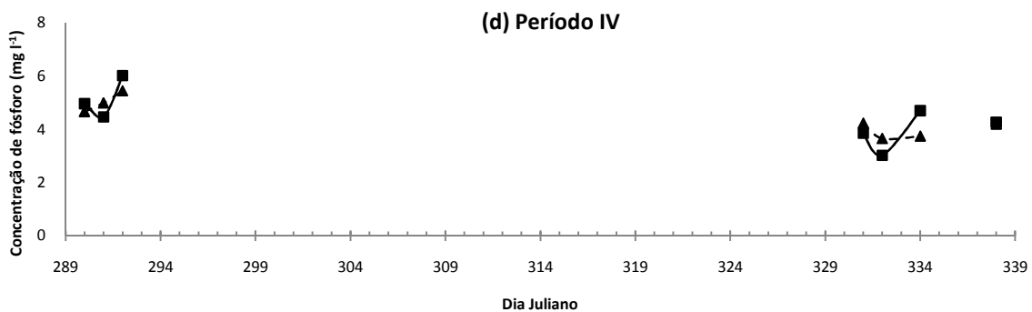
Figura 39. Valor médio de PT_{ed} e PT_{sd} nos quatro períodos monitorados no leito Brita. Período I (a), Período II (b), Período III (c) e Período IV (d). FEAGRI/UNICAMP, 2006 - 2007. Período I (01 a 22/02/2006), Período II (04/09 a 20/12/2006), Período III (24/09 a 16/10/2007) e Período IV (17/10 a 04/12/2007).
