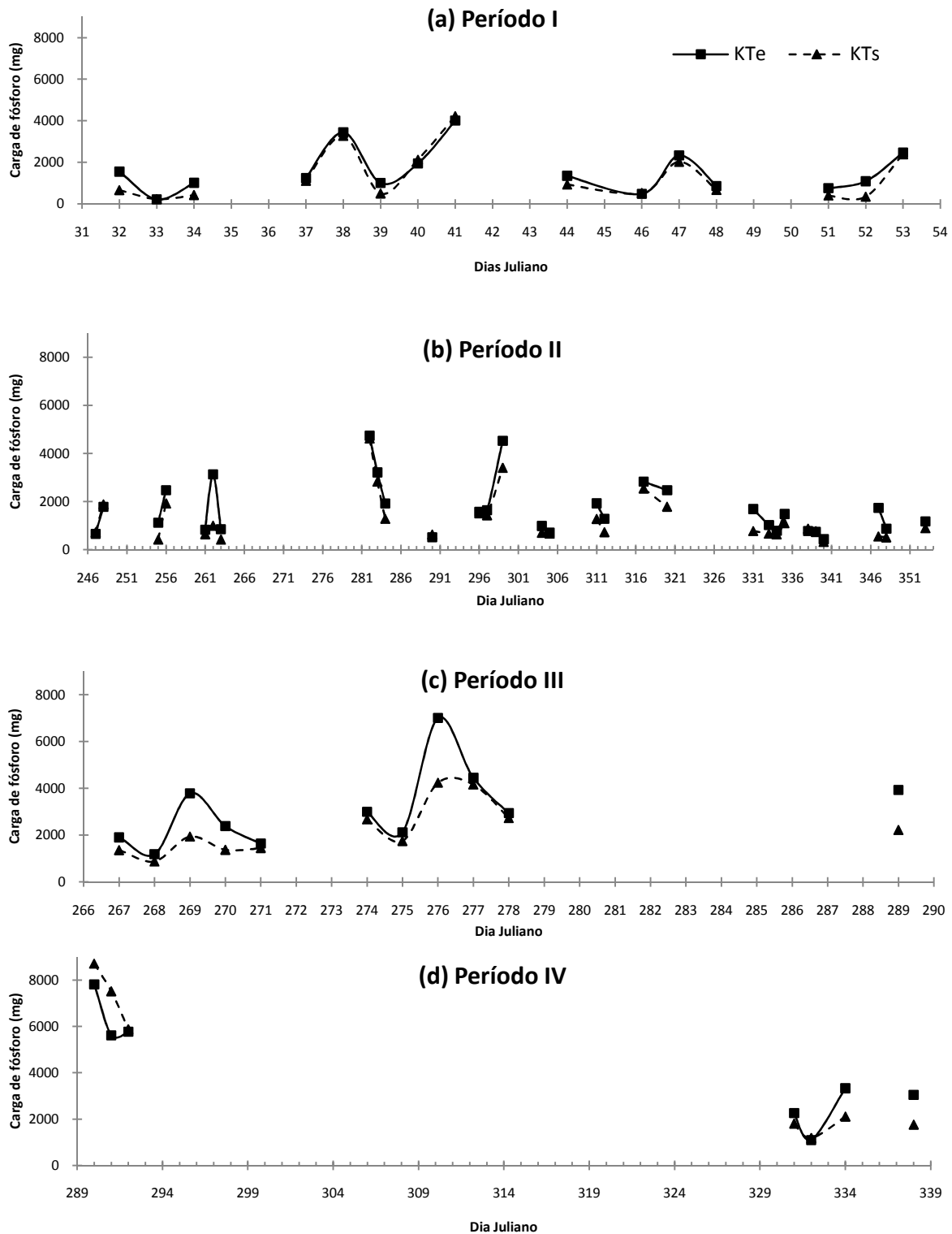
Figura 44. Valor médio de KT_{ed} e KT_{sd} nos quatro períodos monitorados no leito Typha 1. Período I (a), Período II (b), Período III (c) e Período IV (d). FEAGRI/UNICAMP, 2006 - 2007. Período I (01 a 22/02/2006), Período II (04/09 a 20/12/2006), Período III (24/09 a 16/10/2007) e Período IV (17/10 a 04/12/2007).
