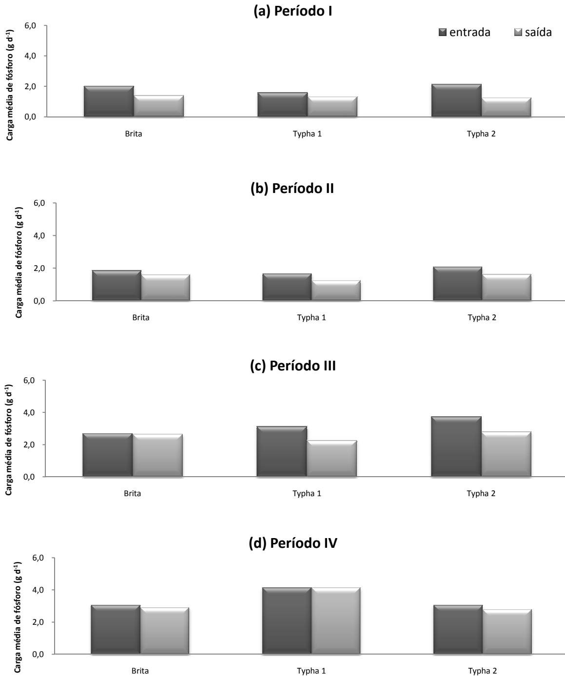
Figura 54. Valor médio diário de KT_{epm} e KT_{spm} dos leitos cultivados (leito Brita, leito Typha 1 e leito Typha 2). Período I (a), Período II (b), Período III (c) e Período IV (d). FEAGRI/UNICAMP, 2006 - 2007. Período I (01 a 22/02/2006), Período II (04/09 a 20/12/2006), Período III (24/09 a 16/10/2007) e Período IV (17/10 a 04/12/2007).
