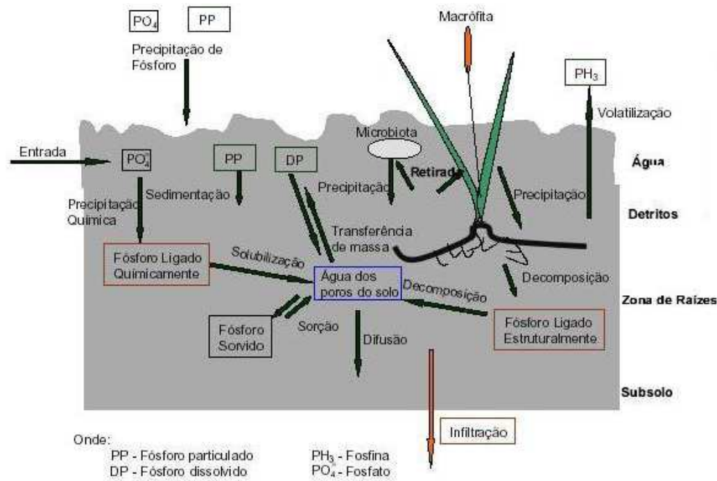
Figura 4. Esquema simplificado dos processos que envolvem o fósforo nos leitos cultivados (Kadlec & Knight, 1996).
