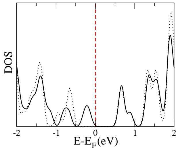
Figura 3.15: Densidade de Estados (DOS) para o nanotubo de \text{BC}_2\text{N} armchair (3,3) com o antissítio B_{CI} . A linha pontilhada representa a DOS do sistema sem defeito enquanto a linha contínua representa a DOS do sistema com defeito. O nível de Fermi para o sistema com defeito está indicado por uma linha vertical tracejada em energia igual a zero.
