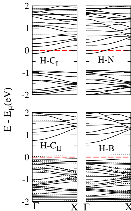
Figura 4.2: Estrutura de bandas para o nanotubo de BC_2N zigzag (4,0) quando um átomo de H é adsorvido sobre os átomos C_I , C_{II} , N e B.
