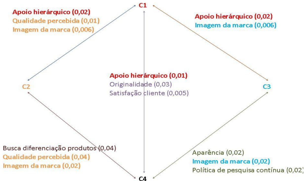
Figura 44 - Clusters e variáveis dos blocos 2, 3, 4 e 5 que apresentam diferenças significativas nas suas médias
