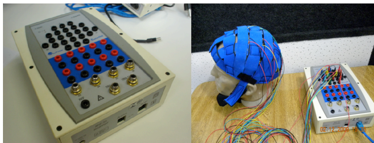
Figura 4.1 – Amplificador de sinais biológicos, BrainNet BNT – 36 da Lynux Tecnologia Eletrônica Ltda.
