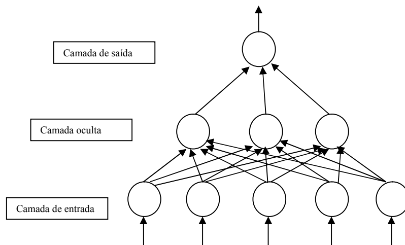
Figura 3.2 – Rede neural MLP com uma camada oculta.
