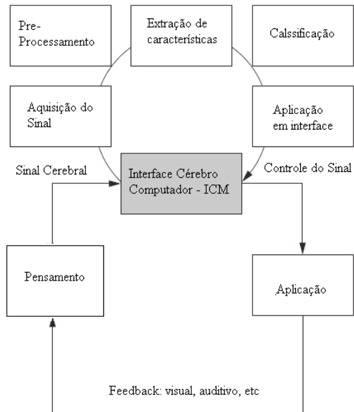
Figura 2.12 – Diagrama esquemático dos processos envolvidos em Interface Cérebro Máquina.
