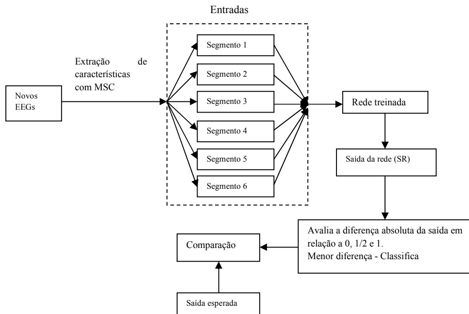
Figura 4.10 – Sistema de validação e classificação para os sinais EEG a partir dos redes treinadas de cada sujeito.
