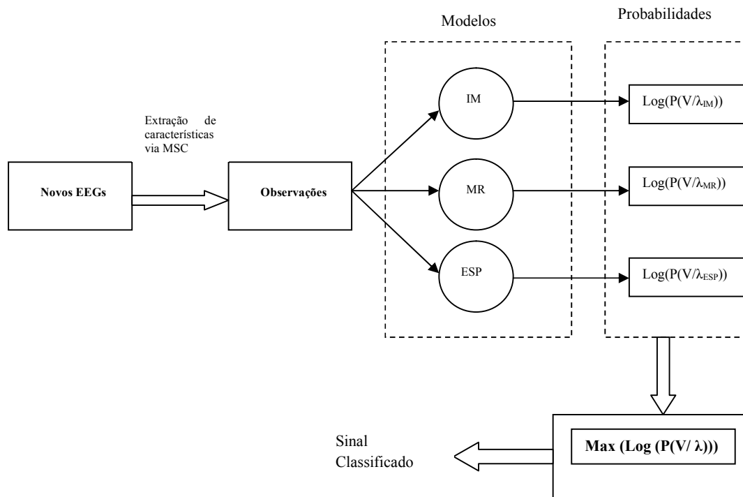
Figura 4.8 – Sistema de classificação para os sinais EEG a partir dos modelos HMM construídos para cada sujeito.
