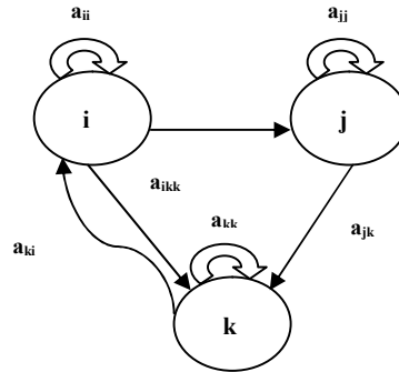
Figura 3.1 – Modelo Oculto de Markov com 3 estados (i, j, k). Modificado de YNOGUTI, 1999.
