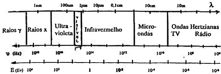
Figura 3. Espectro Eletromagnético.
