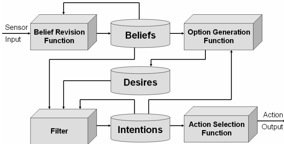
Figura 12 – Diagrama de uma arquitetura BDI genérica Fonte: Wooldridge (2002).
