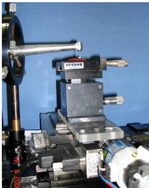
Figura 3 – Posicionamento da amostra e da fibra do laser de Er,Cr:YSGG em suportes ópticos e deslocador micrométrico X-Y para padronizar as irradiações.
