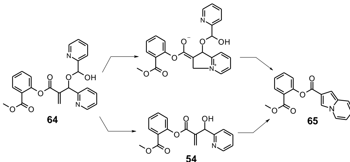
Esquema 4.15 Formação da indolizina ( 65 ) a partir do hemiacetal ( 64 ) ou do aduto de MBH ( 54 ).
