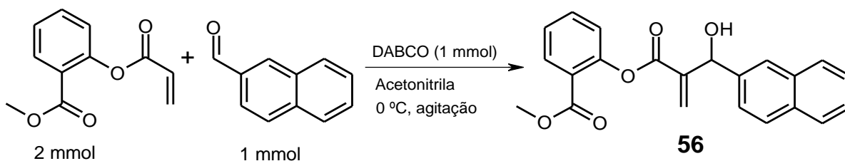
Esquema 4.13 Metodologia para a reação de MBH na obtenção do aduto 56 .
