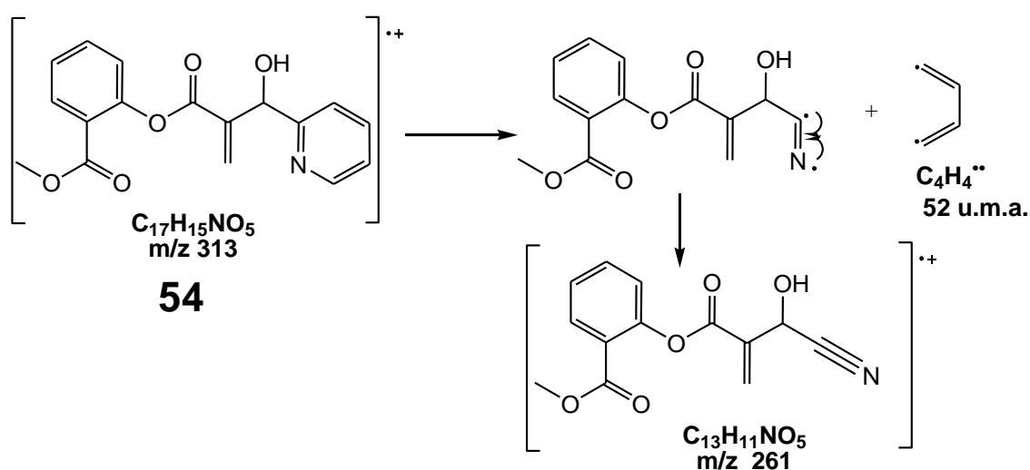
Esquema 4.17 Formação do fragmento de m/z 261.
