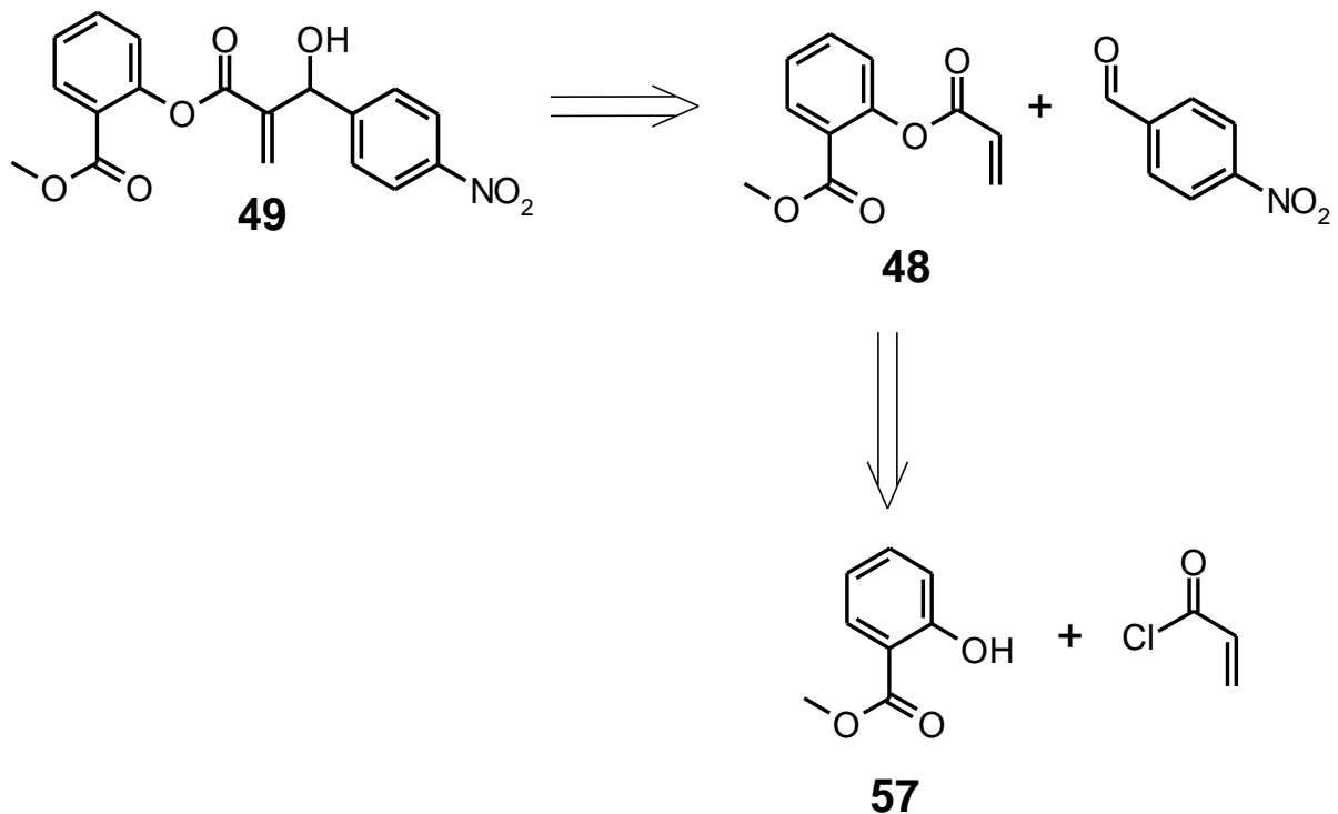
Figura 3.3 Análise retrossintética de um aduto de MBH proposto no trabalho.
