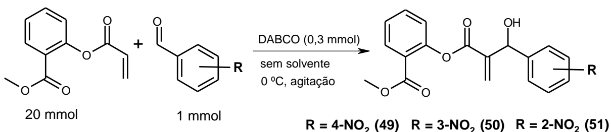
Esquema 4.9 Metodologia de otimização da reação de MBH para os adutos 49 , 50 e 51 .
