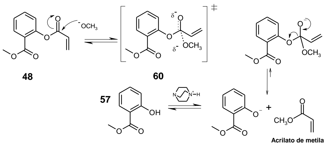
Esquema 4.7 Mecanismo de reação de solvólise básica do acrilato 48 pelo metanol.
