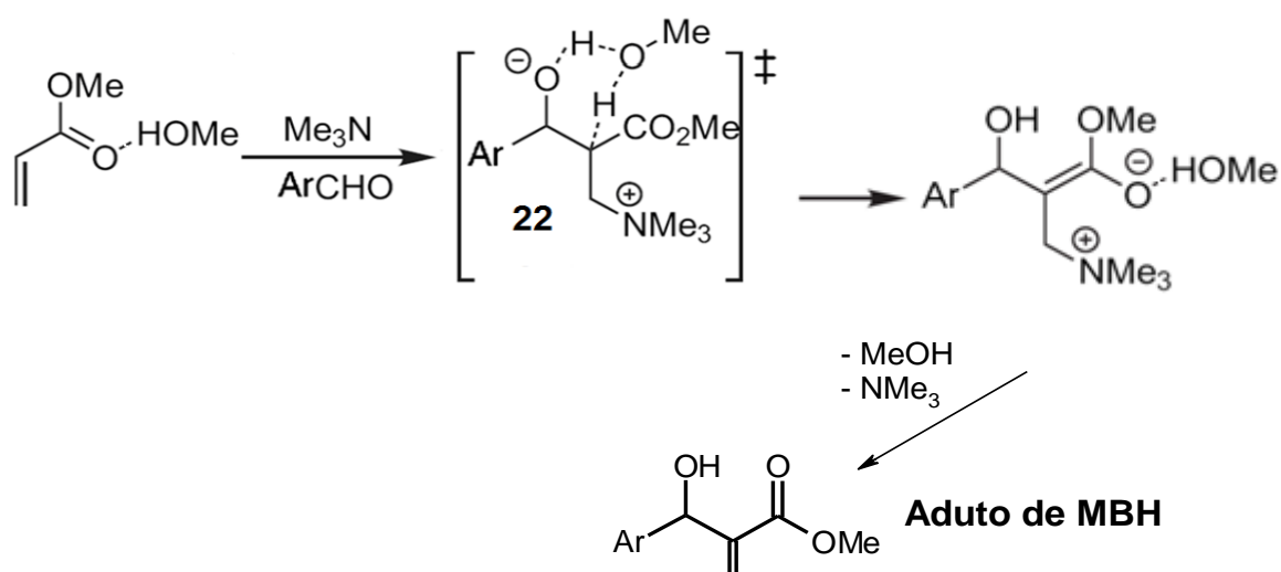
Esquema 1.8 Transferência de próton realizada pelo metanol para a formação do aduto de MBH.
