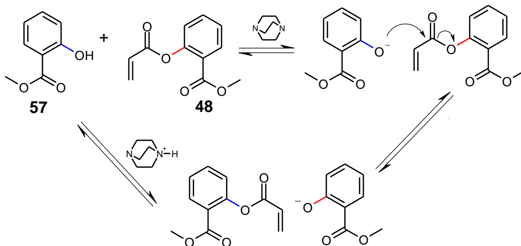
Esquema 4.8 Mecanismo simplificado da reação de transesterificação do acrilato 48 com o salicilato de metila.
