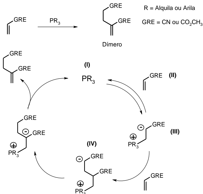
Esquema 1.3 Dimerização de Rauhut e Currier utilizando alcenos ativados.
