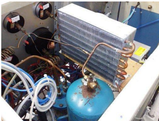
Figura 4.18 – Trocador de calor instalado na entrada do reservatório.
