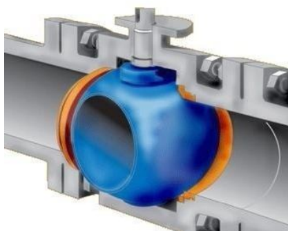
Figura 3.5 – Válvula esfera em corte, em posição fechada (39).
