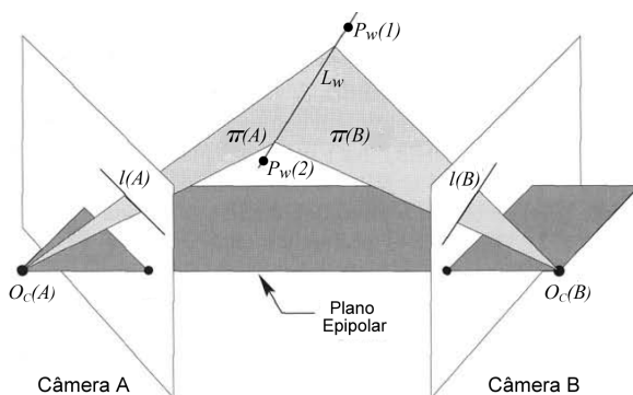
Figura 25: Representação esquemática do processo de reconstrução de linhas (HARTLEY; ZISSERMAN, 2003).
