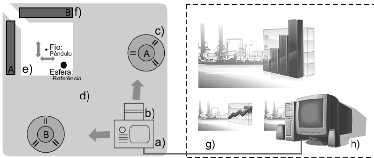
Figura 26: Leiaute do protótipo desenvolvido: a) câmera digital, b) lente objetiva, c) SFI, d) plataforma de montagem, e) abertura de passagem, fio de pêndulo e esfera de referência, f) back-light , g) cabo de comunicação e h) computador.
