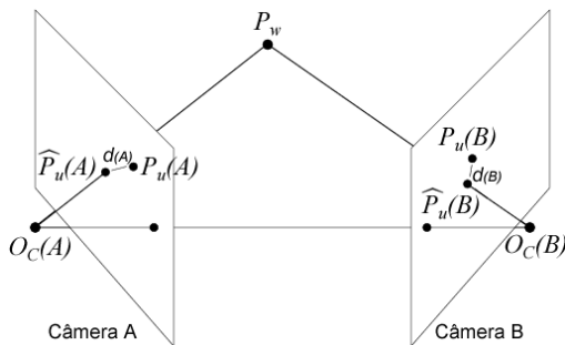
Figura 24: Representação esquemática do processo de triangulação real com restrição epolar imposta (HARTLEY; ZISSERMAN, 2003).
