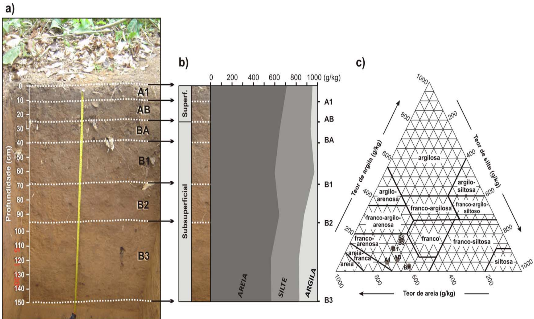
Figura 3: a) Perfil de solo adjacente 1 com delimitação dos horizontes; b) Distribuição das frações granulométricas; c) Classes texturais dos horizontes segundo o triângulo de classificação textural de solos (Lemos & Santos, 2002).
