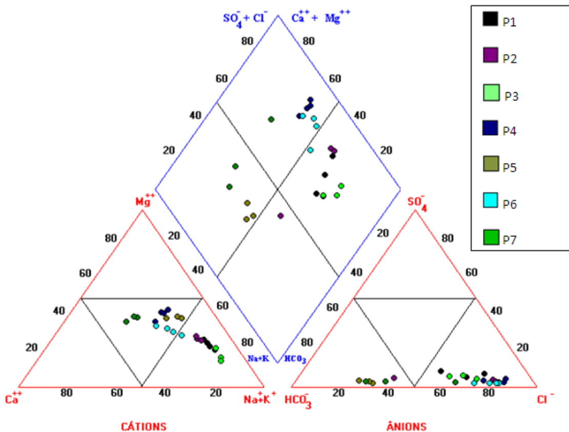
Figura 4.2 - O diagrama de Piper das águas de todos os poços
