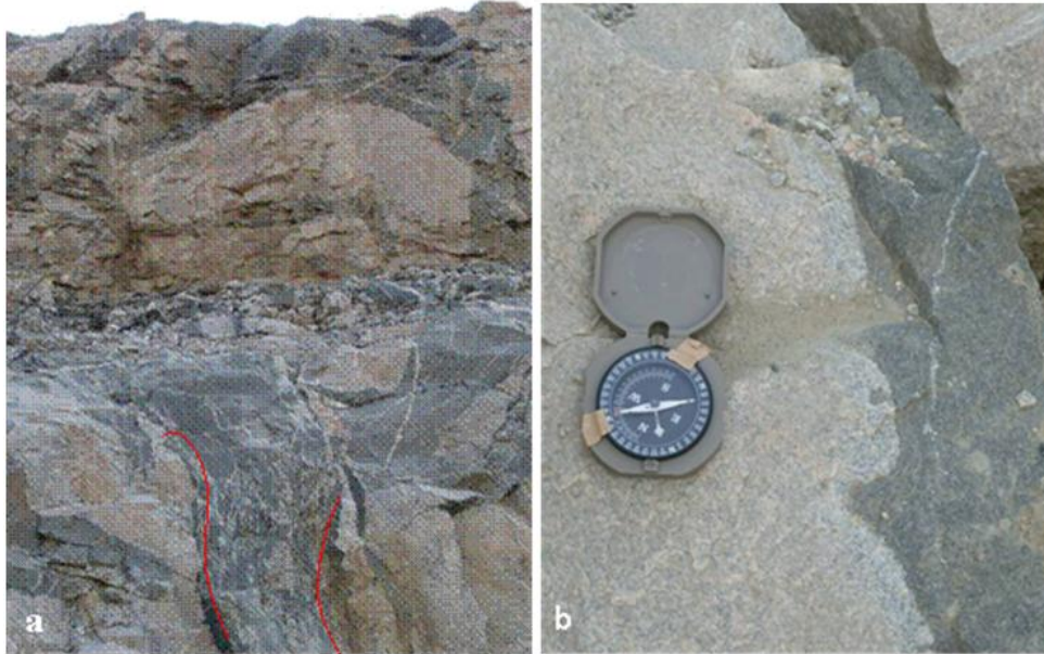
Figura 2.6 - (a) Contato entre o monzo-granito e o anfibolito, destacado em vermelho. (b) Contato típico da mistura de magma entre as litologias. (Fonte: Santos)
