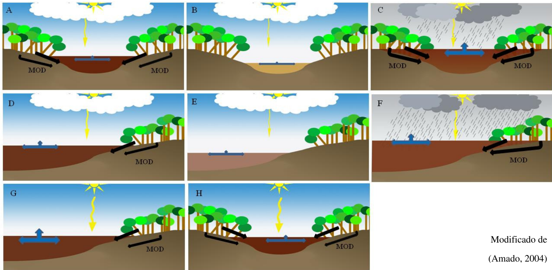
Figura 8 - Modelo esquemático do comportamento dos processos estudados de degradação da matéria orgânica dissolvida (MOD) no Lago Tupé (A-C,H) e Rio Negro (D-G) em um ciclo hidrológico. A e D, representam a vazante de 2008 e G e H, a vazante de 2009. Nesse período do ciclo, há maior coloração d' água, devido à redução do nível d' água e concentração da MOD advinda do igapó inundado na cheia. Mudanças na cobertura de nuvens influenciam os processos de fotodegradação, representado pela seta amarela, e degradação bacteriana, seta azul. Diferenças na espessura das setas representam a intensidade dos processos. B e E representam o período de seca, em que os dois processos atuam com menor intensidade e a cor d' água é mais clara. C e F representam as águas altas, onde há a maior entrada de MOD, do igapó e dos solos inundados. A cor d' água é semelhante entre os dois ambientes, assim como o processo de fotodegradação, enquanto a degradação bacteriana é maior no Lago.
