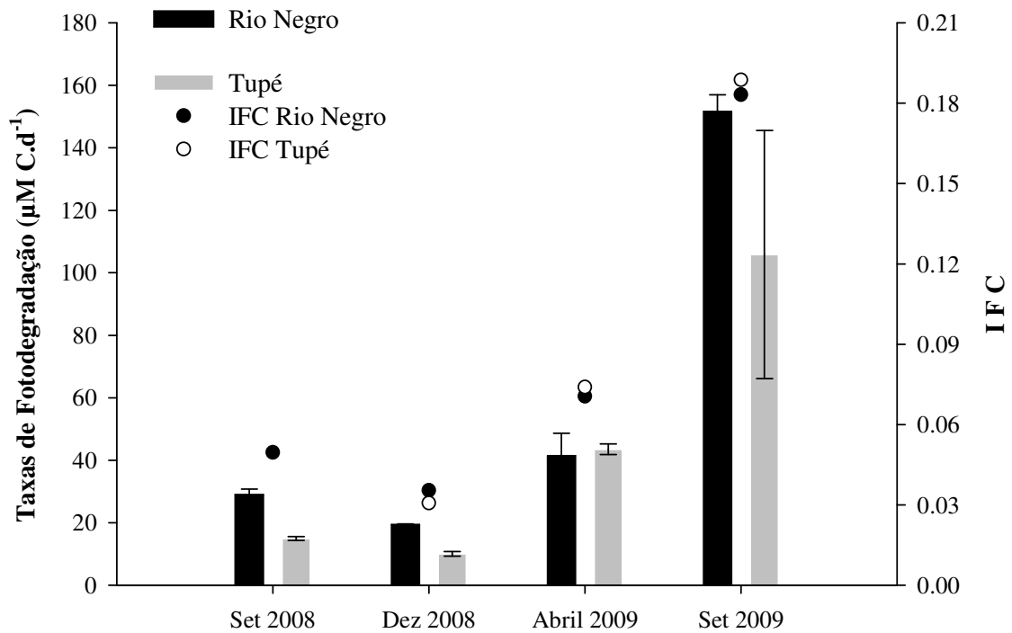
Figura 4 – Taxas de fotodegradação ( \mu\text{M C dia}^{-1} ) para o Rio Negro e lago Tupé. Índice de foto-reatividade (IFC) do COD para o Rio Negro e lago Tupé. Barras de erro representam desvio padrão.
