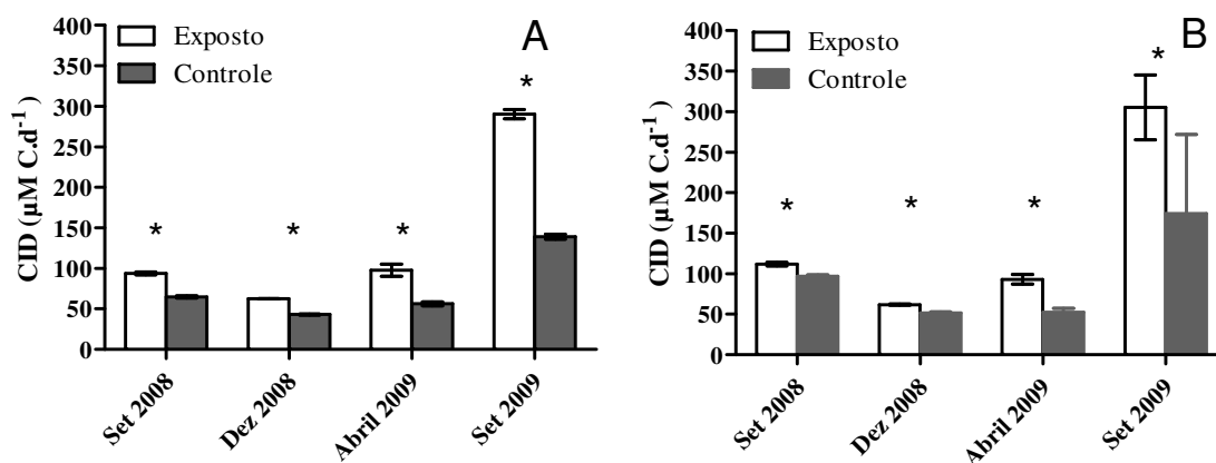
Figura 3- Concentrações de CID ( \mu\text{M C} ) para o Rio Negro (A) e lago Tupé (B) nos tratamentos expostos e controles nos quatro períodos amostrados. Asteriscos representam diferenças significativas entre os tratamentos ( p < 0.05 ). Barras de erro representam desvio padrão da média.
