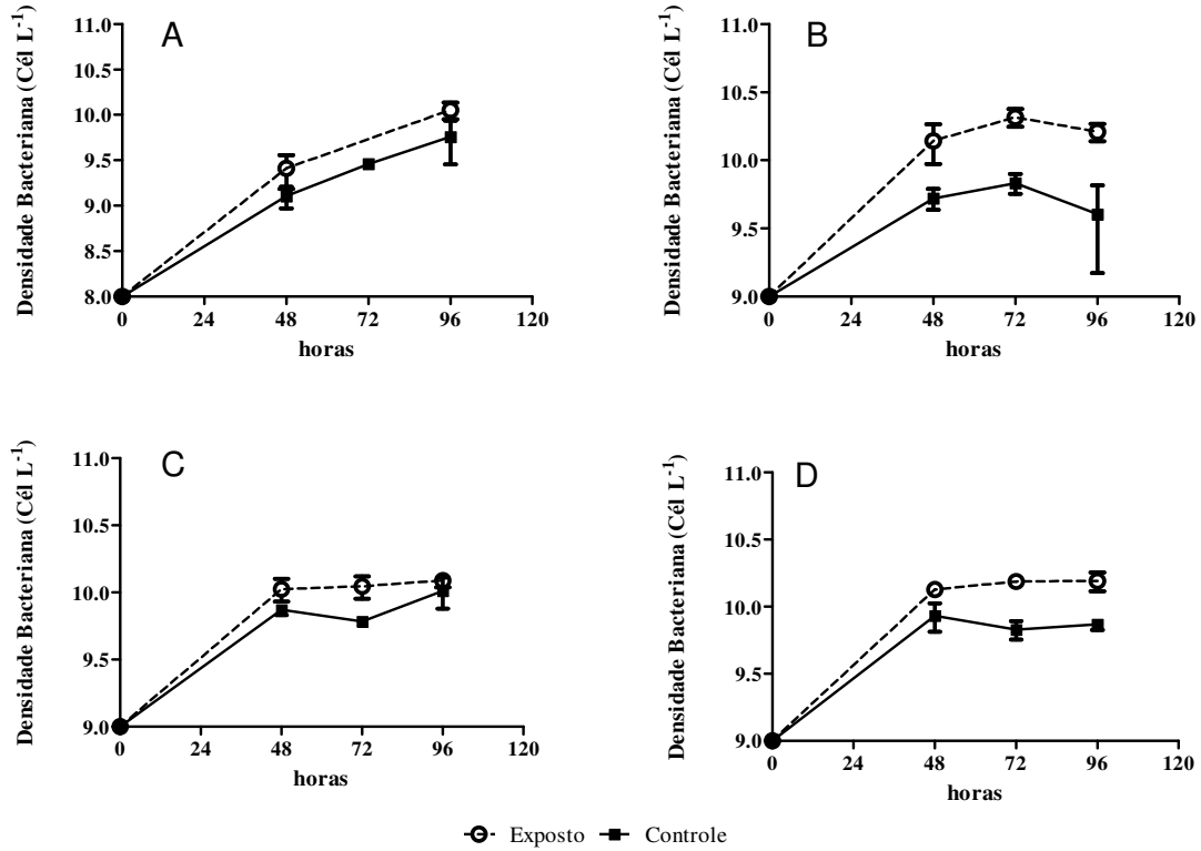
Figura 6- Curvas de crescimento densidade bacteriana ( 10^x células por litro) nos tratamentos Expostos e Controles para o Rio Negro em (A) setembro/vazante 2008 (B) dezembro/seca de 2008 (C) abril/cheia de 2009 e (D) setembro/vazante de 2009. As barras de erro representam o desvio padrão da média.
