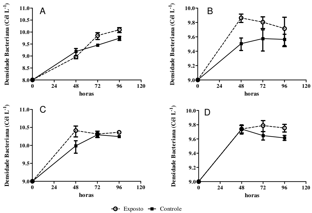
Figura 7- Curvas de crescimento, densidade bacteriana ( 10^x células por litro) nos tratamentos Expostos e Controles para o lago Tupé em (A) setembro/vazante 2008 (B) dezembro/seca de 2008 (C) abril/cheia de 2009 e (D) setembro/vazante de 2009. As barras de erro representam o desvio padrão da média.
