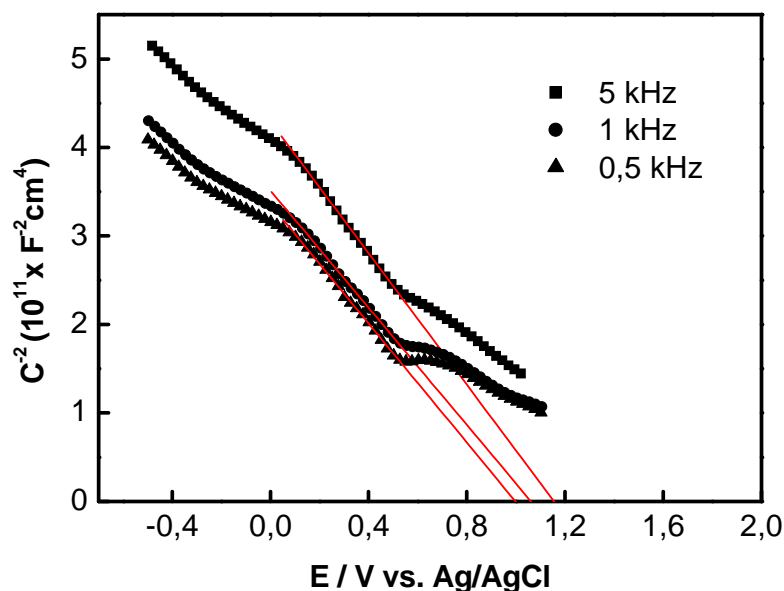
Figura 4.5: Curva Mott-Schottky para eletrodo de DDB em 0,5 \text{ mol L}^{-1} \text{ H}_2\text{SO}_4 e frequência de 5, 1, e 0,5 kHz, respectivamente.
