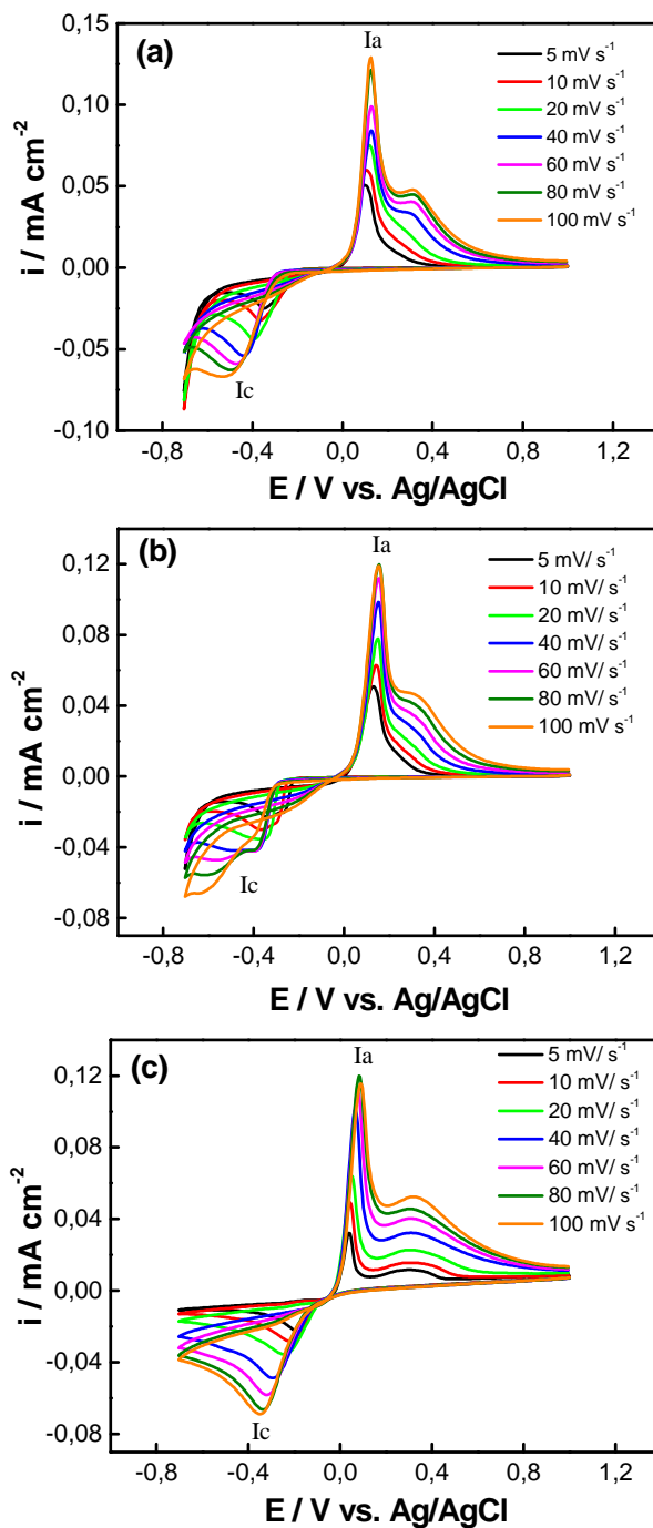
Figura 4.9: Voltamogramas cíclicos dos processos de deposição e dissolução de Cu sobre o eletrodo de DDB em meio de (a) 0,1 \text{ mol L}^{-1} \text{ H}_2\text{SO}_4 + 10^{-3} \text{ mol L}^{-1} \text{ CuSO}_4 , (b) 0,1 \text{ mol L}^{-1} \text{ HClO}_4 + 10^{-3} \text{ mol L}^{-1} \text{ CuSO}_4 e (c) 0,5 \text{ mol L}^{-1} \text{ Na}_2\text{SO}_4 + 10^{-3} \text{ mol L}^{-1} \text{ CuSO}_4 , em diferentes velocidades de varredura.
