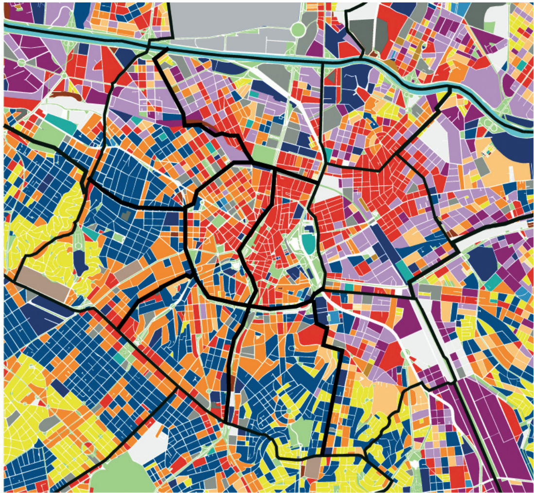
Figura 4. Mapa de uso do solo
