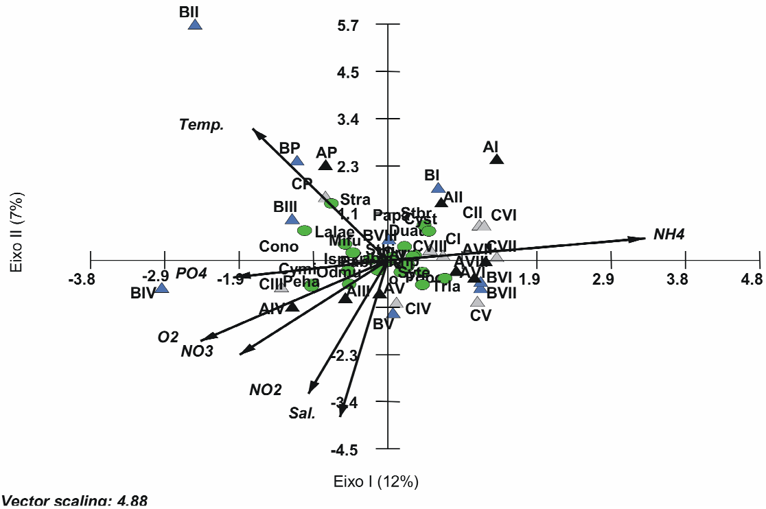
Vector scalina: 4.88 Figura 26. Diagrama fatorial resultante da análise de correspondência canônica evidenciando as 23 espécies mais abundantes em número de indivíduos e mais freqüentes ( > 65\% ) nas campanhas (P = pré-monitoramento e I a VIII = campanhas de monitoramento) e das variáveis ambientais temperatura, salinidade, oxigênio dissolvido, nitrito, nitrato, amônia e fosfato no recife Orion (área A) e nas áreas controle B e C. As espécies Cynoscion striatus (Cyst), Porichthys porosissimus (Popo), Symphurus tessellatus (Syte), Trachurus lathami (Trla), Conodon nobilis (Cono), Pellona harroweri (Peha), Cynoscion microlepidotus (Cymi) e Stellifer rastrifer (Stra) foram as que se destacaram, apresentando correspondência com relação às variáveis ambientais.
