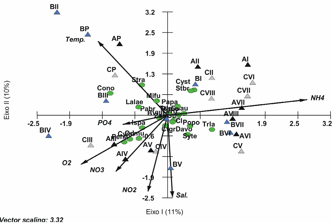
Figura 27. Diagrama fatorial resultante da análise de correspondência canônica evidenciando a biomassa das 23 espécies mais abundantes em número de indivíduos e mais freqüentes (> 65%) nas campanhas (P = pré-monitoramento e I a VIII = campanhas de monitoramento) e das variáveis ambientais temperatura, salinidade, oxigênio dissolvido, nitrito, nitrato, amônia e fosfato no recife Orion (área A) e nas áreas controle B e C. As espécies Trachurus lathami (Trla), Porichthys porosissimus (Popo), Symphurus tessellatus (Syte), Cynoscion striatus (Cyst), Conodon nobilis (Cono), Pellona harroweri (Peha) e Cynoscion microlepidotus (Cymi) foram as que se destacaram, apresentando correspondência com relação às variáveis ambientais.
