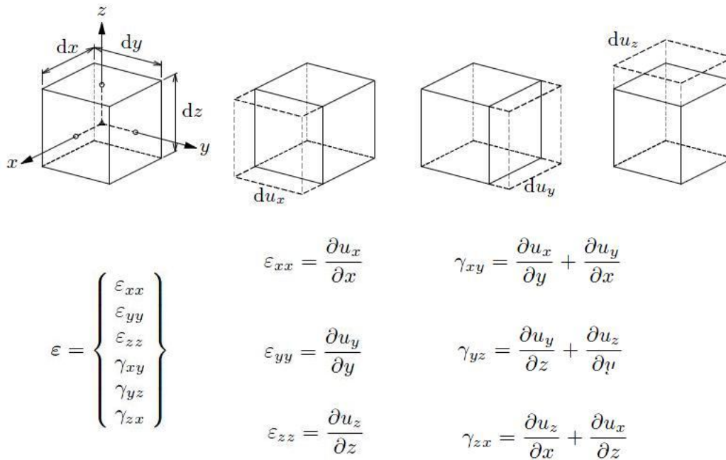
Figura 4.17 – Deformações do elemento sólido
