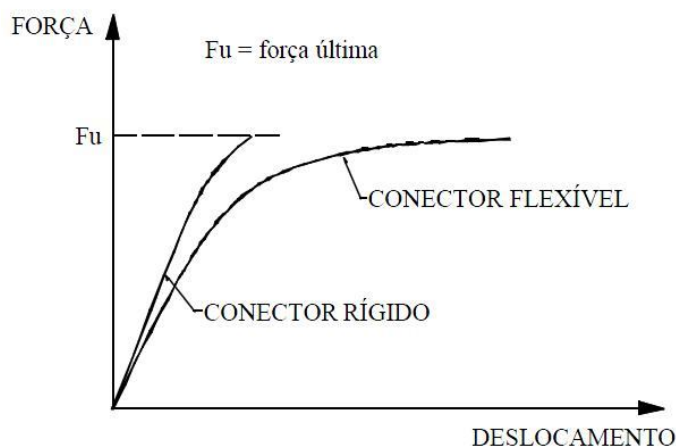
Figura 2.18 – Relação força-deslocamento para conectores de cisalhamento (ALVA, 2000)
