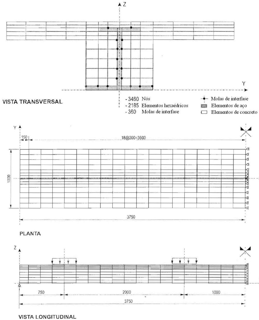
Figura 4.8 – Modelo de elementos finitos proposto por Paes (2003)
