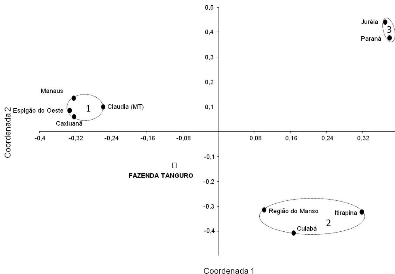
Figura 2. Diagrama de ordenação da Análise de Coordenadas Principais (PCO), baseada na composição de espécies de serpentes (presença e ausência de 171 espécies) de três taxocenoses de área abertas e quatro de áreas florestais. (1) Taxocenoses em regiões amazônicas (Manaus: Martins & Oliveira 1998, Caxiuanã: Maschio et al. 2009, Espigão do Oeste: Bernarde & Abe 2006, Claudia, MT: Carvalho 2006); (2) Taxocenoses em áreas do Cerrado (Região do Manso: Strüssmann 2000, Cuiabá: Carvalho & Nogueira, 1998, Itirapina: Sawaya 2008); (3) Taxocenoses da Mata Atlântica (Juréia: Marques 1998, Paraná: Morato 2005). O quadrado representa a área
