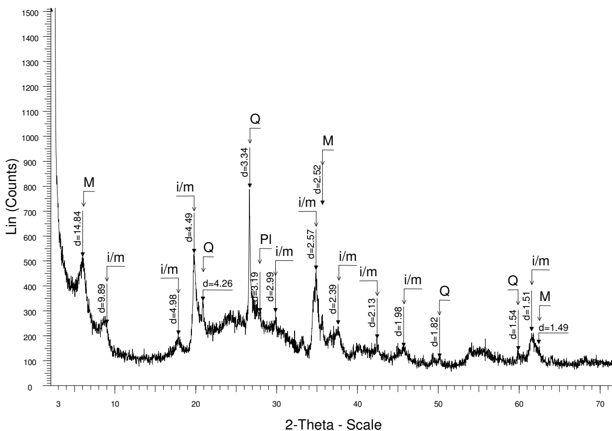
Figura 27 - Difratograma da fração < 0,5 µm na forma pulverizada e sem orientação: montmorilonita (M), ilita/mica (i/m) (dioctaédrica), plagioclásio (PI) e quartzo (Q).
