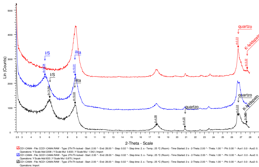
Figura 30 - Difratoogramas de uma amostra da mina de Meleiro mostrando a expansão na condição glicolada (em azul) de 14,64 Å para 16,04 Å evidenciando a identificação do interestratificado I/S
