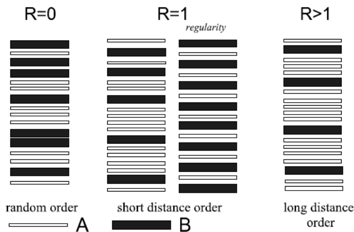
Figura 6 - Diagrama esquemático do ordenamento e regularidade de interestratificados tipo: R=0, R=1 e R>1 (Meunier, 2005).
