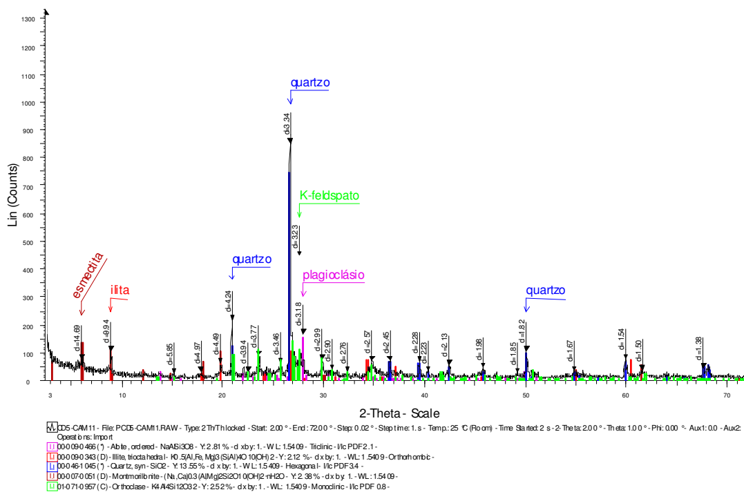
Figura 29 - Difratoograma de uma amostra de rocha total da mina de Meleiro.
