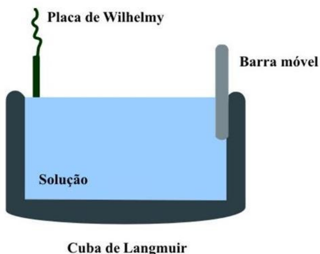
Figura 5 - Esquema da balança de Langmuir-Wilhelmy. A substância a ser testada é colocada como uma monocamada na superfície de uma solução contida na cuba de Langmuir. A tensão superficial é medida através da placa de Wilhelmy que está conectada a um transdutor de pressão. A área da superfície pode variar com o movimento da barra móvel. http://ising.phys.cwru.edu/surfactants/measurements.html
