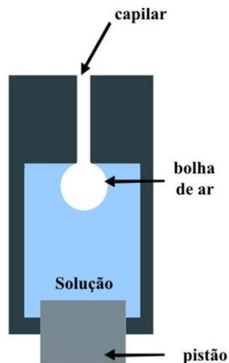
Figura 6 - Esquema do funcionamento do SBP. Uma bolha de 1,1 mm de diâmetro é formada a partir do capilar que está em contato com o ar atmosférico. O movimento do pistão comprime a bolha até um diâmetro de 0,8mm. Os movimentos repetidos do pistão fazem a bolha pulsar.
