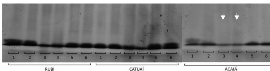
Figura 14 Perfis de bandas do sistema enzimático esterase, extraídos de sementes de café secas em secador, com e sem tratamento (1 e 2), não secas com e sem tratamento (3 e 4) e secas à sombra, com e sem tratamento químico (5 e 6) das cultivares Rubi, Catuai e Acaiá, após 12 meses de armazenamento.
