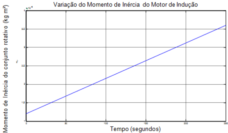
Figura 7.36 – Variação do Momento de Inércia em rampa com saturação de 3 \cdot J = 0.0036 Kg.m^2
