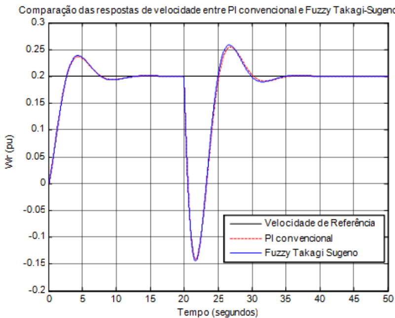
Figura 7.21 – Comparação das respostas de velocidade entre PI convencional e Fuzzy Takagi-Sugeno
