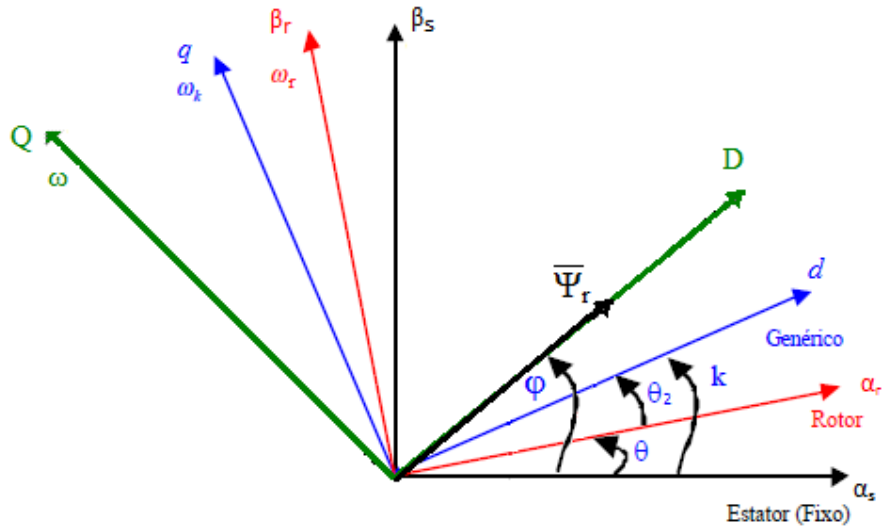
Figura 2.4 – Referencial sobre o fluxo rotórico.
