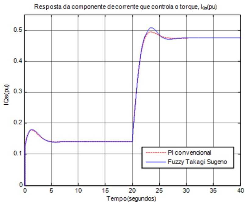
Figura 7.7 – Resposta da componente de corrente que controla o torque, I_{qs}(pu) , I_{base} = 1.589 A . A componente I_{qs} é representada em um referencial girante com o fluxo do rotor
