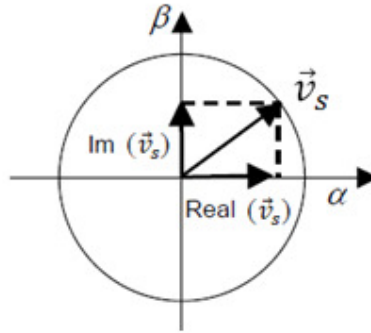
Figura 2.2 – Representação gráfica do sistema de eixos. Sistema bifásico com plano ortogonal complexo
