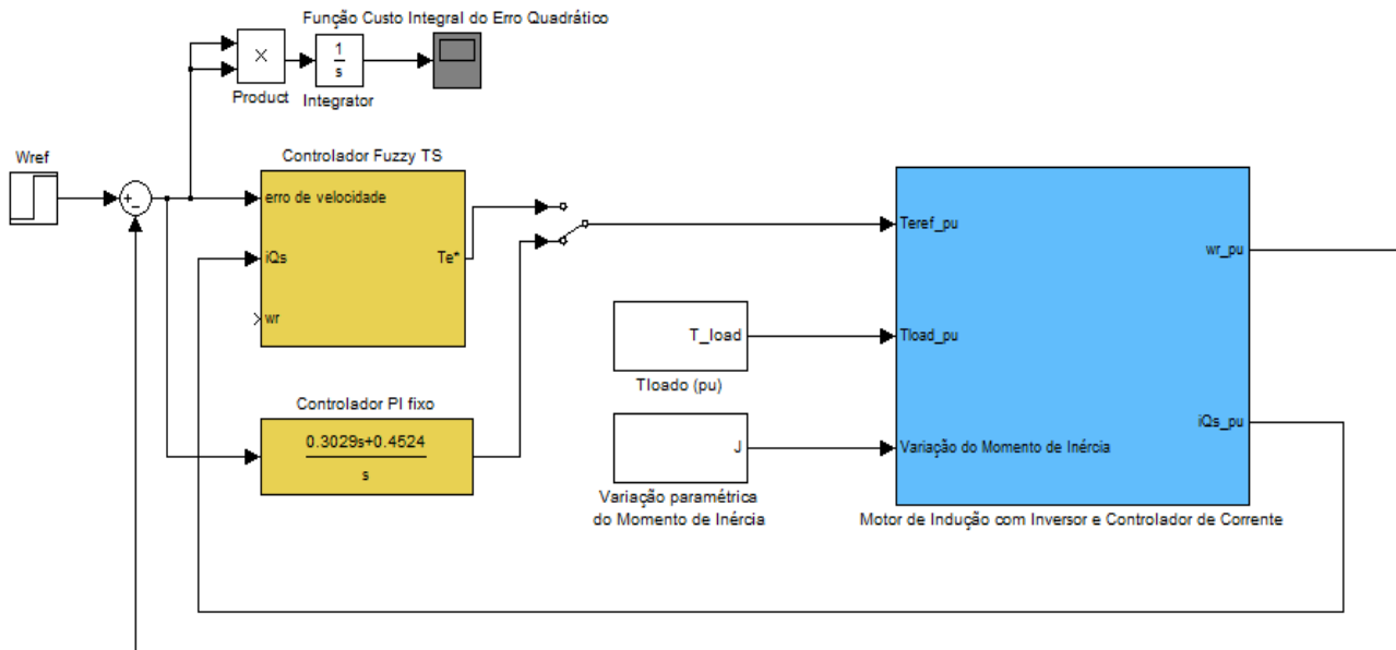
A.1 – Estrutura da Simulação utilizada para o controle de velocidade da planta motor de indução sob a ação de controladores de corrente
