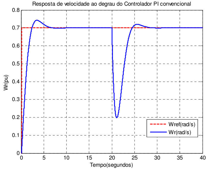
Figura 3.6 – Resposta de velocidade angular do controlador PI convencional ao degrau na velocidade de referência, W_{base} = 377 rad/s
