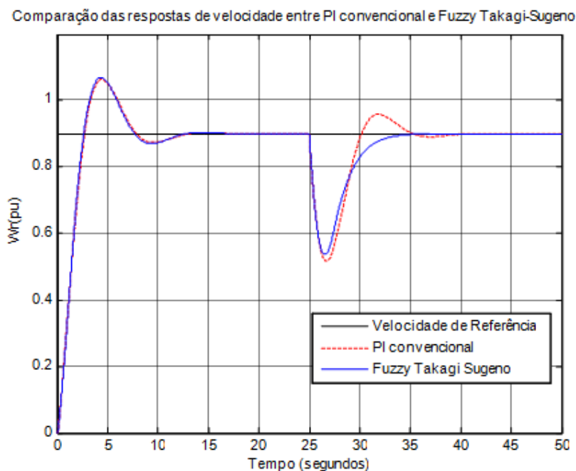
Figura 7.33 – Comparação das respostas de velocidade entre PI convencional e Fuzzy Takagi-Sugeno
