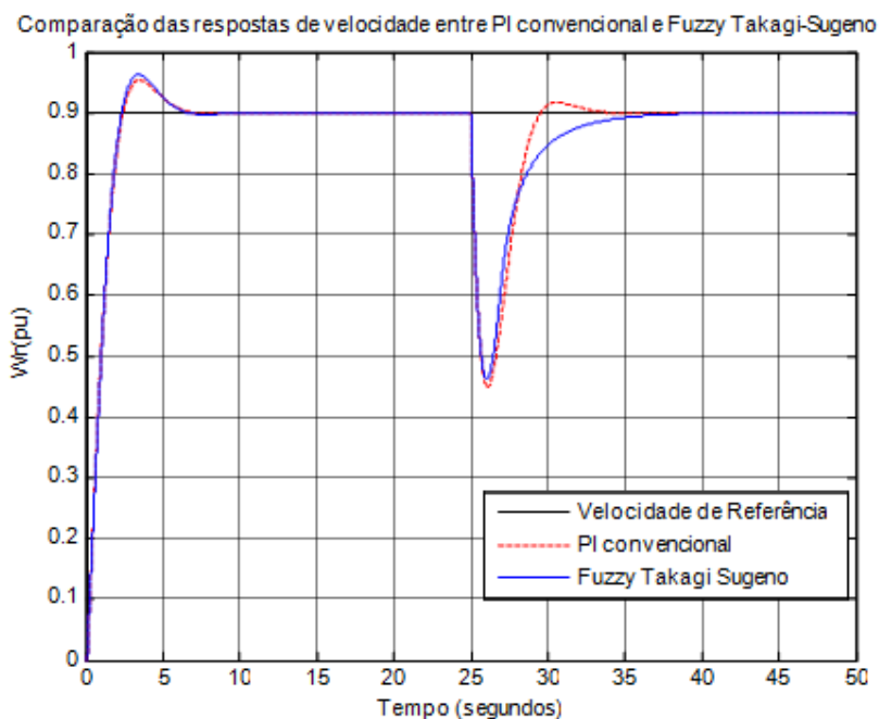
Figura 7.17 – Comparação das respostas de velocidade entre PI convencional e Fuzzy Takagi-Sugeno
