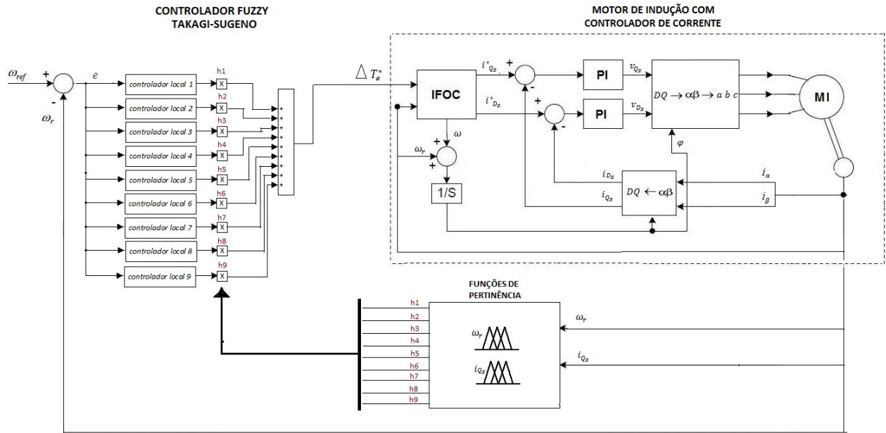
Figura 6.2 – Estrutura do Controlador Fuzzy Takagi-Sugeno para o Controle de Velocidade do Motor de Indução
