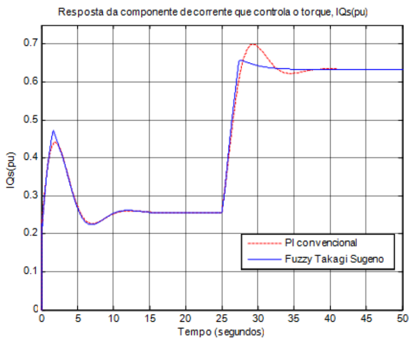
Figura 7.34 – Resposta da componente de corrente que controla o torque, I_{Qs}(pu) , I_{base} = 1.589 A . A componente I_{Qs} é representada em um referencial girante com o fluxo do rotor
