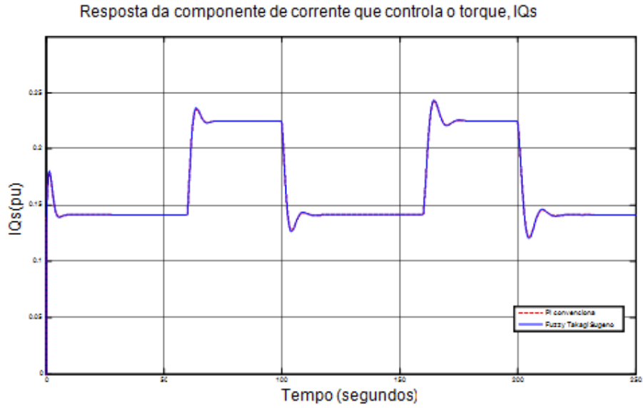
Figura 7.38 – Resposta da componente de corrente que controla o torque, I_{Qs} (pu), I_{base} = 1.589 A. A componente I_{Qs} é representada em um referencial girante com o fluxo do rotor
