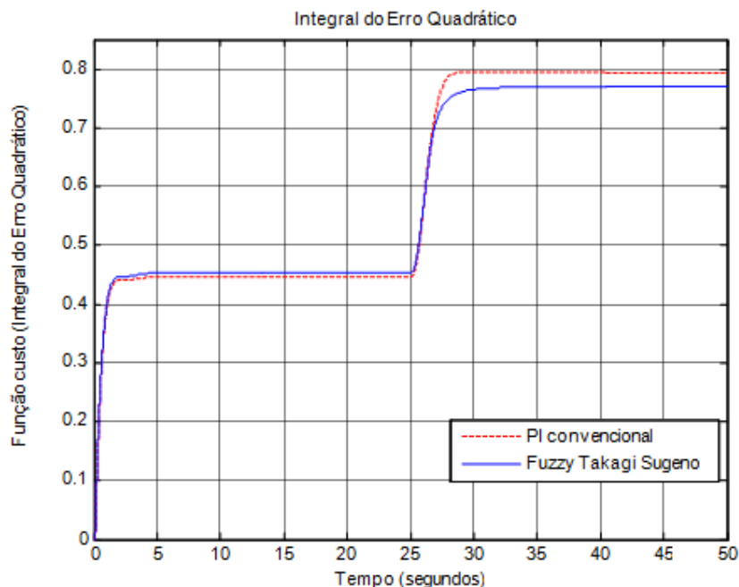
Figura 7.19 – Função custo, integral do erro quadrático
