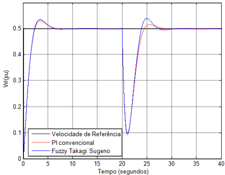
Comparação das respostas de velocidade entre PI convencional e Fuzzy Takagi-Sugeno
