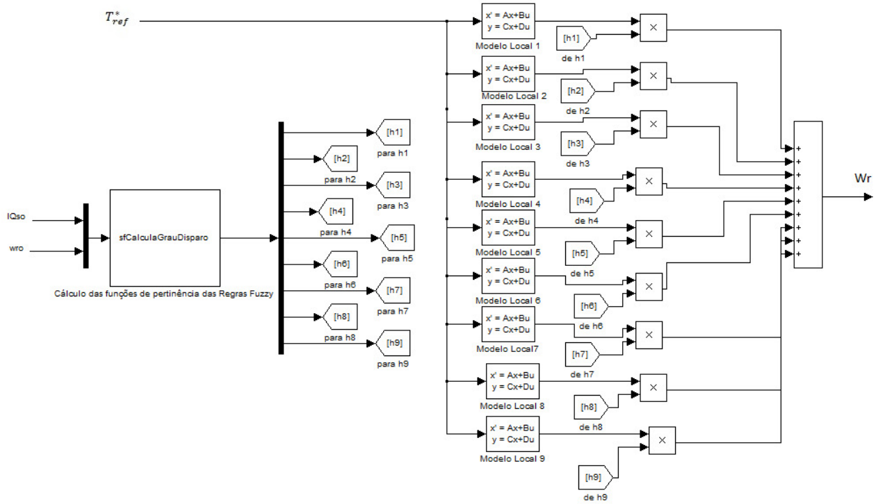
Figura 5.7 – Diagrama de Blocos da Modelagem Fuzzy Takagi_Sugeno
