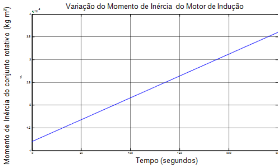
Figura 7.40 – Variação do Momento de Inércia em rampa com saturação de 3 \times J = 0.0036 Kg.m^2
