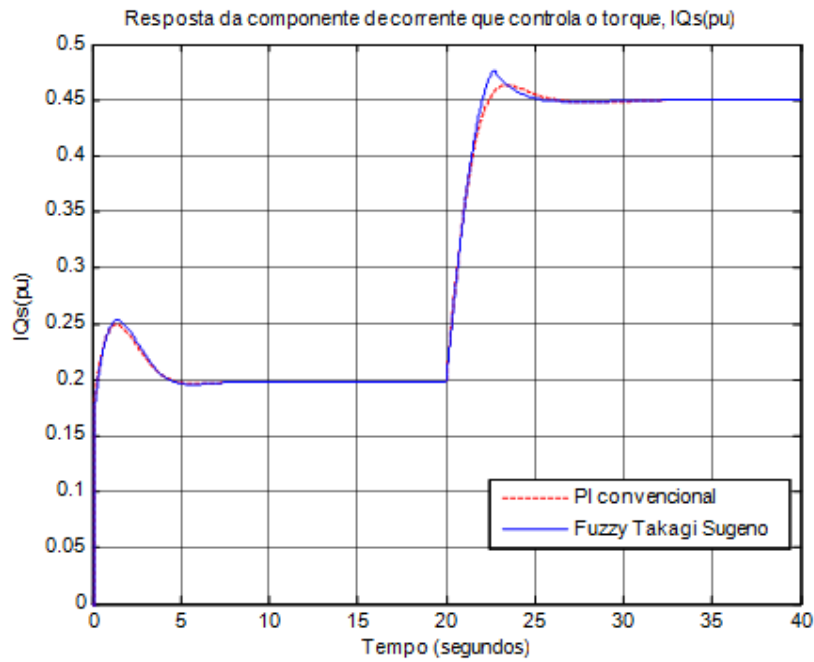
Figura 7.10 – Resposta da componente de corrente que controla o torque, I_{Qs} (pu), I_{base} = 1.589 A. A componente I_{Qs} é representada em um referencial girante com o fluxo do rotor
