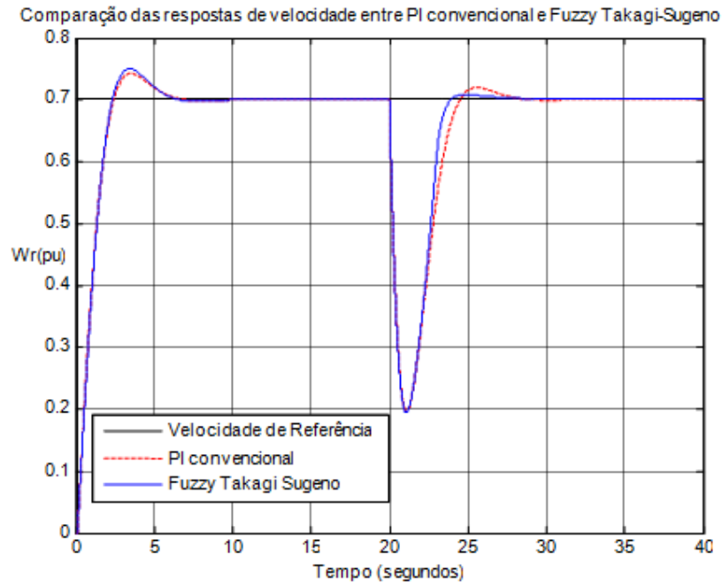
Figura 7.14 – Comparação das respostas de velocidade entre PI convencional e Fuzzy Takagi-Sugeno
