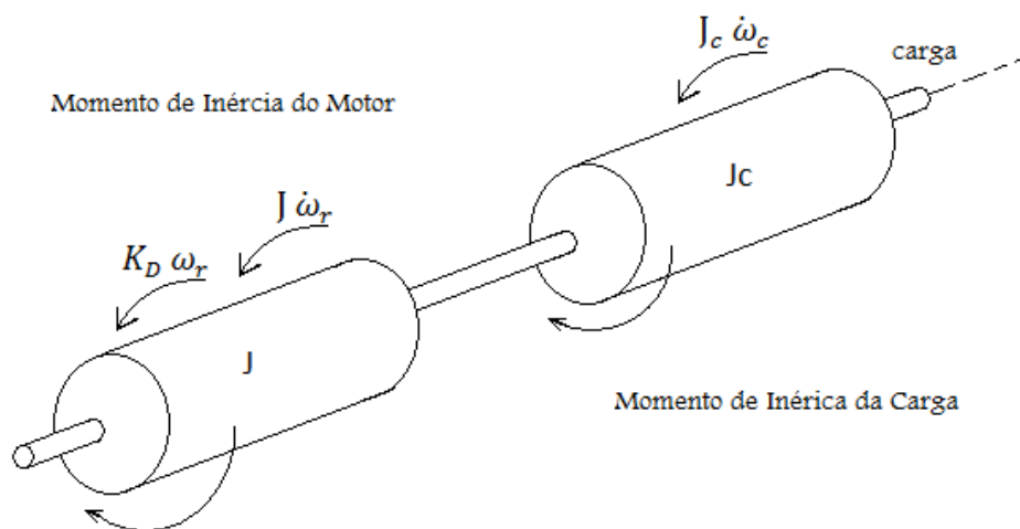
Figura 7.20 – Momento de Inércia do conjunto motor mais carga
