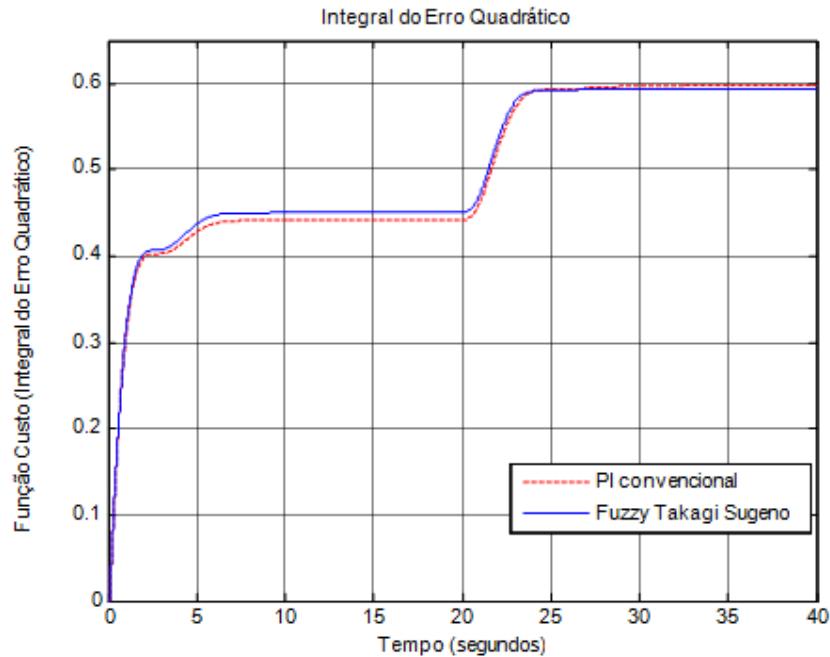
Figura 7.11 – Função Custo, Integral do erro quadrático
