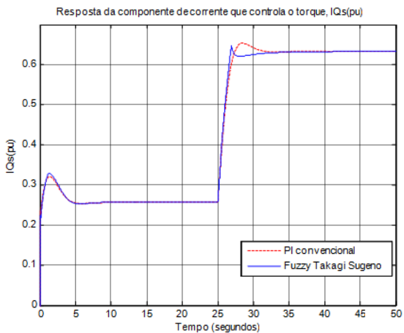
Figura 7.18 – Resposta da componente de corrente que controla o torque, I_{Qs}(pu) , I_{base} = 1.589 A . A componente I_{Qs} é representada em um referencial girante com o fluxo do rotor
