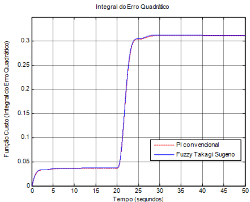
Figura 7.23 – Função custo, integral do erro quadrático
