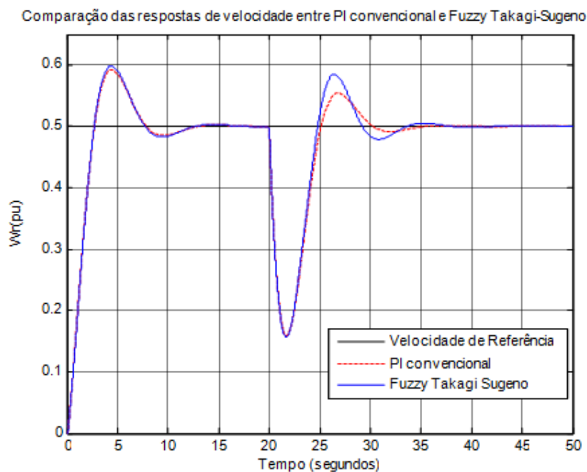
Figura 7.24 – Comparação das respostas de velocidade entre PI convencional e Fuzzy Takagi-Sugeno
