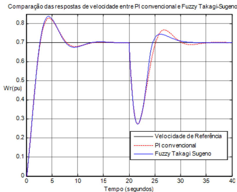
Figura 7.30 – Comparação das respostas de velocidade entre PI convencional e Fuzzy Takagi-Sugeno
