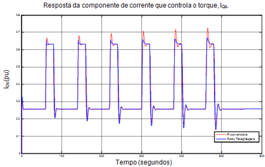
Figura 7.43 – Resposta da componente de corrente que controla o torque, I_{Qs} (pu), I_{base} = 1.589 A. A componente I_{Qs} é representada em um referencial girante com o fluxo do rotor
