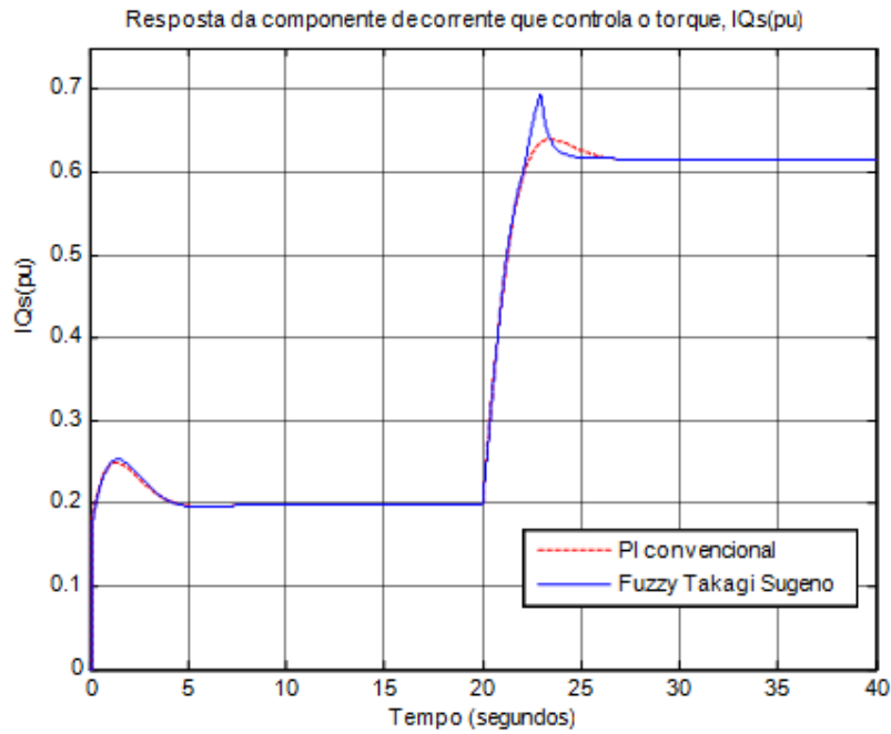
Figura 7.15 – Resposta da componente de corrente que controla o torque, I_{Qs} (pu), I_{base} = 1.589 A. A componente I_{Qs} é representada em um referencial girante com o fluxo do rotor
