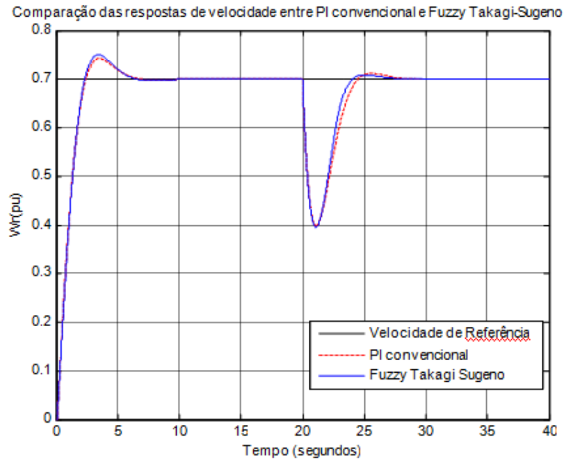
Figura 7.9 – Comparação das respostas de velocidade entre PI convencional e Fuzzy Takagi-Sugeno
