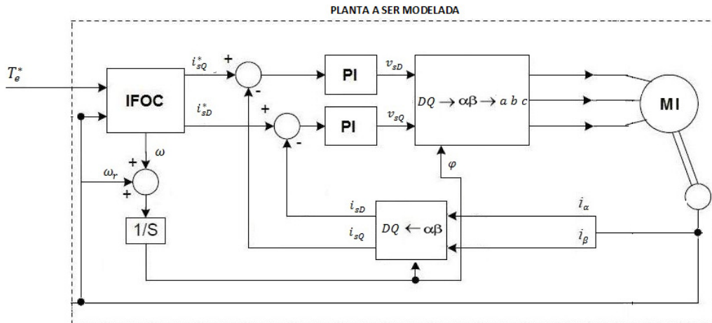
Figura 5.1 – Diagrama de Blocos da planta a ser modelada por fuzzy Takagi-Sugeno.
