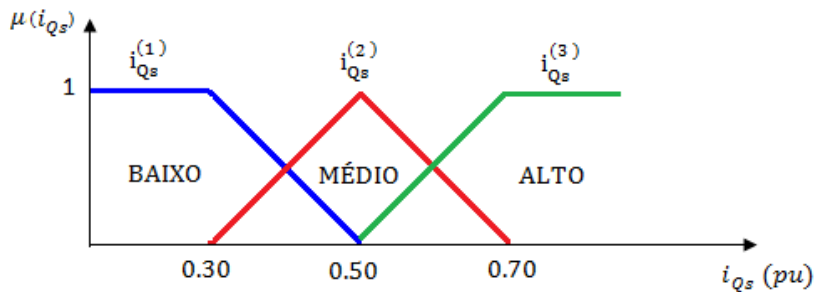
Figura 5.4 – Conjuntos Fuzzy para a componente da corrente de estator responsável pelo controle do torque elétrico do motor i_{Qs} , em pu em relação à corrente nominal do motor
