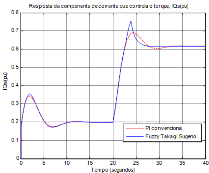
Figura 7.31 – Resposta da componente de corrente que controla o torque, IQs(pu), Ibase = 1.589 A. A componente IQs é representada em um referencial girante com o fluxo do rotor
