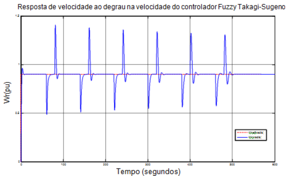
Figura 7.41 – Resposta de velocidade angular do controlador Fuzzy Takagi-Sugeno ao degrau na velocidade de referência, W_{rbase} = 377 \text{ rad/s}
