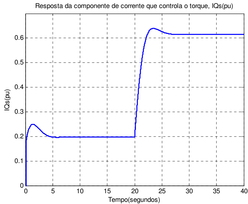
Figura 3.7 – Resposta da componente de corrente que controla o torque, I_{Qs} (pu), I_{base} = 1.589 A. A componente I_{Qs} é representada em um referencial girante com o fluxo do rotor
