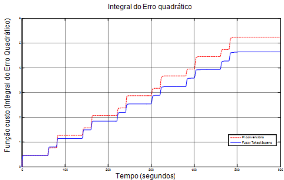
Figura 7.44 – Função custo, integral do erro quadrático
