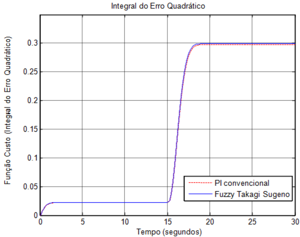
Figura 7.5 – Função Custo, Integral do Erro Quadrático
