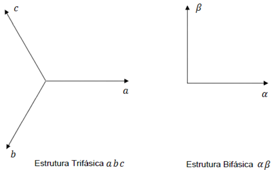
Figura 2.1 – Representação no eixo alfa beta
