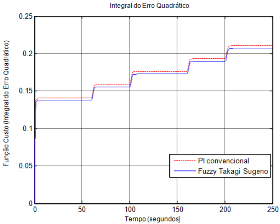
Figura 7.39 – Função custo, integral do erro quadrático
