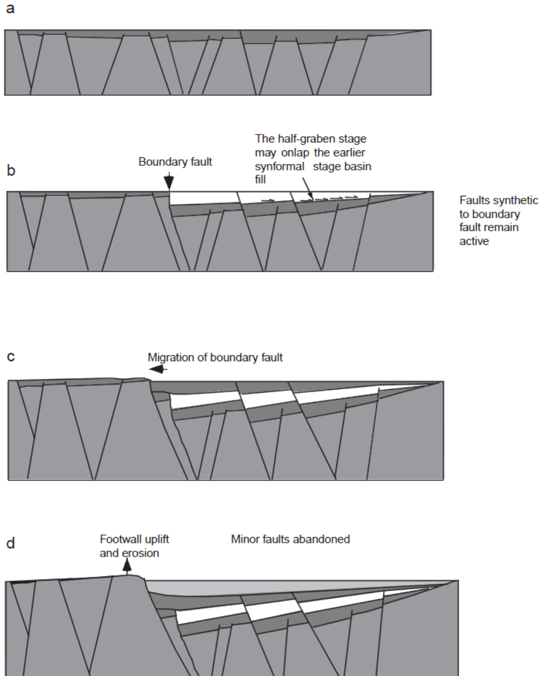
Figura 33: Seções esquemáticas do modelo evolutivo de riftes de Morley (2002), com o (a) estágio rifte inicial (depressão sinforme – ex. Usangu Flats), (b) meio-gráben inicial, (c) meio-gráben maturo, e (d) final do meio-gráben.
