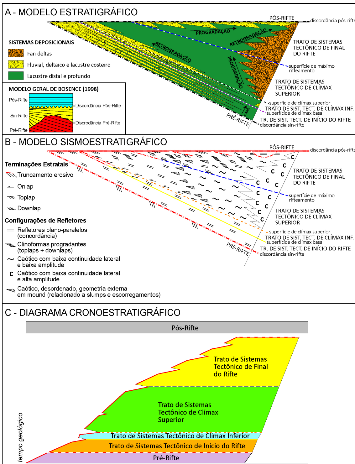
Figura 38: A: Modelo estratigráfico idealizado de uma bacia rifte, com os tratos de sistemas tectônicos, superfícies limítrofes, arranjo dos sistemas deposicionais e padrões de empilhamento (extraído de Kuchle & Scherer, 2010). B: Transposição do modelo estratigráfico de tratos de sistemas tectônicos (A) para a terminologia sismoestratigráfica, com os tratos de sistemas tectônicos, suas superfícies limítrofes, terminações estratiais e configurações de refletores idealizados para cada trato de sistemas tectônico. C: diagrama cronoestratigráfico (diagrama de Wheeler) com o arranjo temporal dos tratos de sistemas tectônicos derivados das figuras A e B. Extraído do Artigo 2.
