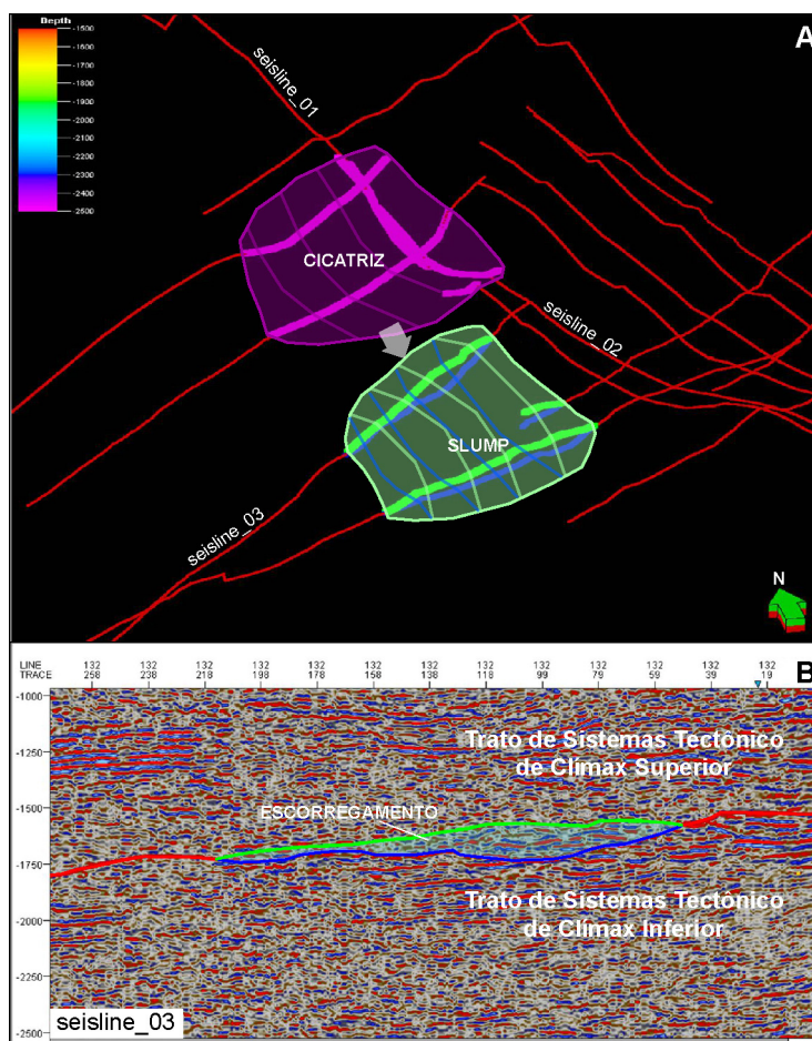
Figura 7 A: Mapeamento em diversas linhas da cicatriz observada no topo do Trato de Sistemas Tectônico de Clímax Basal, e da feição de escorregamento (slump) próxima a ela. B: detalhe da linha seisline_03 (localizada no quadro A) onde observa-se a feição de escorregamento (ou deslizamento) mapeada tridimensionalmente e interpretada como o depósito de fluxo associado a cicatriz adjacente, indicando um deslocamento completo do depósito.
