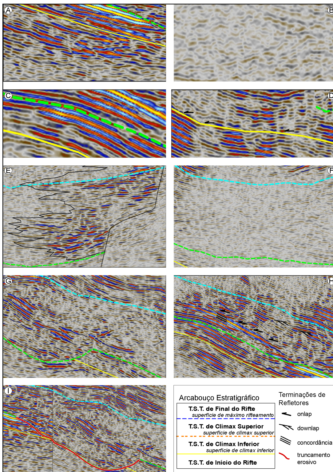
Figura 5: Quadros de detalhe da composição sísmica mostrando feições específicas dos padrões de refletores, terminações, estruturação interna e externa das unidades sismoestratigráficas, tratos de sistemas tectônicos e superfícies limitrofes, conforme descrito no texto.
