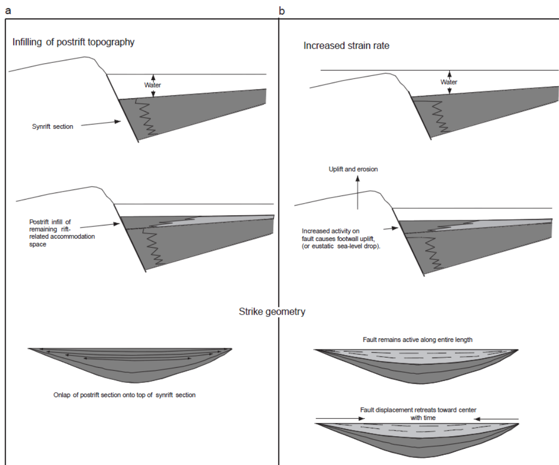
Figura 34: Modelo esquemático de Morley (2002) mostrando a problemática de definição do final da fase rifte, onde uma situação de (a) preenchimento “pós-rifte” do espaço criado durante a fase rifte, sem atividade tectônica no pós-rifte, pode apresentar a mesma assinatura deposicional de (b) uma reativação tectônica tardia do rifte ou rebaixamento do nível do lago, implicando em registros sedimentares semelhantes.
