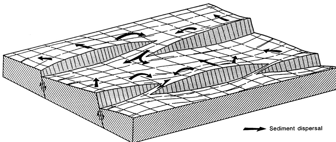
Figura 14: Exemplo de terminações laterais de falha de borda, com zonas de transferência, gerando as rampas de revezamento ( relay ramps ), que controlam as principais entradas de sedimentos em sistemas de meio-grábens adjacentes (transporte indicado pelas setas). Extraído de Ravnás & Steel (1998).
