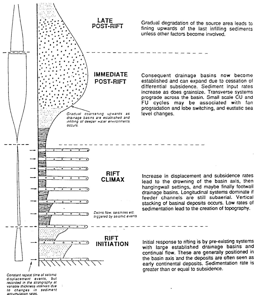
Figura 25: Sucessão estratigráfica vertical idealizada, apresentando os padrões de empilhamento e sistemas deposicionais para os respectivos tratos tectônicos formadores da fase rifte de uma bacia. Extraído de Prosser (1993).
