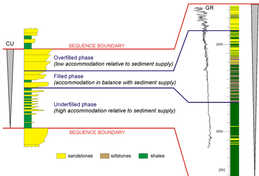
Figura 35: Arquitetura de uma seqüência rifte completa, conforme Martins-Neto & Catuneanu (2010), apresentando os ciclos de gradação normal ( coarsening upward cycles ) e as fases de subpreenchimento, preenchimento equilibrado e superpreenchimento ( underfilled, filled e overfilled phases , respectivamente).
