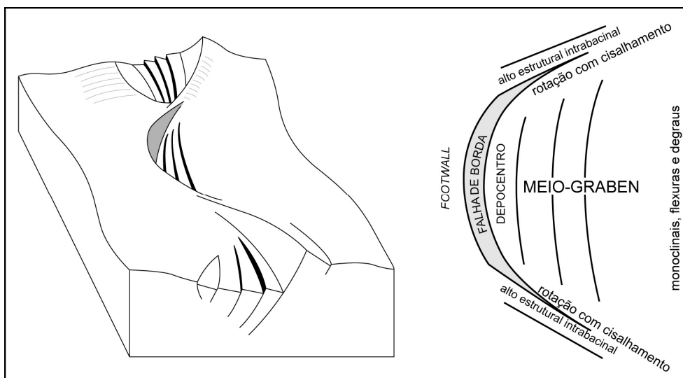
Figura 10: Modelo de meio-gráben com terminações laterais em zonas de transferência, com depocentro bem definido e com inversão de sentido e arqueamento da falha de borda, gerando assim uma sucessão de meio-grábens rotacionados (modif. de Rosendahl et al. , 1986).
