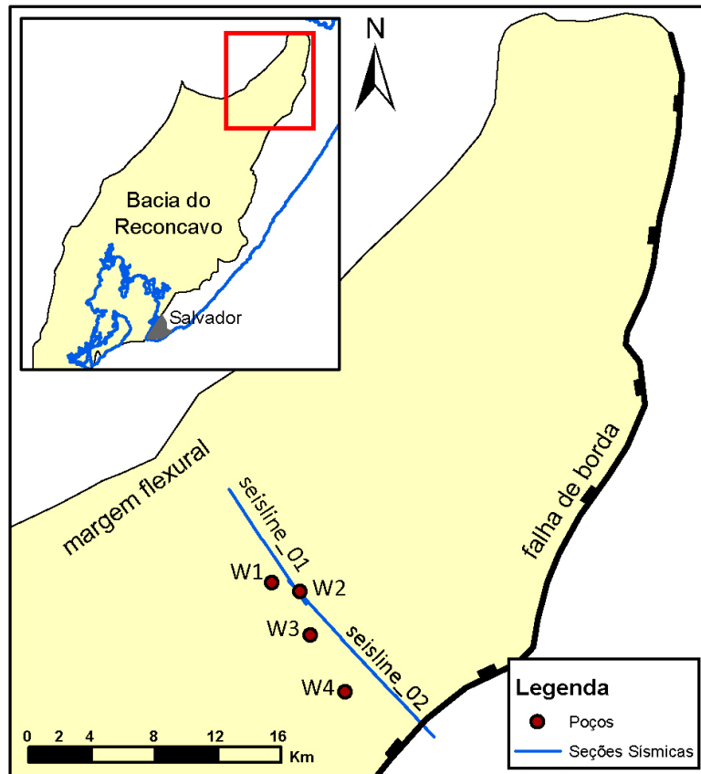
Figura 02: Mapa de localização da Bacia do Recôncavo, mostrando a composição de linhas sísmicas 2D utilizada, os poços relacionados e a principal estruturação da calha do Recôncavo, com a forma de um meio-gráben alongado a NE, com falha de borda a leste e margem flexural a oeste.
