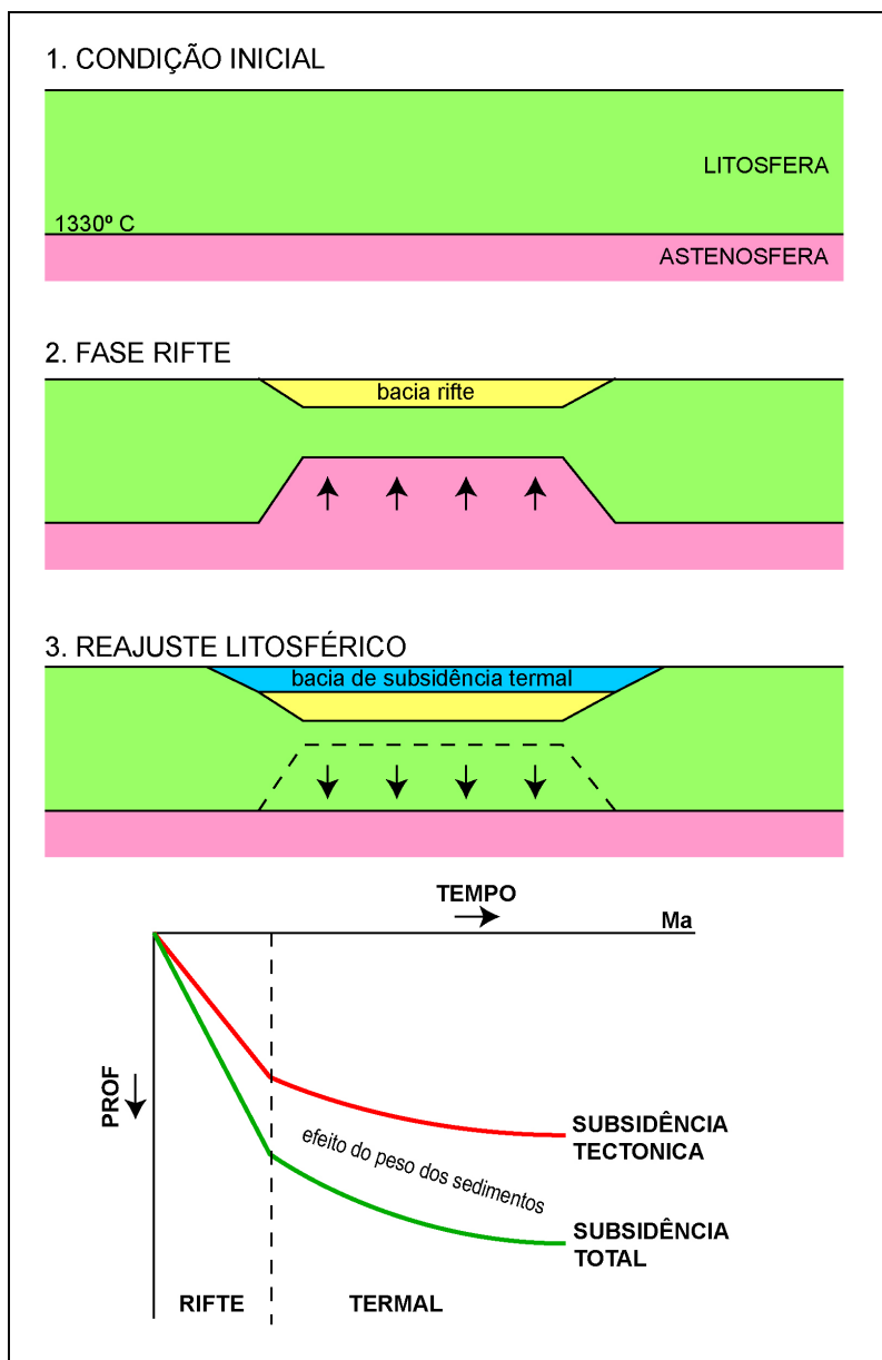
Figura 3: Modelo evolutivo geodinâmico de rifteamento modificado de Dewey (1988, baseado no modelo de Mackenzie, 1978), onde a partir de uma condição inicial (1), onde existe um equilíbrio entre litosfera e astenosfera (isoterma de 1330° C horizontal), a fase rifte (2) é gerada por uma ascensão astenosférica que gera um afinamento crustal e desenvolvimento da bacia rifte. Ao final da subsidência rifte, ocorre o reequilíbrio térmico com retorno da isoterma 1330°C á sua posição original. O resfriamento e conseqüente espessamento da litosfera induzem uma nova fase de subsidência (neste caso, termal) na área afinada. Assim, a curva de subsidência tectônica apresenta uma fase rifte de alta taxa e uma fase posterior termal, de baixa e decrescente taxa (curva vermelha). A esta curva deve-se adicionar o componente de carga sedimentar (peso dos sedimentos), que deprime flexuralmente a litosfera afinada (resultando na curva verde).
