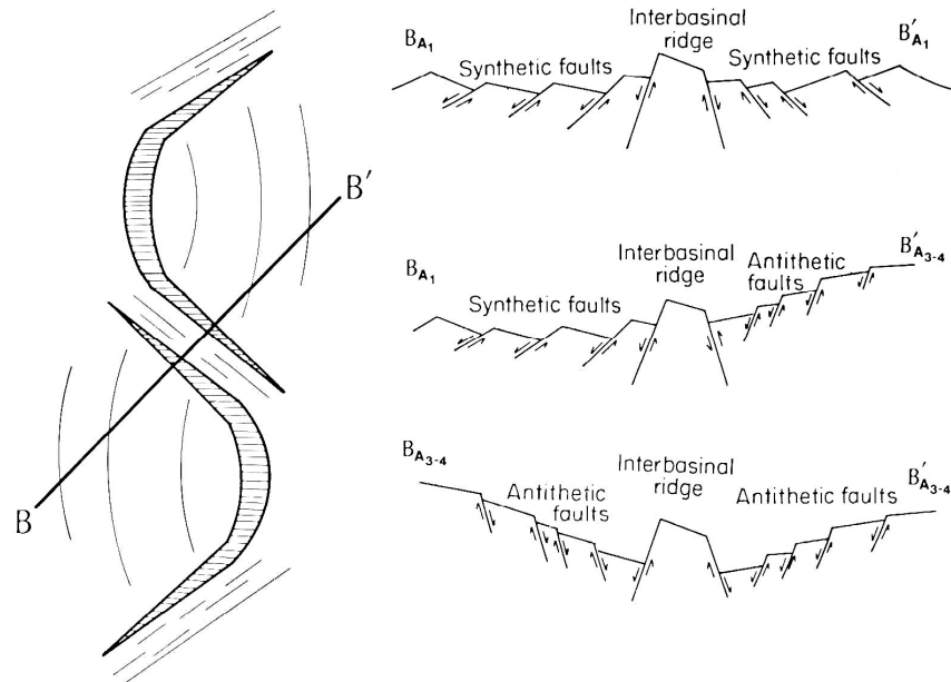
Figura 12: Variações morfológicas das bacias geradas pelo desenvolvimento de sistemas de meio-grábens inversos e conectados, gerando assim, altos estruturais internos à bacia, associados a zonas de transferência. Extraído de Rosendahl et al. (1986).
