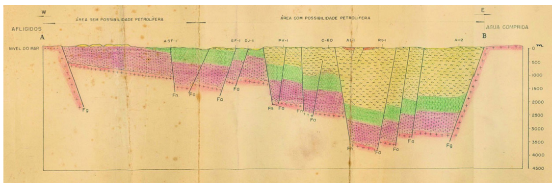
Figura 7: Seção geológica regional da Bacia do Recôncavo, desenvolvida na década de 1950, ilustrando a interpretação de um tectonic though . Extraído de Moura & Fernandes (1952).
