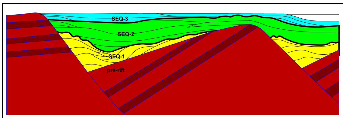
Figura 20: Modelo de evolução estratigráfica proposto por Bosence (1998), em uma sub-bacia formada por meio-grábens: na seqüência 1 há, de modo síncrono, onlap, agradação e downlap na área do hangingwall , e erosão/formação de limite de seqüências na área do footwall , devido a subsidência diferencial causada pela falha rotacional do bloco. A seqüência 2 exhibe inicialmente um onlap do hangingwall para o footwall . O limite de seqüências 3 se origina em resposta a rotação de blocos com soerguimento no footwall em sincronia com subsidência no hangingwall . (Extraído de Bosence, 1998).
