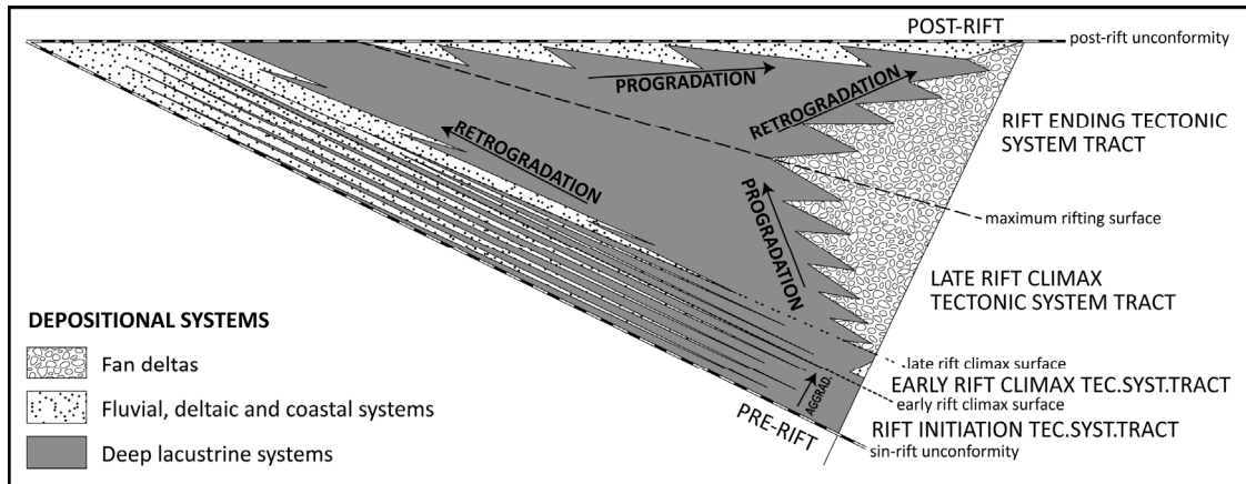
Figura 36: Modelo idealizado dos tratos de sistemas tectônicos propostos na presente tese, com seus respectivos padrões de empilhamentos (na margem flexural e na falha de borda) e superfícies limítrofes. Extraído do Artigo 1.
