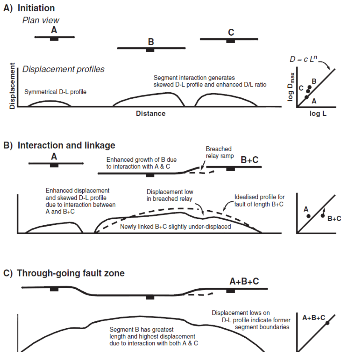
Figura 26: Modelo esquemático de Gawthorpe & Leeder (2000) para o processo de conexão de falhas ( fault linkage ), que controla o desenvolvimento de falhamentos em um rifte, principalmente a falha de borda. Observa-se que no início (A) as falhas apresentam pouco rejeito e pequena extensão lateral. A conectividade lateral (B) faz gradualmente aumentar a extensão do falhamento e seu rejeito até a fase de amplo estabelecimento (C).
