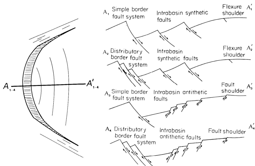
Figura 11: Variações morfológicas do sistema de falhamentos internos em um meio-gráben individual, podendo este ocorrer como uma simples falha-mestra, ou como um sistema de falhas distributárias. Também, o sistema de falhamentos interno pode ser sintético, ou antitético. Extraído de Rosendahl et al. (1986).
