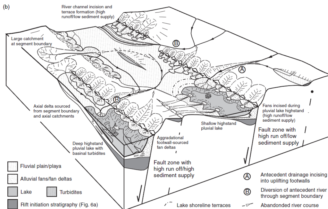
Figura 29: Modelo evolutivo de Gawthorpe & Leeder (2000) para a fase de interação e conexão de falhas, onde os meio-grábens se desenvolvem, ganham extensão lateral, inicia-se o desenvolvimento de lagos e ocorrem inflexões da drenagem.
