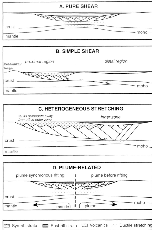
Figura 2: Modelos geodinâmicos propostos para a evolução de bacias rifte. (A): modif. de McKenzie (1978); (B): modif. de Wernicke & Burchfiel (1982); (C): modif. de Coward (1986); (D): modif. de White & McKenzie (1989). Extraído de Bosence (1998).
