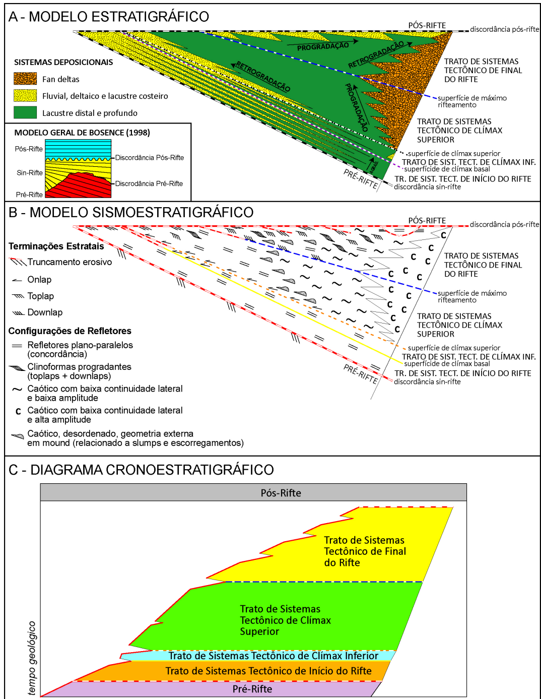
Figura 01 A: Modelo estratigráfico idealizado de uma bacia rifte, com os tratos de sistemas tectônicos, superfícies limitrofes, arranjo dos sistemas deposicionais e padrões de empilhamento (extraído de Kuchle & Scherer, 2010). B: Transposição do modelo estratigráfico de tratos de sistemas tectônicos (A) para a terminologia sismoestratigráfica, com os tratos de sistemas tectônicos, suas superfícies limitrofes, terminações estratais e configurações de refletores idealizados para cada trato de sistemas tectônico. C: diagrama cronoestratigráfico (diagrama de Wheeler) com o arranjo temporal dos tratos de sistemas tectônicos derivados das figuras A e B.
