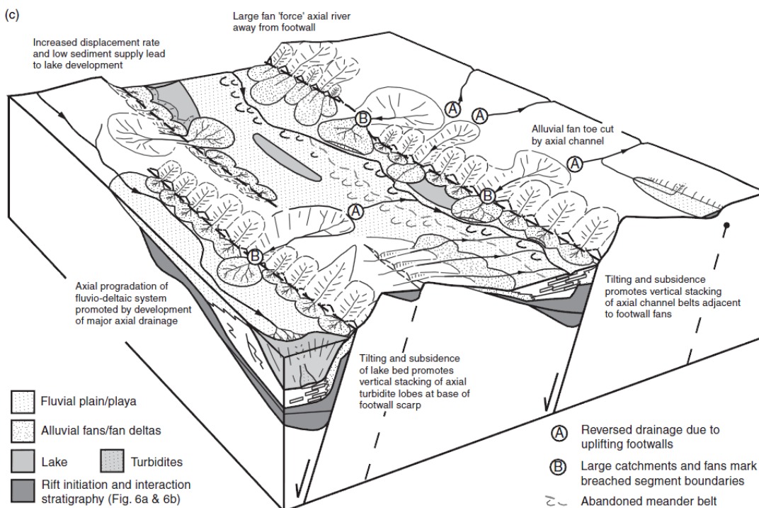
Figura 30: Modelo evolutivo de Gawthorpe & Leeder (2000) para a fase de estabelecimento do meio-grábem, onde a atividade tectônica diminui, o sistema de drenagem é fixado e começa efetivamente a transportar sedimentos preenchendo os meio-grábens.
