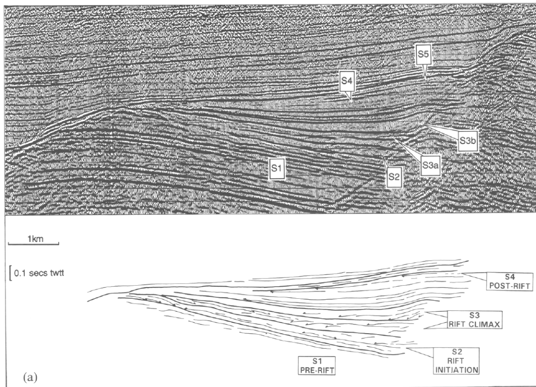
Figura 23: Linha sísmica e interpretação no rifte do Mar de Barents, extraído de Prosser (1993). Observar a fase de início do rifte ( rift initiation , S2), que apresenta na margem flexural (à esquerda) truncamentos erosivos, indicando uma área deposicional maior que o meio-gráben posteriormente desenvolvido.
