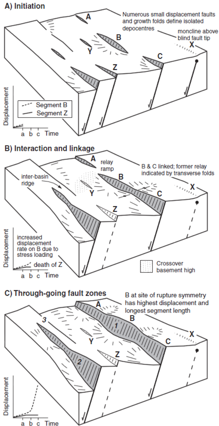
Figura 27: Blocos diagrama apresentando o modelo evolutivo da conexão de falhas conforme apresentado na Figura 26 (anterior). Extraído de Gawthorpe & Leeder (2000).
