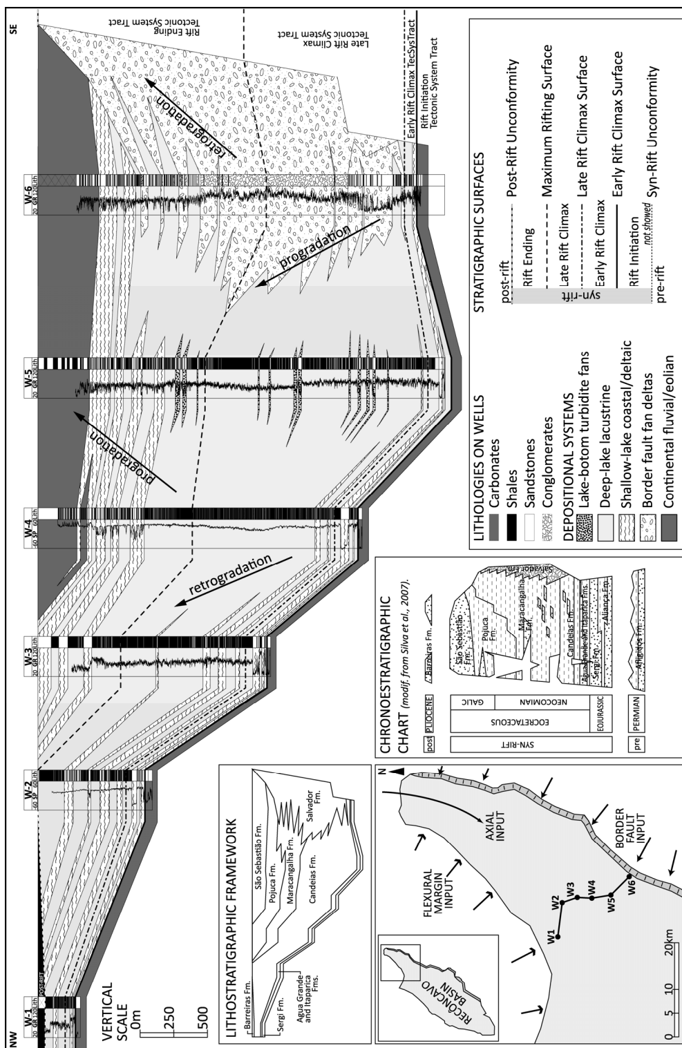
Figura 37: Seção estratigráfica com poços na porção norte da Bacia do Recôncavo, de orientação dip, mostrando os tratos de sistemas tectônicos mapeados e os padrões de empilhamento reconhecidos com base no arranjo dos sistemas deposicionais. Os poços W1 a W5 apresentam o padrão de empilhamento da margem flexural e o poço W6 tem o padrão de empilhamento da falha de borda. Extraído do Artigo 1.
