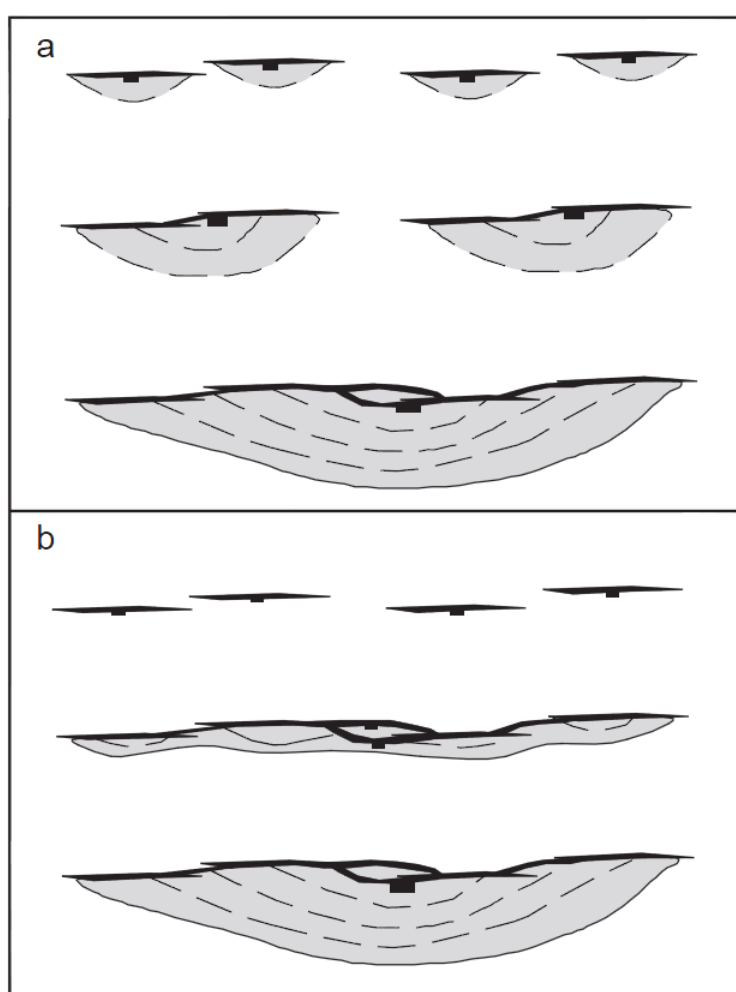
Figura 32: Ilustração esquemática do modelo de propagação de falha ( fault propagation ) de Morley (2002), com (a) ligação progressiva de falhas laterais durante um longo período evolutivo, onde se desenvolve uma ampla área deposicional no meio-gráben; (b) ligação progressiva de curta duração e sistemas de falhamentos laterais, desenvolvendo uma falha de borda. Inicialmente, a extensão deposicional do meio-gráben não é grande, e somente se desenvolve com a estabilidade da propagação e altos rejeitos verticais.
