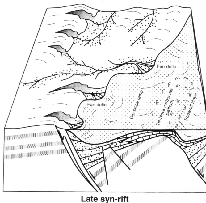
Figura 19: Modelo tectono-sedimentar do estágio sin-rifte final, conforme Bosence (1998), onde a atividade tectônica diminuiu, a drenagem se estabiliza e o aporte domina, com erosão das escarpas e entrada de sedimentos nos meio-grábens.
