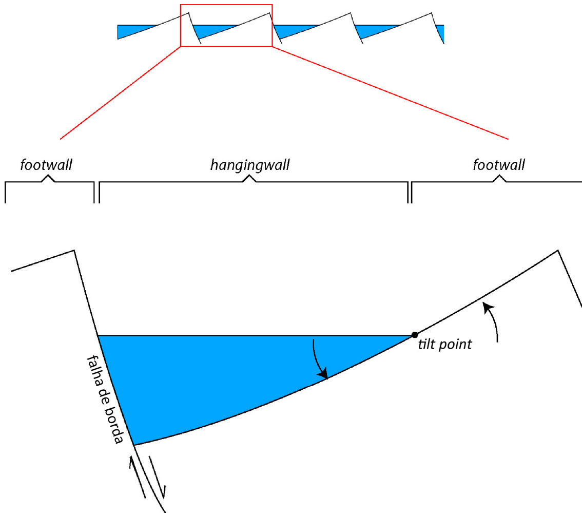
Figura 9: Modelo adaptado para o presente estudo, do sistema de meio-gráben com seus principais elementos e compartimentações. Devido à recorrência adjacente dos sistemas de meio-grábens, denomina-se hangingwall toda a região a qual sofre subsidência, enquanto que a região que sofre soerguimento é denominada footwal . O ponto que regula a ocorrência de footwal ou hangingwall é denominado tilt point . Extraído de Kuchle (2004).
