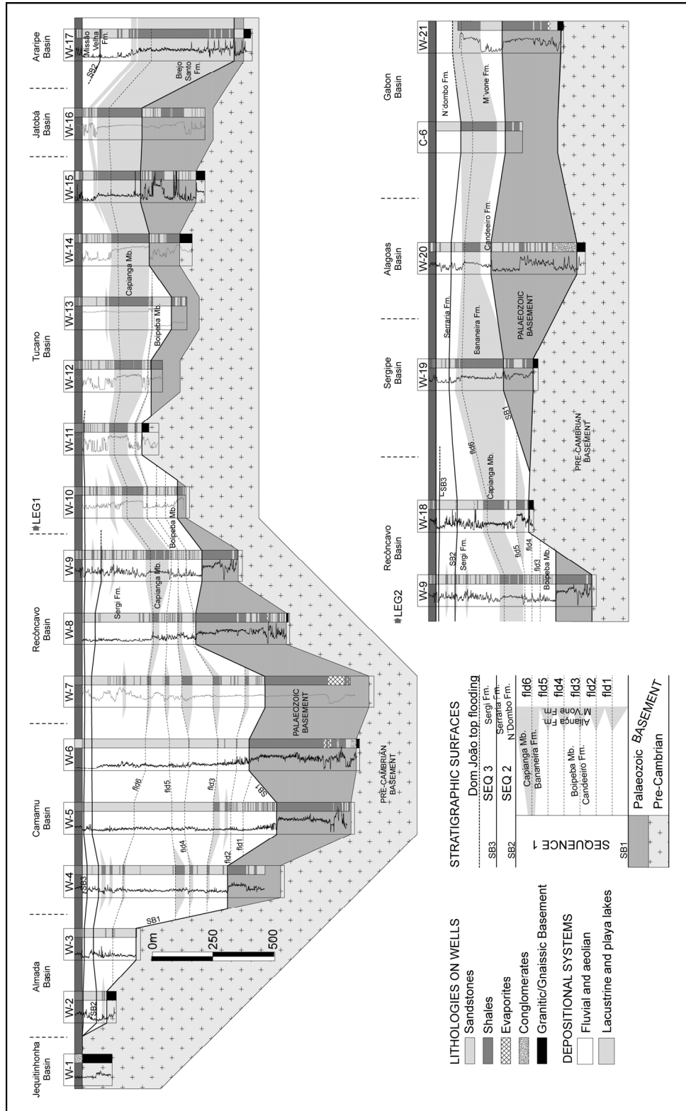
Figura 39: Seção de correlação estratigráfica regional compreendendo as bacias estudadas. O datum é a superfície de inundação no topo do Andar Dom João. Extraído do Artigo 3.
