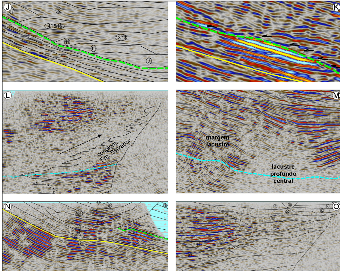
Figura 6: Quadros de detalhe da composição sísmica mostrando feições específicas dos padrões de refletores, terminações, estruturação interna e externa das unidades sismoestratigráficas, tratos de sistemas tectônicos e superfícies limítrofes, conforme descrito no texto.
