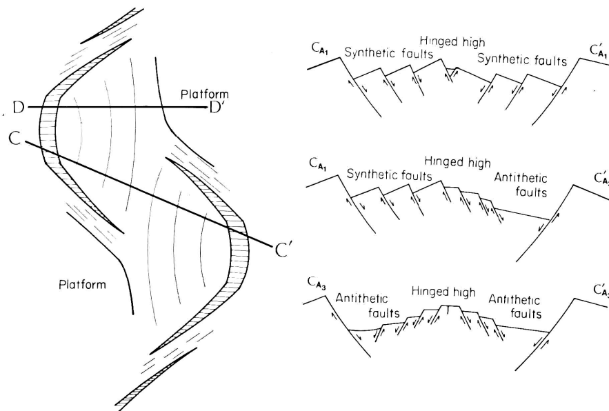
Figura 13: Outras possíveis morfologias geradas por disposições inversas de meio-grábens, gerando sistemas de horst-grabens , altos estruturais internos associados a margens flexurais conectadas e inversões na direção de falhamentos no interior da bacia. Extraído de Rosendahl et al. (1986).
