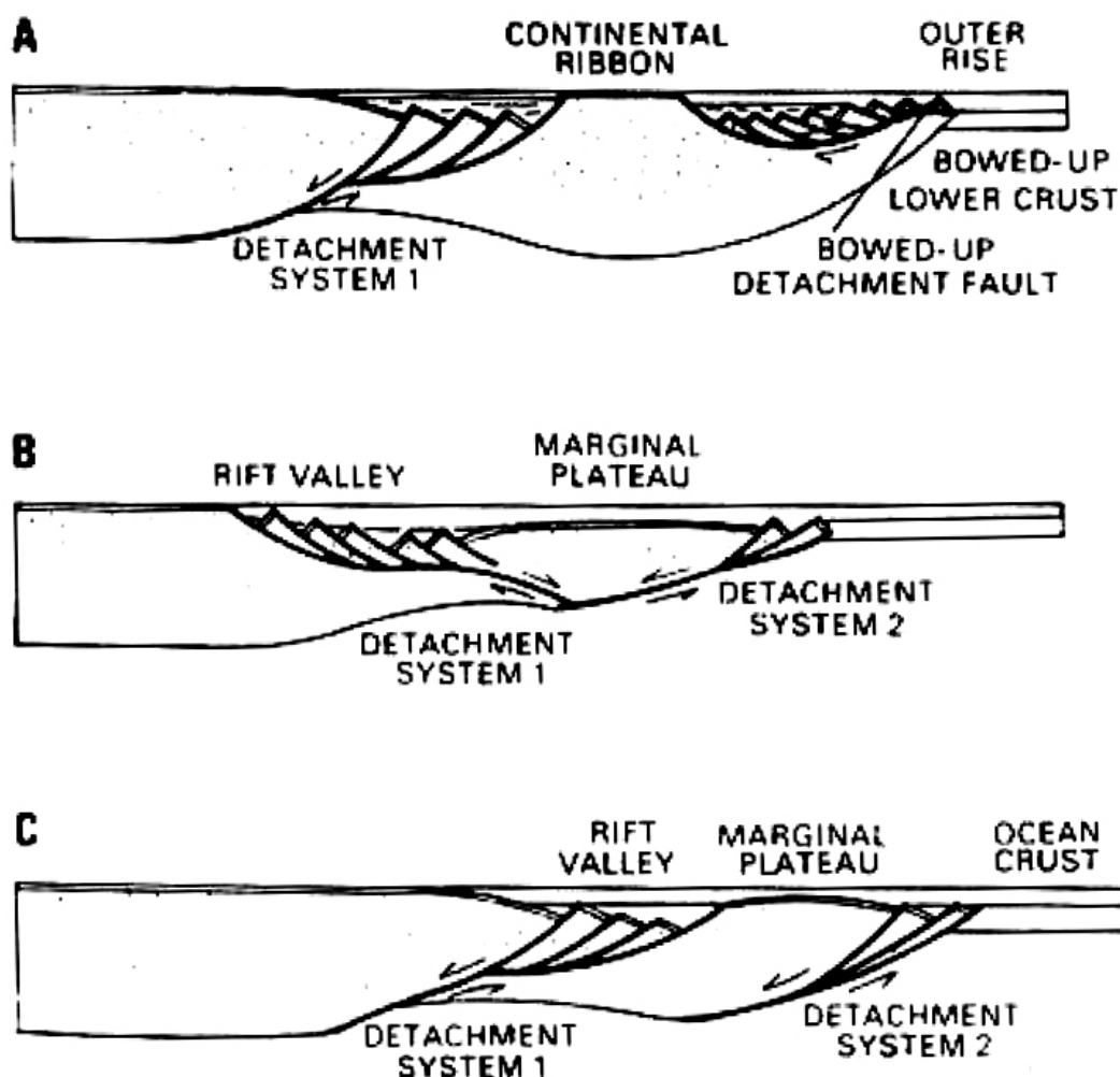
Figura 6: Modelo de múltiplos descolamentos de Lister (1986) baseado no modelo inicial de Wernicke (1985), com uma complexidade avançada do sistema de descolamento e desenvolvimento de meio-grábens adjacentes.
