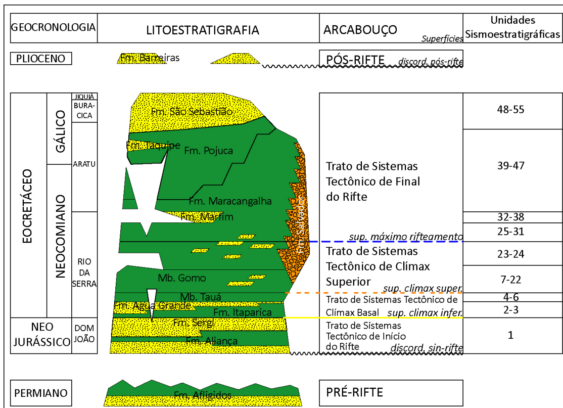
Figura 8: Carta cronoestratigráfica geral da Bacia do Recôncavo (modificado de Silva et al. , 2007) com o arcabouço de tratos de sistemas tectônicos proposto e as unidades sismoestratigráficas componentes dos tratos.
