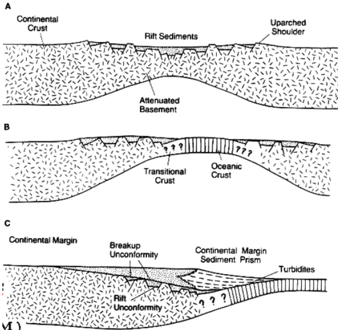
Figura 4: Modelo de rompimento crustal conforme o modelo de estiramento de Mackenzie (1978), extraído de Davis (1984). Como o estiramento é uniforme, a ruptura é simétrica e central, gerando duas bacias espelhadas.
