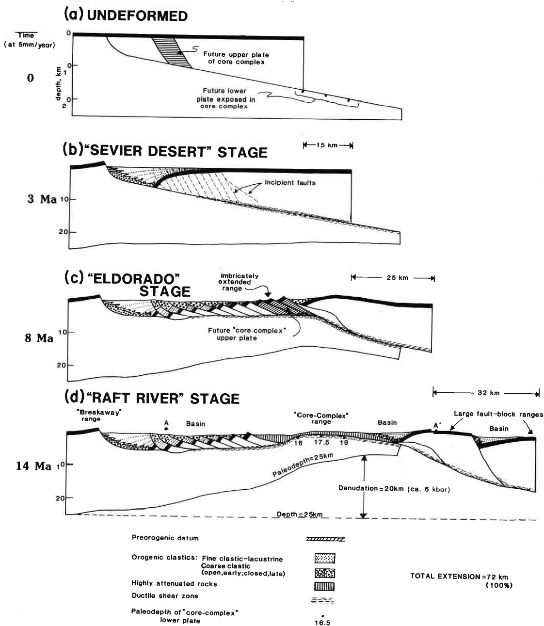
Figura 5: O modelo de Wernicke (1985) propõe um processo de deslizamento sob uma zona de cisalhamento de raiz subhorizontal. Assim, a evolução do rompimento crustal gera bacias diferentes em cada margem continental, tendo uma extensa seção sin-ripte na região à esquerda do modelo, e discretas seções sin-ripte à direita. Outro aspecto importante é que o rompimento não se dá exatamente abaixo do meio-gráben principal, pois neste modelo esta não é a zona de maior afinamento crustal – que no final do processo evolutivo, encontra-se lateralmente adjacente ao meio-gráben principal, com exposição dos complexos de núcleos metamórficos. É nesta zona que ocorrerá a abertura e geração dos primeiros SDR's ( seaward dipping reflectors ) e crostas oceânicas iniciais.
