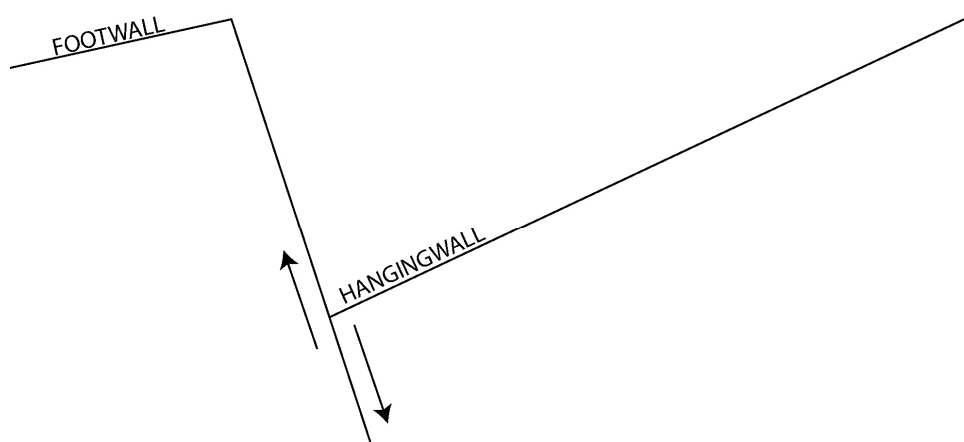
Figura 8: Compartimentação do meio-gráben - o footwal é o bloco ascendente em relação ao hangingwall como bloco descendente. Adaptado de Davis (1984).
