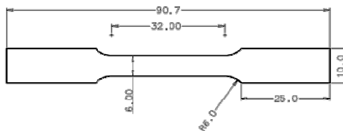
Figura 19. Corpo-de-Prova de tração
