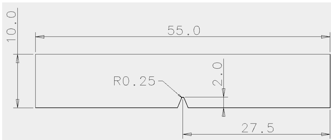
Figura 21. CDP para ensaio de impacto
