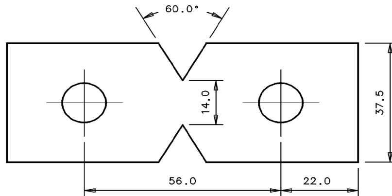
Figura 20. CDP para ensaio de tração com entalhe
