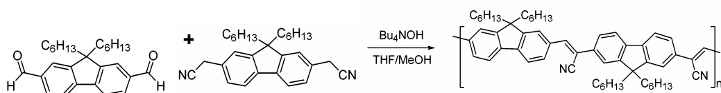
Figura 10: exemplos ilustrativos das reações de polimerização mais utilizadas na síntese de polímeros conjugados [26-30].
