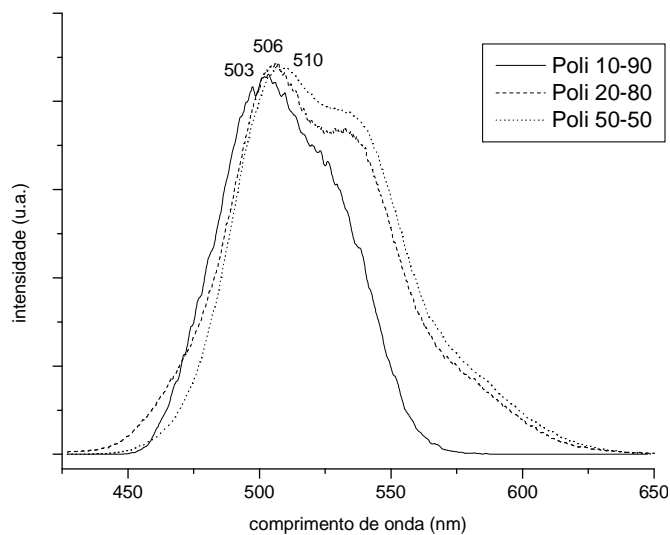
Figura 64: Espectros de fluorescência do filme do Poli 10-90, Poli 20-80, Poli 50-50. ( \lambda_{exc} = 400 \text{ nm} ): (a) não normalizada e (b) normalizada.
