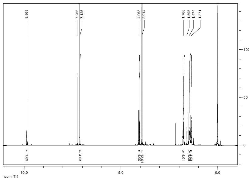
Figura 19: Espectro de RMN 1 H do DIAL.
