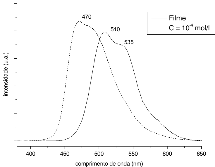
Figura 58: Espectros de fluorescência em filme e em solução
