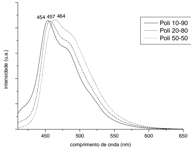
Figura 63: Espectros de fluorescência em solução ( C = 10^{-5} mol/L) do Poli 10-90, Poli 20-80, Poli 50-50. ( \lambda_{exc} = 400 nm): (a) não normalizada e (b) normalizada
