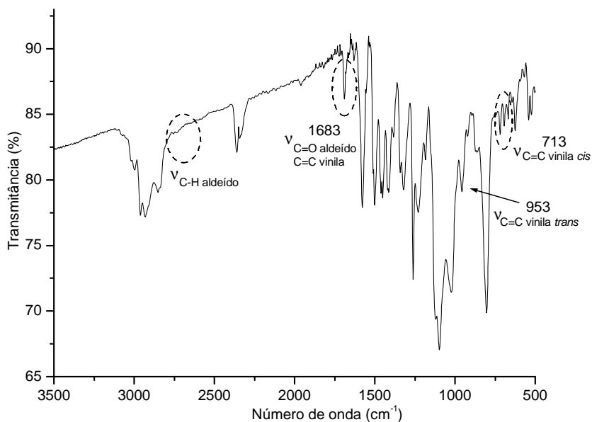
Figura 31: Espectro de FTIR do Poli 20-80.
