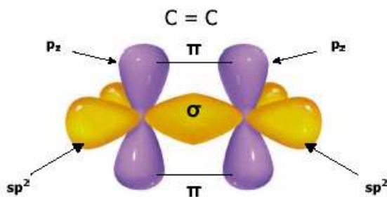
Figura 3: Representação dos orbitais moleculares \pi e \sigma formados entre dois átomos de carbono sp^2 [13].
