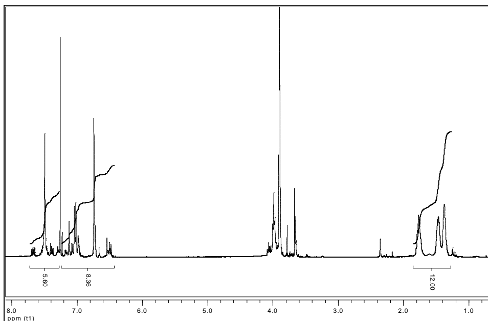
Figura 39: Espectro de RMN ^1\text{H} integrado do Poli 10-90.
