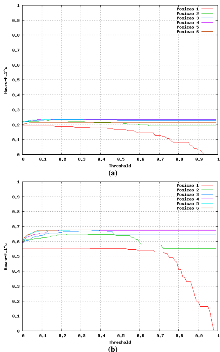
Figura 5-19 - Calibração de PBCut para VG-RAM WNN-COR e para (a) AT100 e (b) EX100.
