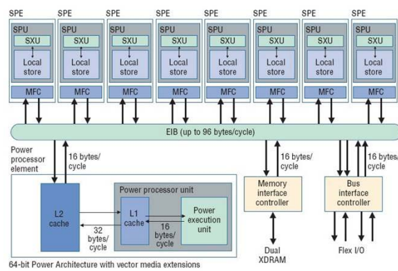
FIGURA 2.4. MPSOC CELL DESENVOLVIDO POR IBM, SONY E TOSHIBA PARA O PLAYSTATION 3 [KIS06].
