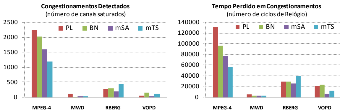
FIGURA 6.8. NÍVEL DE CONGESTIONAMENTOS NA NOC PARA OS ALGORITMOS INVESTIGADOS.
