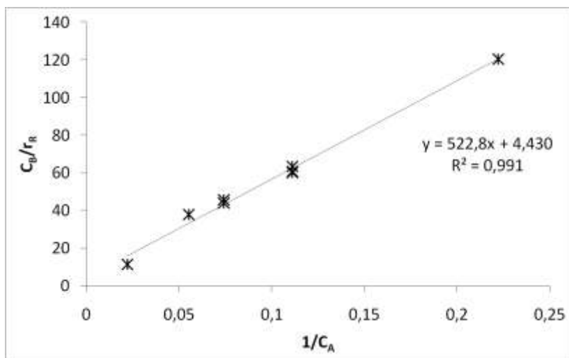
Figura 7-1: Ajuste do modelo de Langmuir-Hinshelwood aos dados experimentais de fotoredução catalítica de nitrato a \text{N}_2 em efluente solução aquosa utilizando \text{Zn-TiO}_2 como catalisador e \text{CHOOH} como seqüestrante de vacância. \text{CHOOH} = 450 \text{ mg L}^{-1} = 117,43 \text{ mg C L}^{-1} . \text{NO}_3^- = 4,5, 9,0, 13,5, 18,1 \text{ e } 45,2 \text{ mg N L}^{-1} . \text{Zn-TiO}_2 = 1 \text{ g L}^{-1} .
