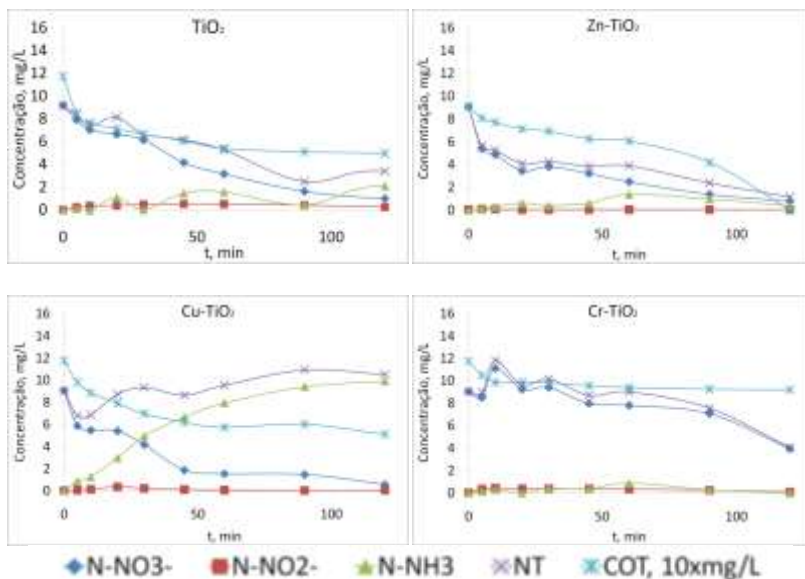
Figura 6-4: Cinética de fotodegradação de nitrato e COT, e formação de amônia e nitrito. pH \sim 2,5. \text{TiO}_2 , \text{Zn-TiO}_2 , \text{Cr-TiO}_2 e \text{Cu-TiO}_2 = 1 \text{ g L}^{-1} . \text{NO}_3^- = \sim 0,6 \text{ mM} ou 9,0 \text{ mg N L}^{-1} . \text{CHOOH} = \sim 9,8 \text{ mM} ou 117,4 \text{ mg COT L}^{-1} . Volume total 2,7 \text{ L} .
