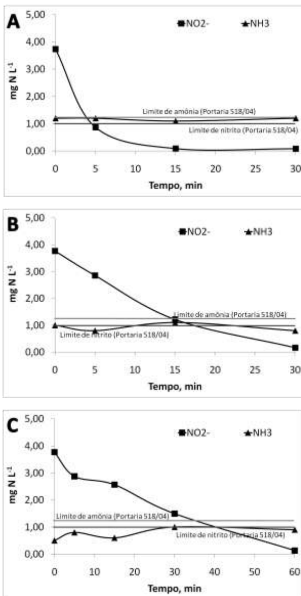
Figura 7-3: Comportamento de nitrito e amônia durante a redução fotocatalítica de nitrato em efluente real. Razão molar \text{CHOOH}:\text{nitrato} = (A) 2,7, (B) 1,6 e (C) 1,0, respectivamente para [\text{HCOOH}] = 1636, 1000 e 500 \text{ mg L}^{-1} ou 427, 261 e 130 \text{ mg C L}^{-1} . Catalisador \text{Zn-TiO}_2 = 1 \text{ g L}^{-1} .
