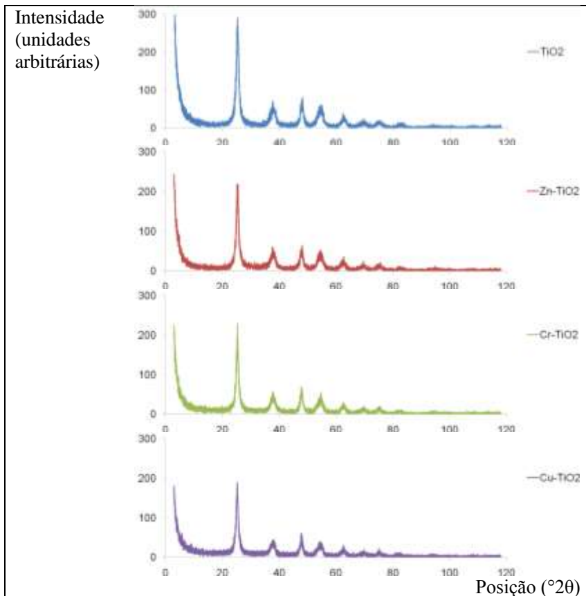
Figura 6-2: Difractogramas de raios X dos catalisadores
