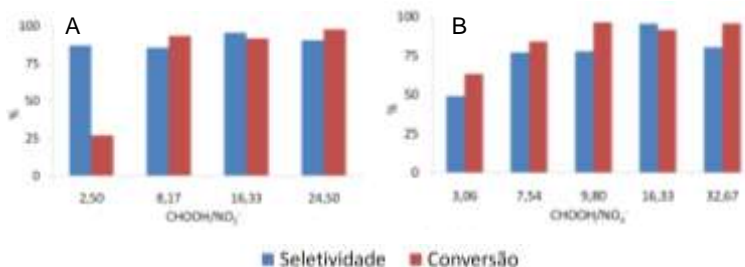
Figura 6-5: Avaliação do efeito da variação da concentração de (A) CHOOH mantido \text{NO}_3^- = 0,6 mM e (B) \text{NO}_3^- mantido CHOOH = 9,8 mM. \text{CHOOH}/\text{NO}_3^- : mM/mM.
