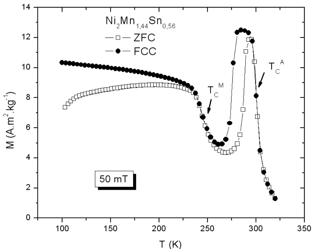
Figura 4.13 - Magnetização em função da temperatura para a amostra Ni_2Mn_{1,44}Sn_{0,56} , em um campo magnético de 50 mT.
