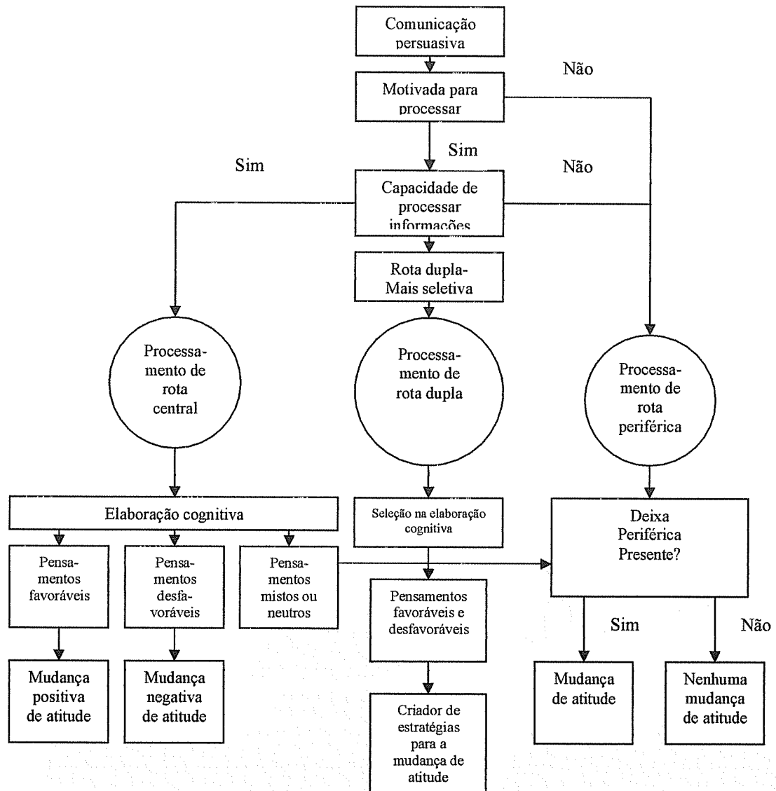
Figura 2 – Modelo intermitente para a probabilidade de elaboração
