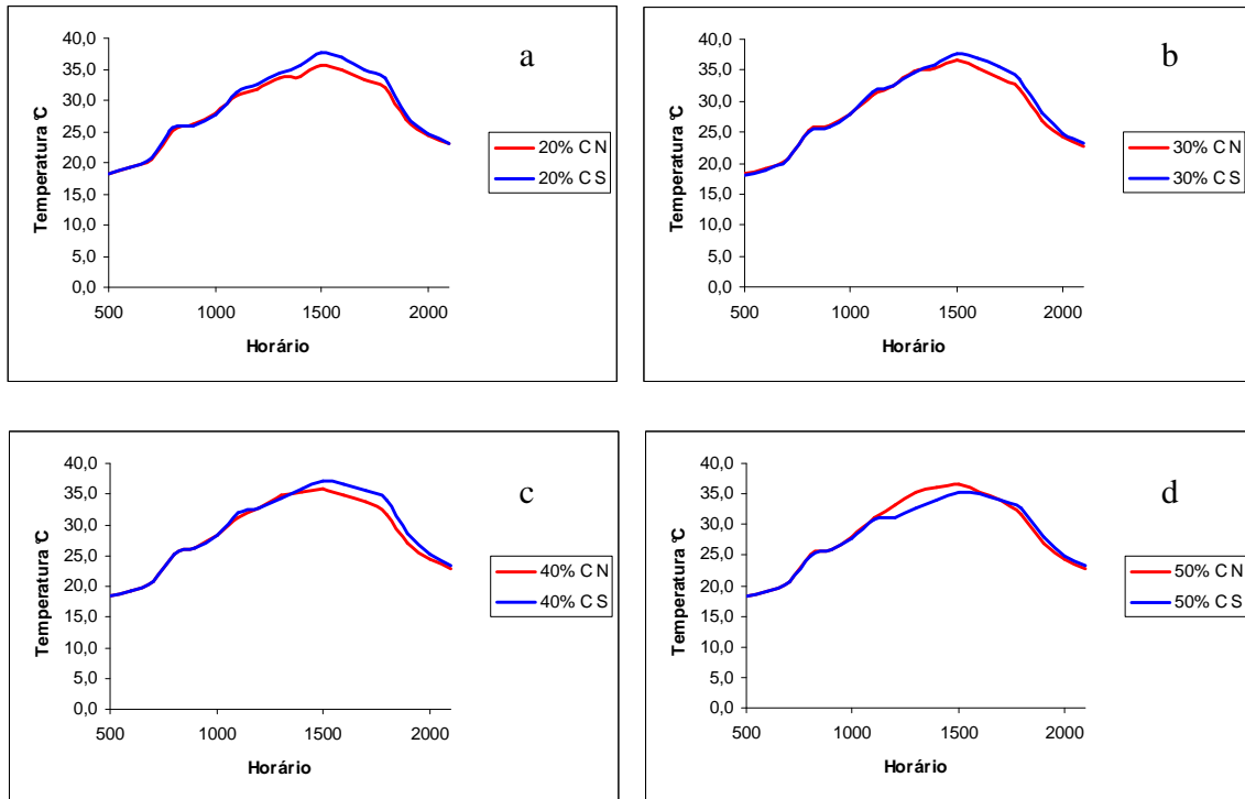
Figura 9. Variação de temperatura ao longo do dia crítico de verão nas exposições Norte e Sul com cobertura de cerâmica. Figura “a” representa a inclinação de 20%, a figura “b” 30%, a figura “c” 40% e a figura “d” 50% de inclinação
