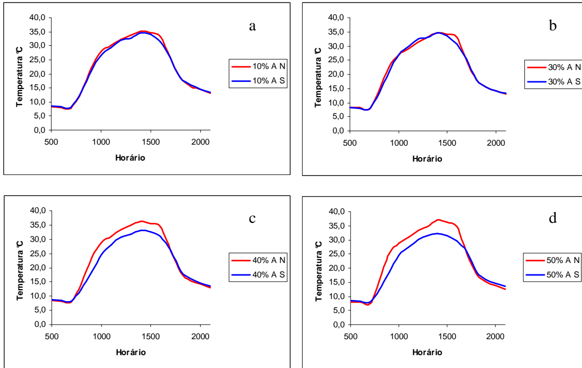
Figura 8. Variação de temperatura ao longo do dia crítico de inverno nas exposições Norte e Sul com cobertura de aço galvanizado. Figura “a” representa a inclinação de 10%, a figura “b” 30%, a figura “c” 40% e a figura “d” 50% de inclinação
