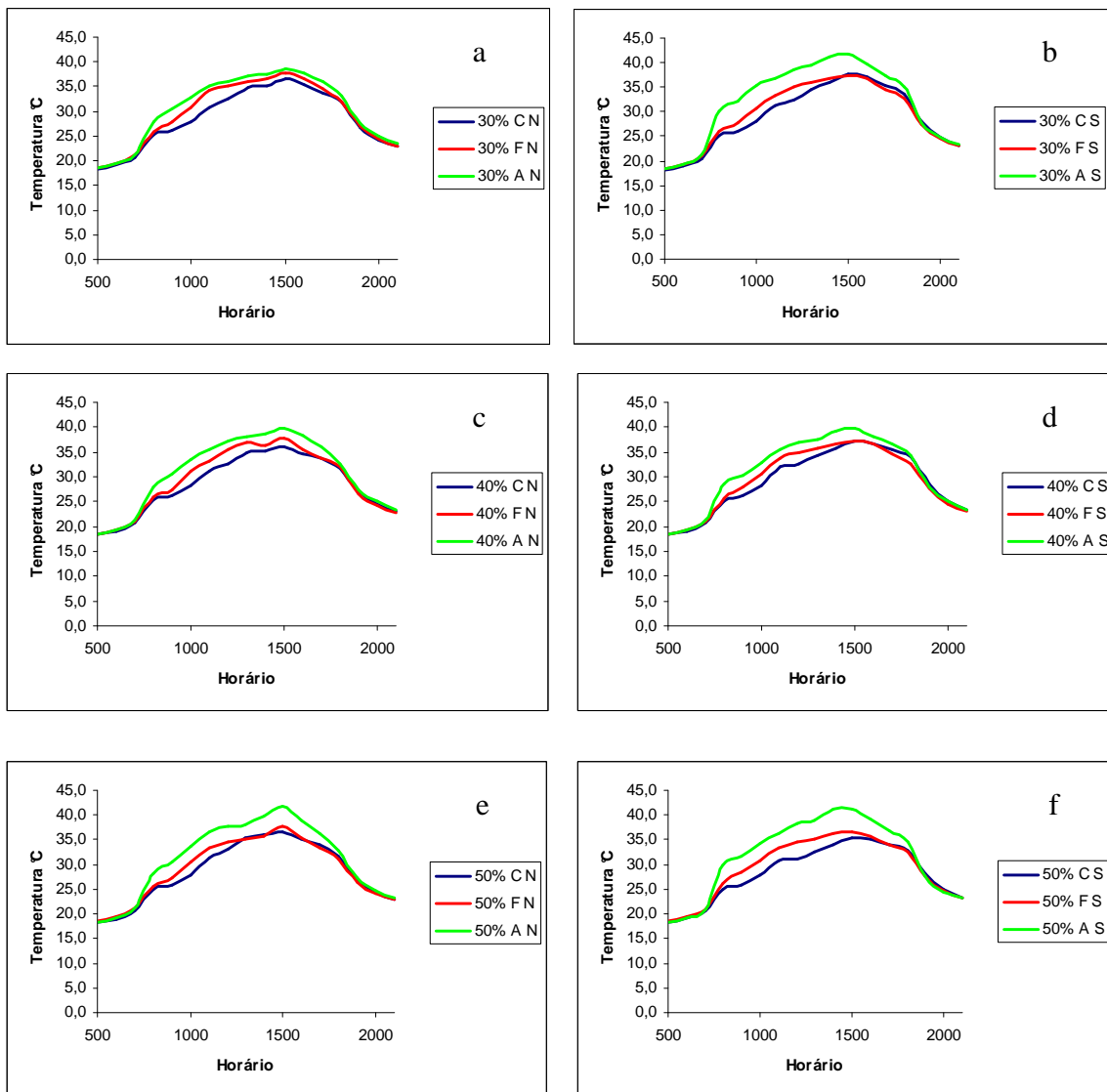
Figura 13. Variação de temperatura ao longo do dia crítico de verão nas diferentes coberturas. Figura “a” representa a inclinação de 30% na exposição Norte, a figura “b” 30% na exposição Sul, a figura “c” 40% na exposição Norte, a figura “d” 40% na exposição Sul, a figura “e” 50% na exposição Norte, e a figura “f” 50% na exposição Sul.
