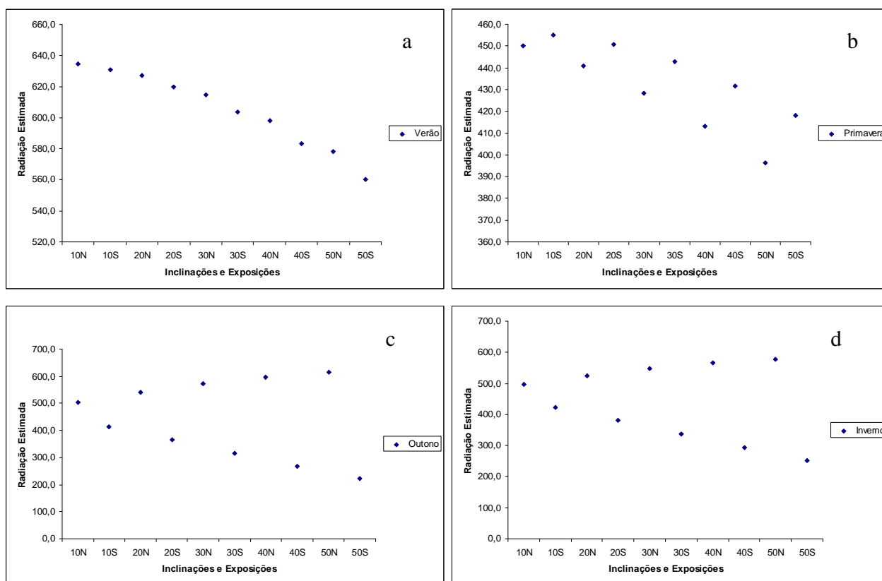
Figura 5. Radiação Solar Global Estimada nas inclinações de 10,20,30,40 e 50% nas exposições Norte e Sul. Figura “a” representa a estação verão, figura “b” a estação primavera, a figura “c” a estação outono e a figura “d” a estação inverno.
