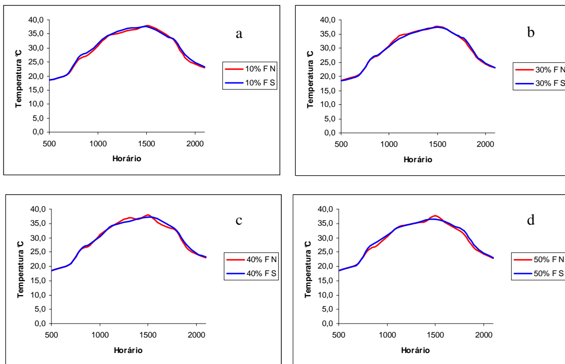
Figura 10. Variação de temperatura ao longo do dia crítico de verão nas exposições Norte e Sul com cobertura de fibrocimento. Figura “a” representa a inclinação de 10%, a figura “b” 30%, a figura “c” 40% e a figura “d” 50% de inclinação
