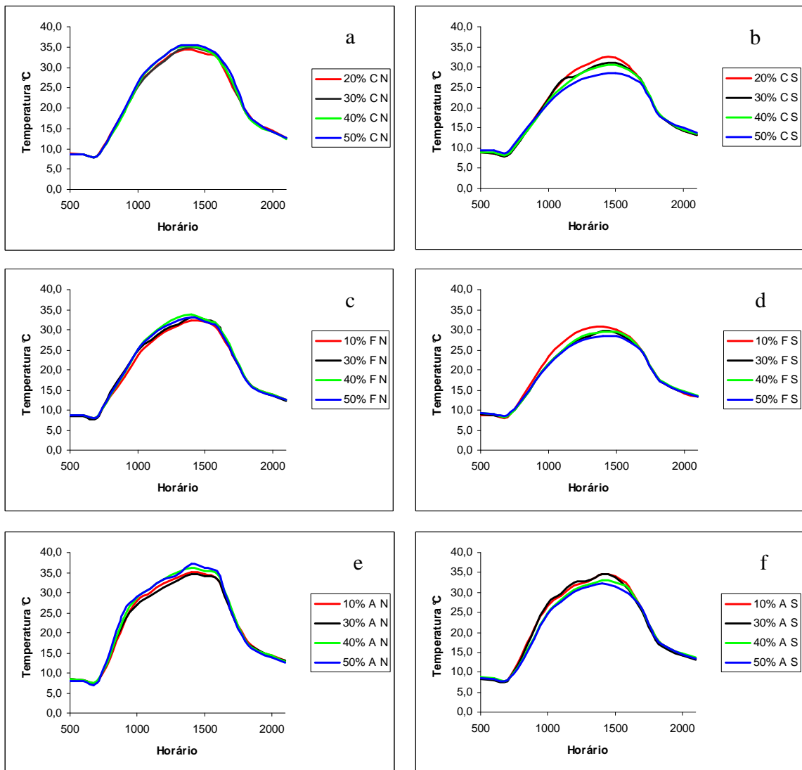
Figura 14. Variação de temperatura ao longo do dia crítico de inverno nas inclinações de 20,30,40 e 50% com cobertura de cerâmica e 10,30,40 e 50% com cobertura de fibrocimento e aço galvanizado. Figura “a” representa a cobertura de cerâmica na exposição Norte, a figura “b” cobertura de cerâmica na exposição Sul, a figura “c” cobertura de fibrocimento na exposição Norte, a figura “d” cobertura de fibrocimento na exposição Sul, a figura “e” cobertura de aço galvanizado na exposição Norte, e a figura “f” cobertura de aço galvanizado na exposição Sul.
