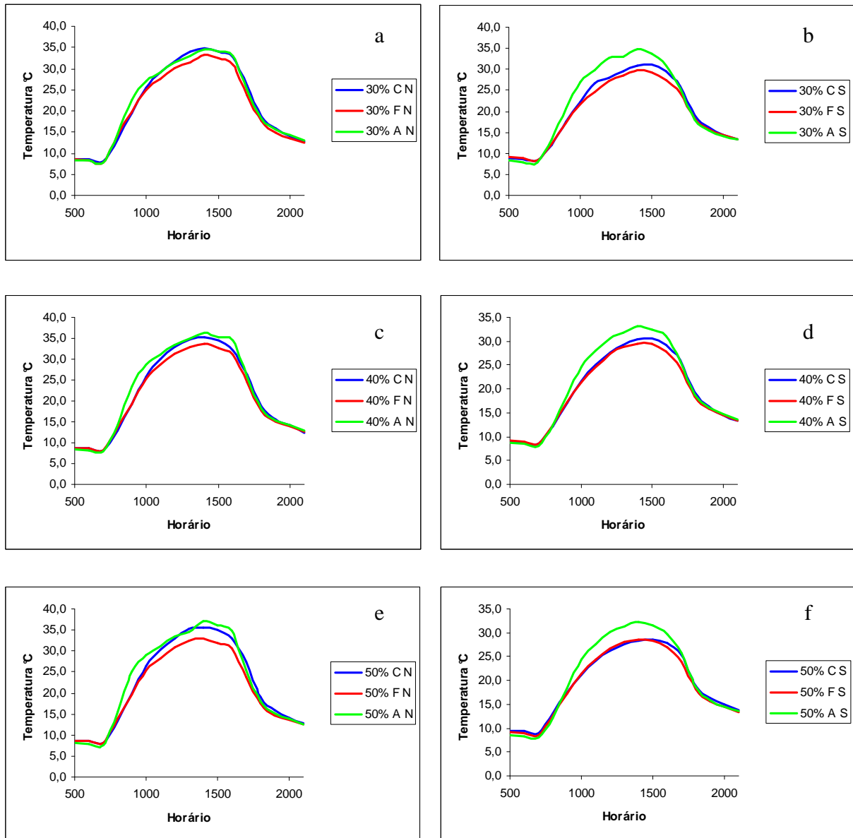
Figura 12. Variação de temperatura ao longo do dia crítico de inverno nas diferentes coberturas. Figura “a” representa a inclinação de 30% na exposição Norte, a figura “b” 30% na exposição Sul, a figura “c” 40% na exposição Norte, a figura “d” 40% na exposição Sul, a figura “e” 50% na exposição Norte, e a figura “f” 50% na exposição Sul.
