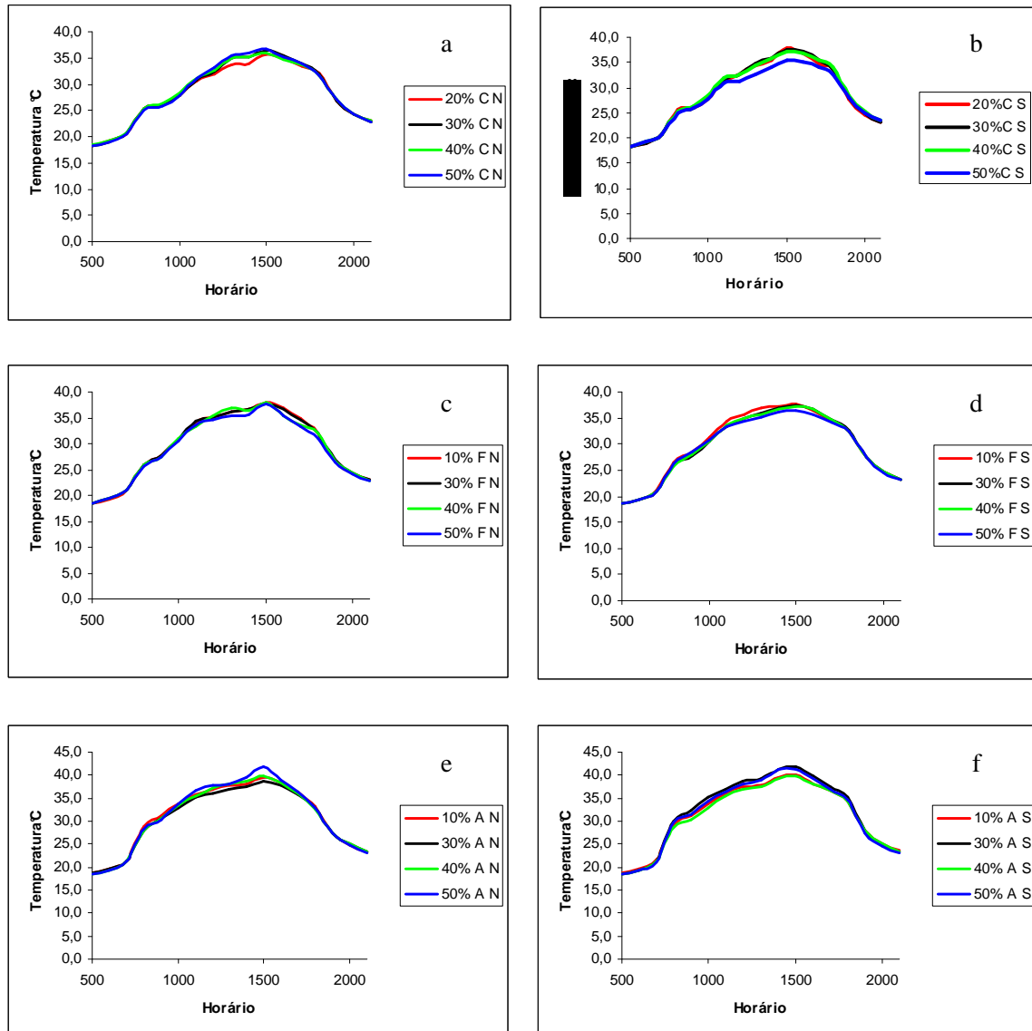
Figura 15. Variação de temperatura ao longo do dia crítico de verão nas inclinações de 20,30,40 e 50% com cobertura de cerâmica e 10,30,40 e 50% com cobertura de fibrocimento e aço galvanizado. Figura “a” representa a cobertura de cerâmica na exposição Norte, a figura “b” cobertura de cerâmica na exposição Sul, a figura “c” cobertura de fibrocimento na exposição Norte, a figura “d” cobertura de fibrocimento na exposição Sul, a figura “e” cobertura de aço galvanizado na exposição Norte, e a figura “f” cobertura de aço galvanizado na exposição Sul.
