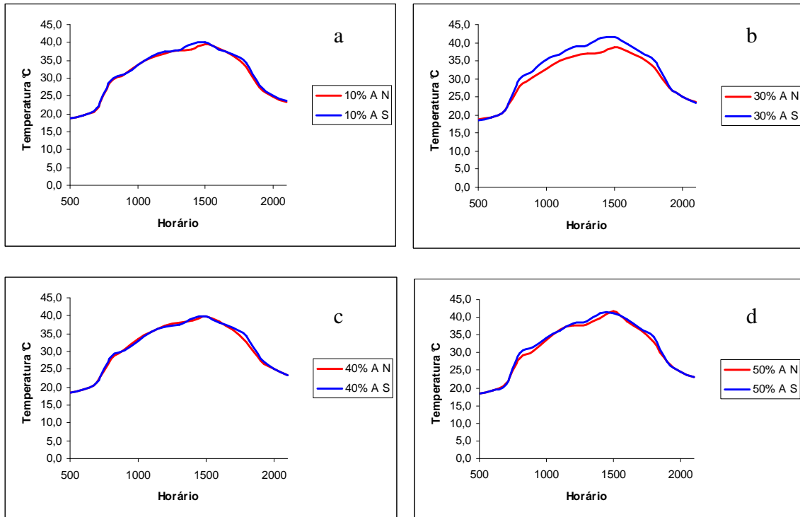
Figura 11. Variação de temperatura ao longo do dia crítico de verão nas exposições Norte e Sul com cobertura de aço galvanizado. Figura “a” representa a inclinação de 10%, a figura “b” 30%, a figura “c” 40% e a figura “d” 50% de inclinação
