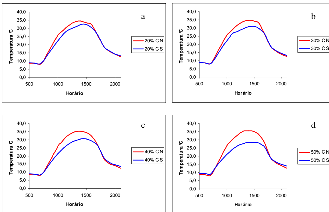
Figura 6. Variação de temperatura ao longo do dia crítico de inverno nas exposições Norte e Sul com cobertura de cerâmica. Figura “a” representa a inclinação de 20%, a figura “b” 30%, a figura “c” 40% e a figura “d” 50% de inclinação.
