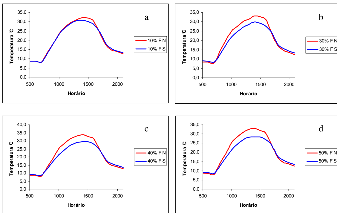
Figura 7. Variação de temperatura ao longo do dia crítico de inverno nas exposições Norte e Sul com cobertura de fibrocimento. Figura “a” representa a inclinação de 10%, a figura “b” 30%, a figura “c” 40% e a figura “d” 50% de inclinação
