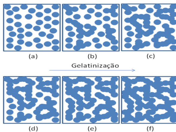
Figura 30. Evolução da gelificação com o aumento de fração de microgel [90] .
