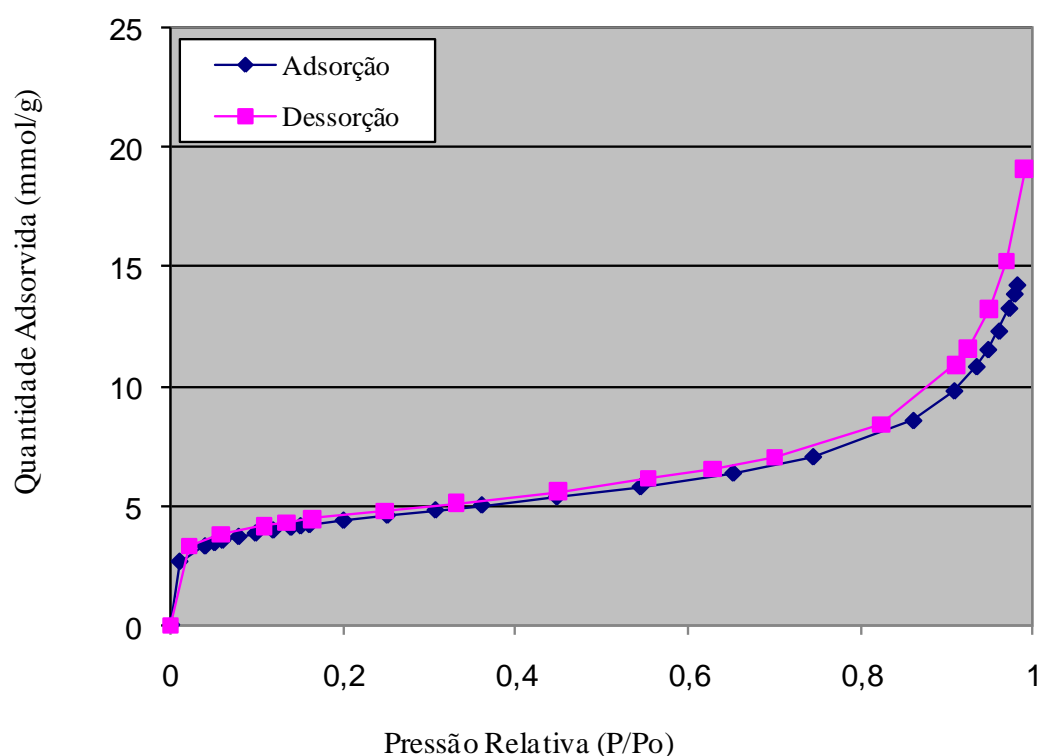
Figura 53. Isothermas de Adsorção e Dessorção de nitrogênio do xerogel híbrido \beta -diimina/sílica, contendo o ligante L_1 2-(fenil)amino-4-(fenil)imino-2-penteno) ( MH_4 ).
