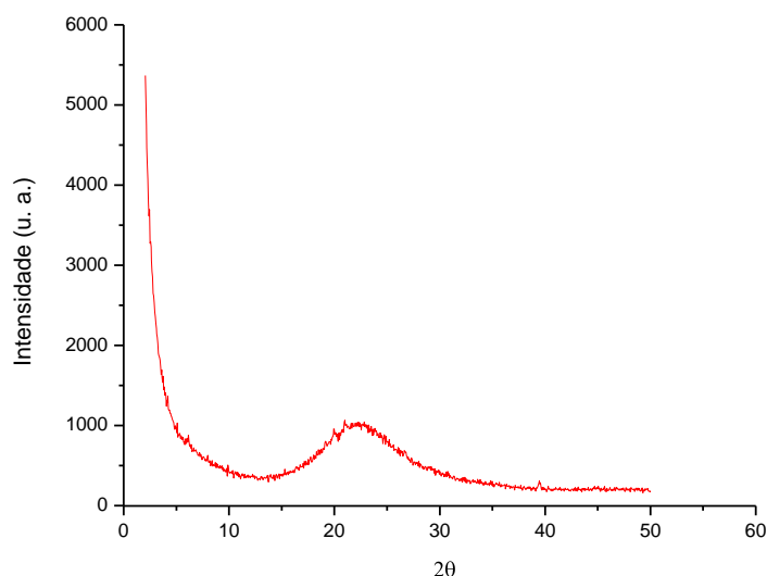
Figura 54. Difratograma do xerogel híbrido \beta -diimina/sílica, contendo o ligante L 1 2-(fenil)amino-4-(fenil)imino-2-penteno) (MH 4 ).
