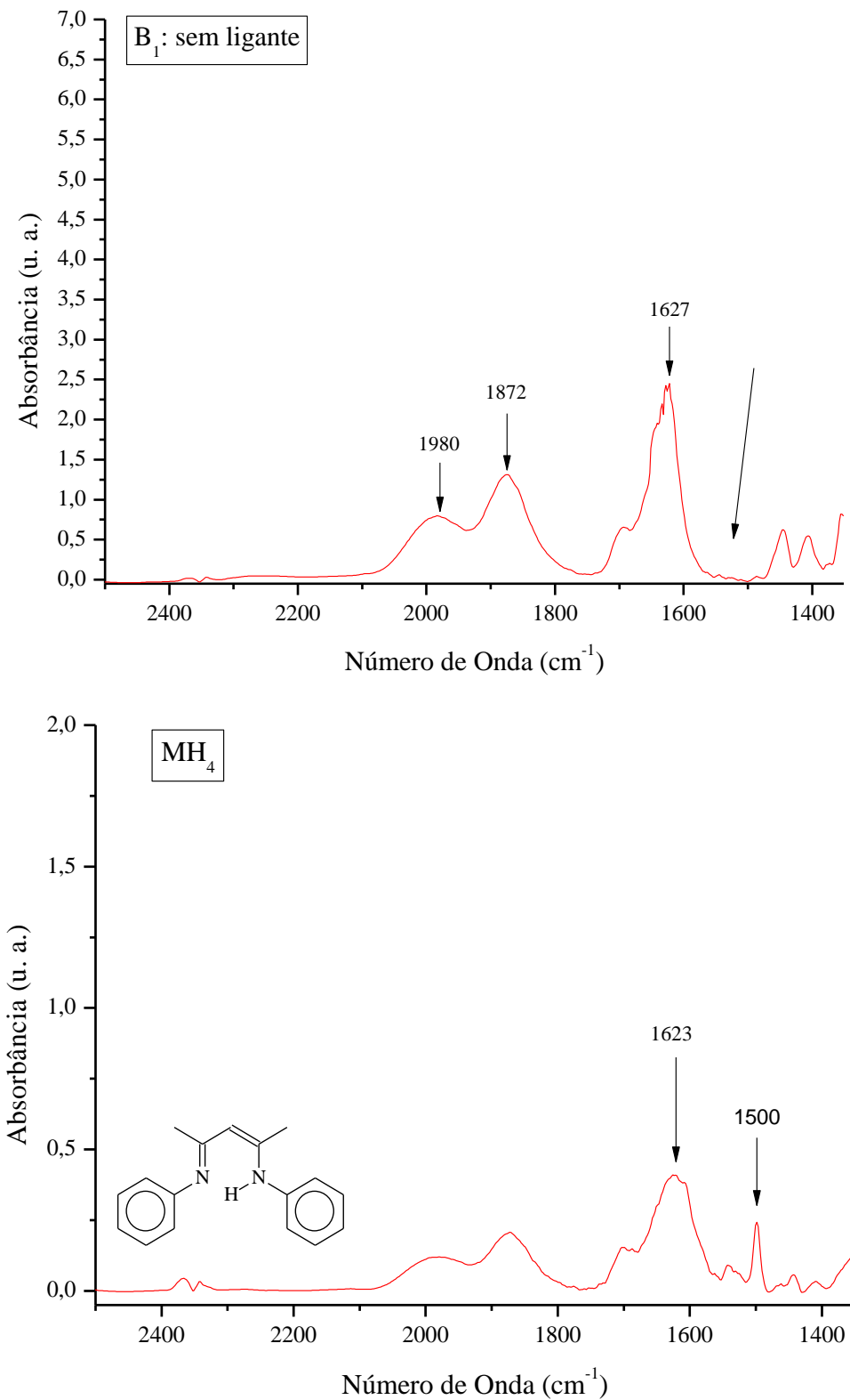
Figura 50. Espectro vibracional de infravermelho de uma amostra sem incorporação de ligante, B_1 , e do xerogel híbrido \beta -diimina/sílica, contendo o ligante L_1 2-(fenil)amino-4-(fenil)imino-2-penteno) ( MH_4 ).
