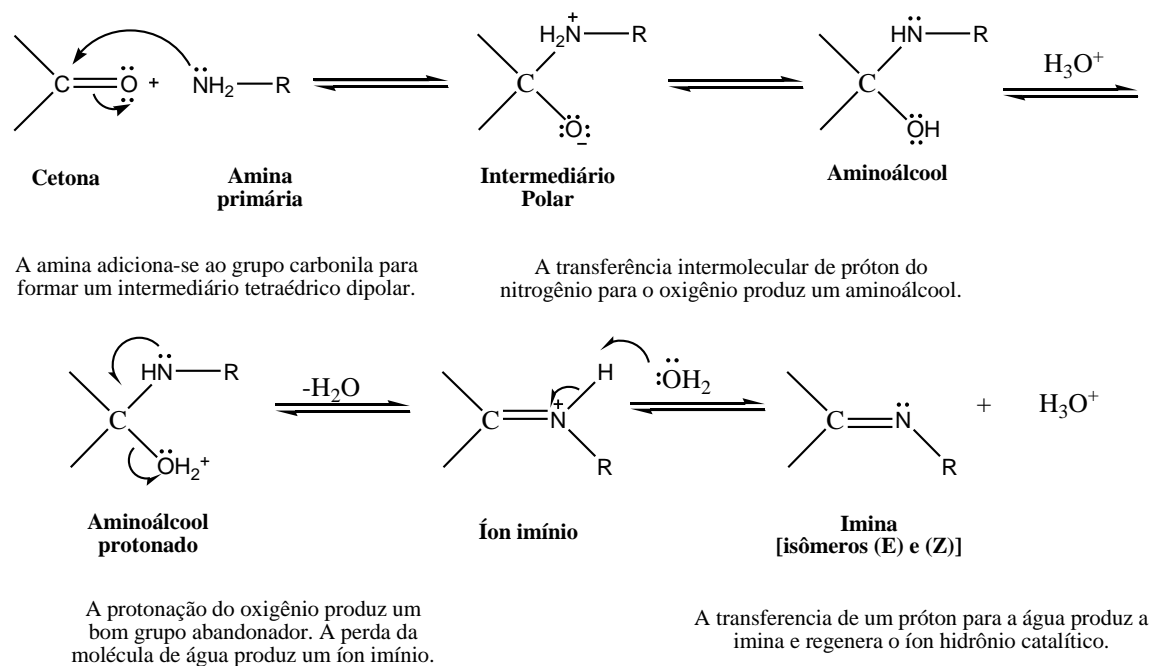
Figura 44. Mecanismo de formação de uma imina. [108]
