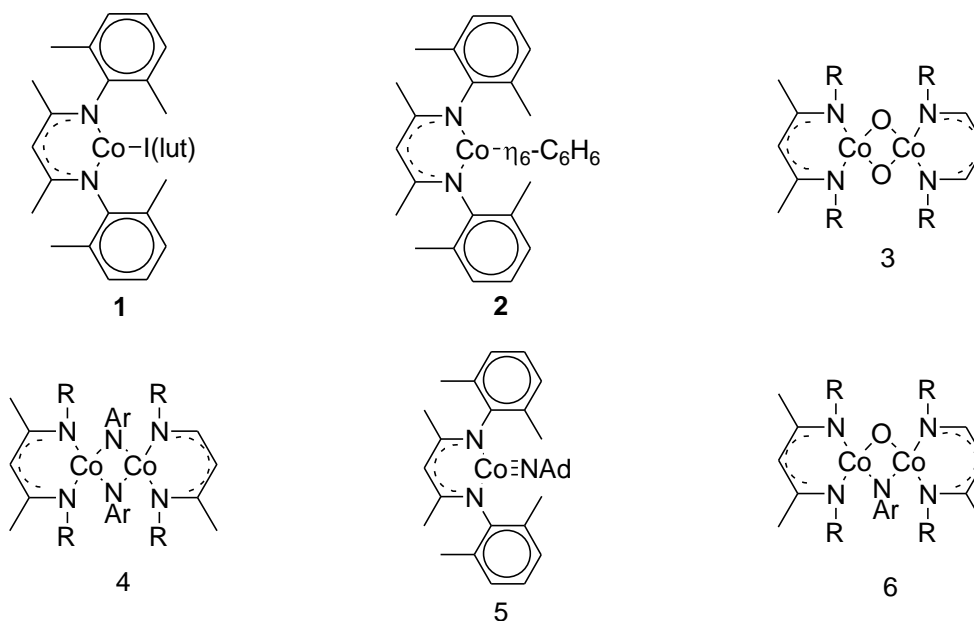
Figura 6. Estrutura molecular dos complexos de cobalto sintetizados por Dai, Kapoor e Warren. Estruturas 3, 4 e 6 R = 2,6-dimetilfenil. Estrutura 5, Ad = 1-adamantil.
