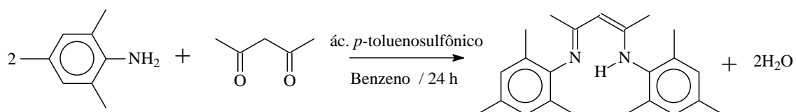
Figura 33. Rota de síntese do ligante 2-(2,4,6-trimetilfenil)amino-4-(2,4,6-trimetilfenil)imino-2-penteno.
