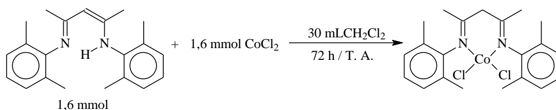
Figura 36. Rota de síntese para o complexo dicloro-1,5- bis (2,6-dimetilfenil)pentanodiiminacobalto(II).
