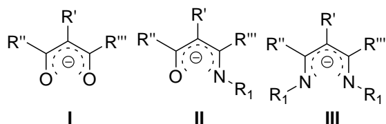
Figura 3. Ligantes \beta -dicetona (I) \beta -enaminocetona (II) e \beta -diimina (III).
