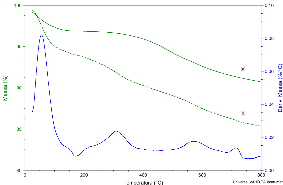
Figura 52. Termograma do (a) B 1 e (b) xerogel híbrido β-diimina/sílica, contendo o ligante L 1 2-(fenil)amino-4-(fenil)imino-2-penteno) (MH 4 ).
