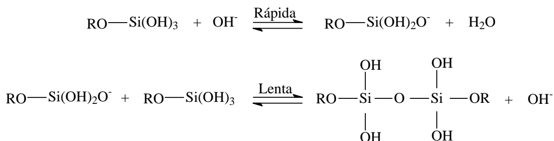
Figura 29. Mecanismo de condensação catalisada por base.
