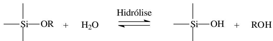
Figura 23. Reação de hidrólise.
