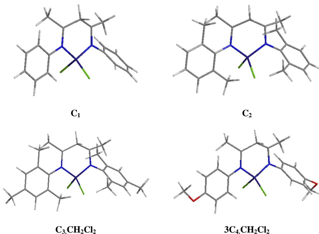
Figura 57. Modelo em 3D das estruturas propostas para os complexos C_1 [dicloro-1,5- bis (fenil)pentanodiiminacobalto(II)], C_2 [dicloro-1,5- bis (2,6-dimetilfenil)pentanodiiminacobalto(II)], C_3 [dicloro-1,5- bis (2,4,6-trimetilfenil)pentanodiimina e C_4 [dicloro-1,5- bis (4-metoxifenil)pentanodiiminacobalto(II)].
