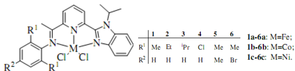
Figura 18. Complexos de Ni, Fe e Co contendo os ligantes imidazolil-piridil diferentemente substituídos.
