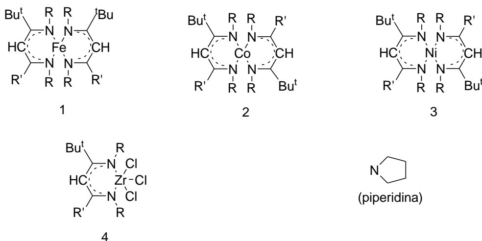
Figura 14. Estrutura molecular dos complexos de Fe ( 1 ), Co ( 2 ), Ni ( 3 ) e Zr ( 4 ) empregados nas reações de polimerização. Em todas as estruturas, \text{R} = \text{SiMe}_3 e \text{R}' = piperidina.
