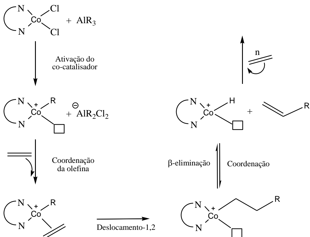
Figura 20. Mecanismo de oligomerização do eteno proposto para os complexos de Co- \beta -diimina, homogêneos e heterogeneizados.
