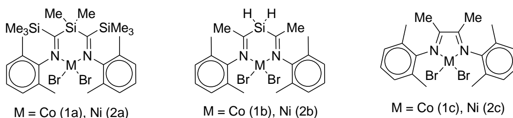
Figura 15. Estrutura molecular dos complexos de níquel e cobalto empregados nas reações de polimerização.
