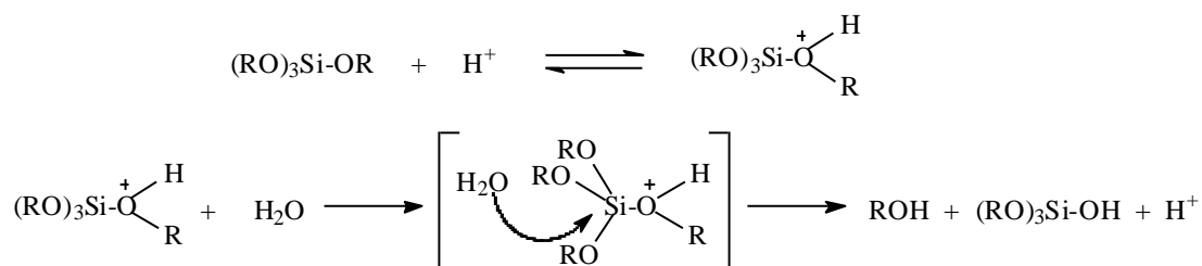
Figura 25. Mecanismo de hidrólise catalisada por ácidos.
