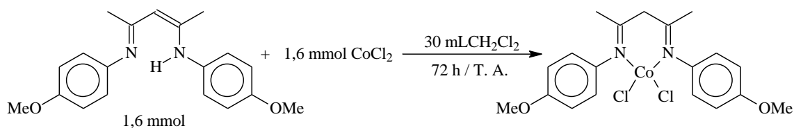
Figura 38. Rota de síntese para o complexo dicloro-1,5- bis (4-metoxifenil)pentanodiiminacobalto(II).
