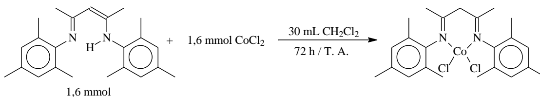
Figura 37. Rota de síntese para o complexo dicloro-1,5- bis (2,4,6-trimetilfenil)pentanodiiminacobalto(II).
