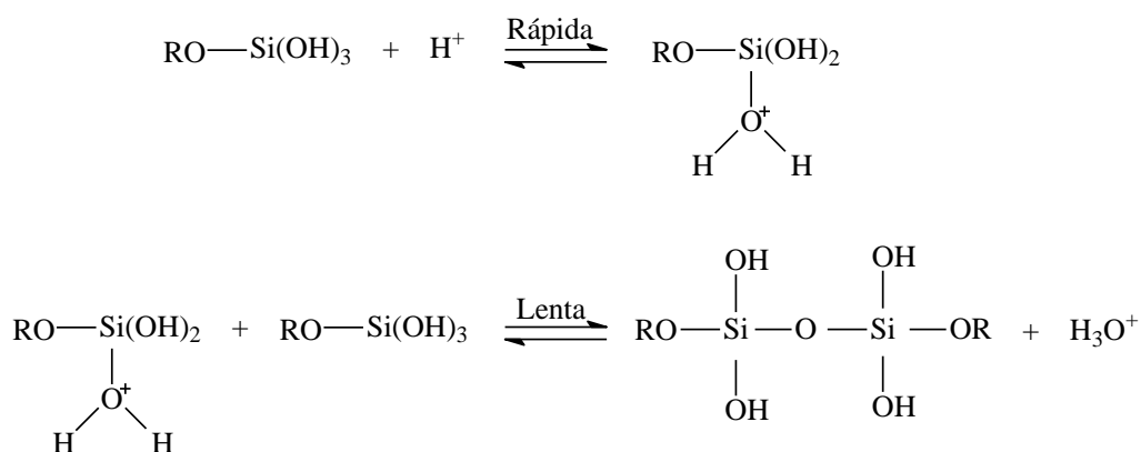
Figura 28. Mecanismo de condensação catalisada por ácido.
