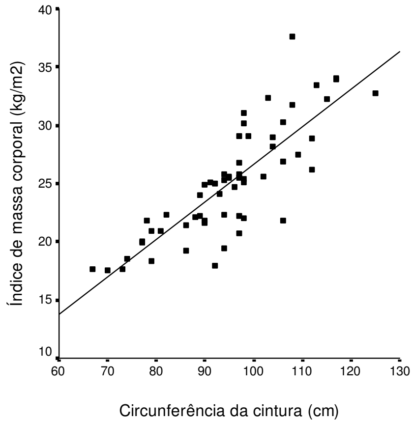
Figura 3: Scatter plot ilustrando a correlação bivariada entre índice de massa corporal e circunferência da cintura ( r=0,828 ; r^2=0,685 ; p<0,001 ).
