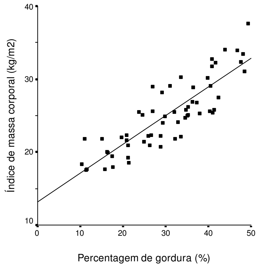
Figura 2: Scatter plot ilustrando a correlação bivariada entre porcentagem de gordura e índice de massa corporal ( r=0,859 ; r^2=0,738 ; p<0,001 ).
