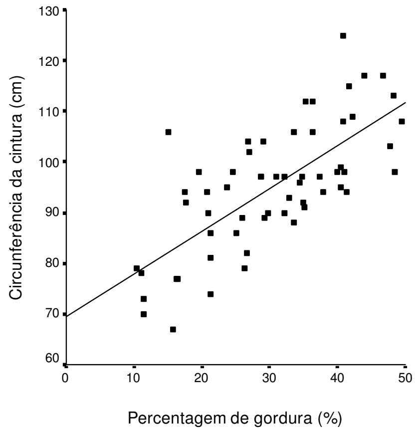
Figura 1: Scatter plot ilustrando a correlação bivariada entre porcentagem de gordura e circunferência da cintura ( r=0,716 ; r^2=0,513 ; p<0,001 ).
