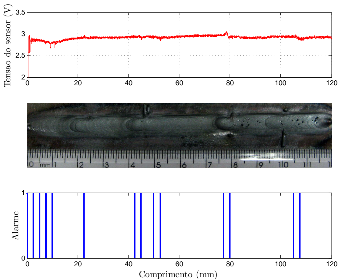
Figura 4.28. Resultado da detecção on-line de descontinuidades geradas por arame. stand-off = 5 mm e descontinuidades no par distância/quantidade-de-aramé: 25 mm/1, 45 mm/2, 80 mm/3 e 100 mm/1.
