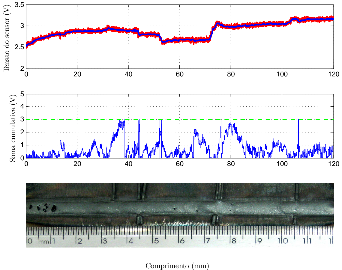
Figura 4.21. Resultado do ajuste para a detecção de descontinuidades por arame. stand-off = 3 mm e descontinuidades no par distância/quantidade-de-arame: 35 mm/1, 45 mm/2, 75 mm/3 e 105 mm/1.
