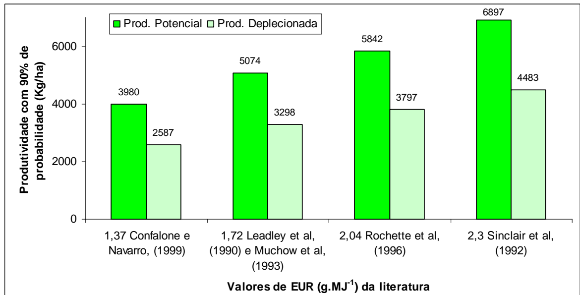
Figura 27 - Produtividades potencial e deplecionada resultantes do modelo PPDSO com diferentes valores de EUR ( \text{g.MJ}^{-1} ) encontrados na literatura e semeadura em primeiro de setembro para a localidade de Piracicaba (SP)
