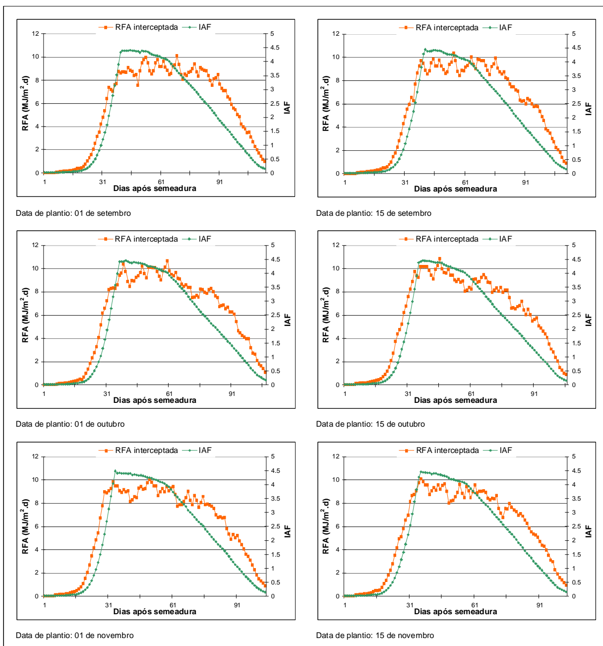
Figura 14 - Índice de área foliar (IAF, m^2.m^{-2} ) e radiação fotossinteticamente ativa interceptada (RFA, MJ.m^{-2}.dia^{-1} ) para a localidade de Piracicaba (SP) em semeaduras efetuadas em setembro, outubro e novembro
