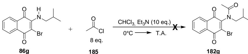
Esquema 72 - Tentativa de acetilação do composto 86a utilizando cloreto de acetila.
