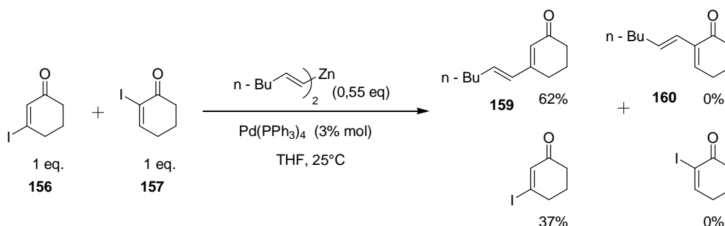
Esquema 54 – Regioseletividade no acoplamento de halogêneos em sistemas \alpha,\beta -insaturados. 63,69
