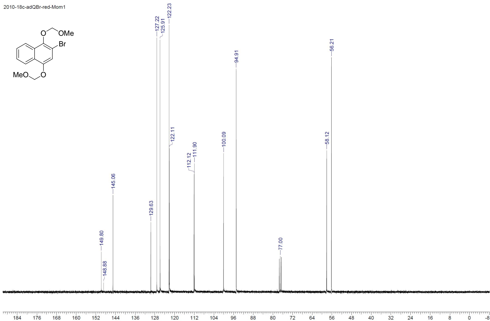
Espectro E – 18.3 - (RMN ^{13}\text{C} , 75 MHz, \text{CDCl}_3 ) – Composto reduzido 110a
