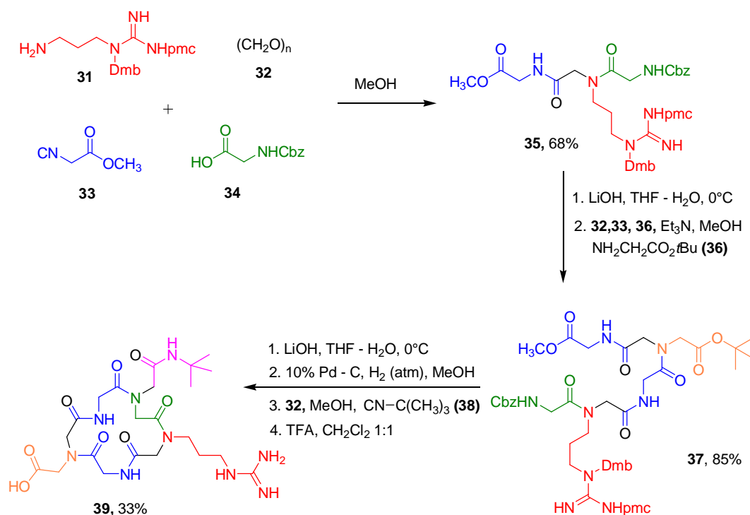
Esquema 6 – Síntese de peptídeos cíclicos e acíclicos via reação de Ugi. 16
