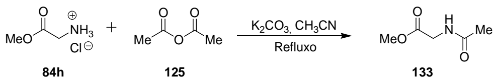
Esquema 73 - Síntese da amida 133 .
