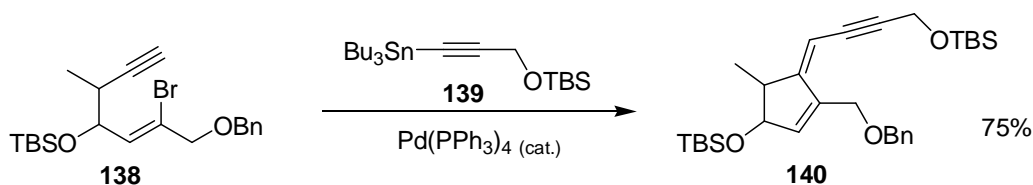
Esquema 46 - Ciclização e posterior alquilação do grupo acetileno. 61
