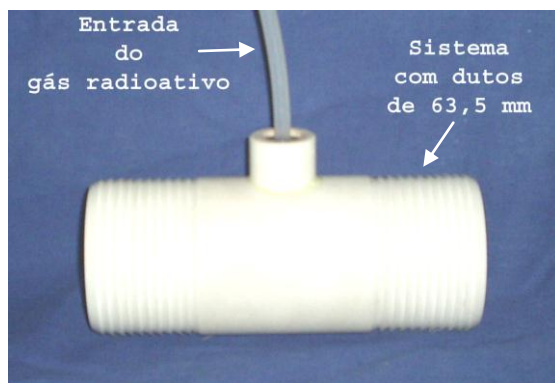
Figura III.11 – Sistema Injetor da Unidade Compacta de Produção de Radiotraçadores Gasosos.
