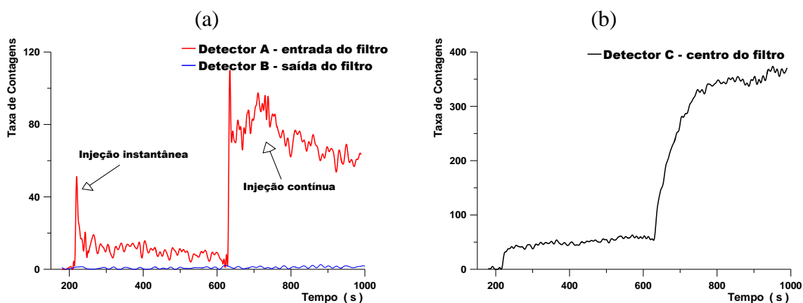
Figura IV.11 – Curvas de resposta dos três detectores, após injeções instantânea e contínua: (a) A e B; (b) C.
