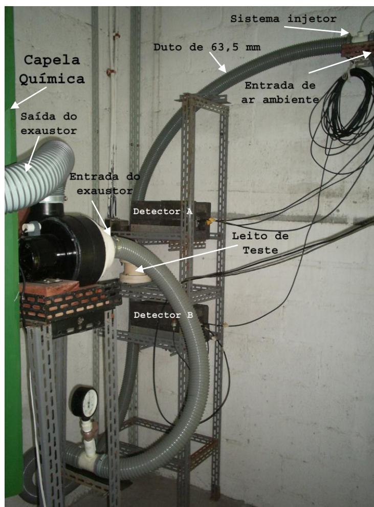
Figura III.13 – Protótipo experimental para a condução do ar ambiente.
