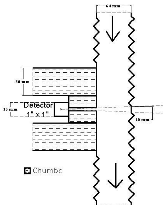
Figura III.18 – Quarta configuração: colimadores com 50 mm de espessura de chumbo e 5 mm de abertura.
