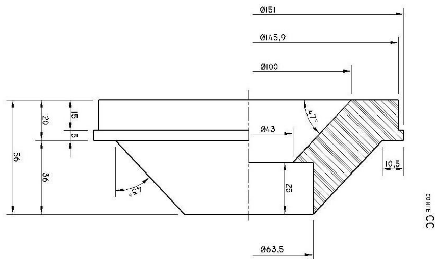
Figura III.9 – Peça D: Cone redutor do exaustor.
