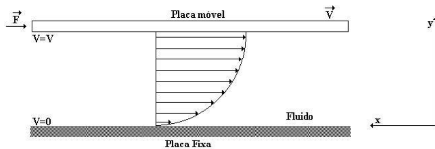
Figura D3 – Experiência das duas placas planas.
