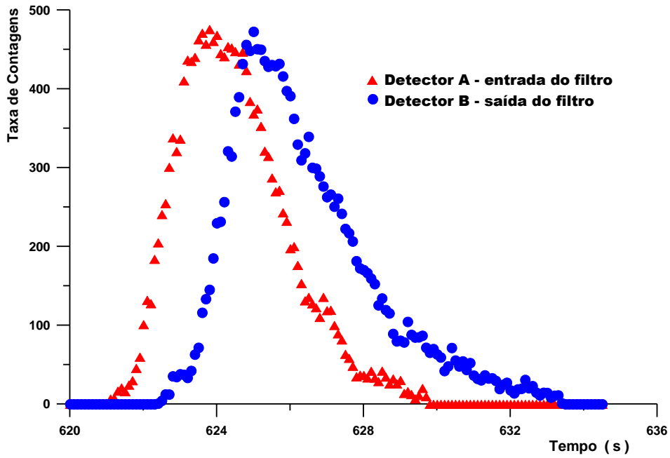
Figura IV.3 – Curvas de resposta dos detectores A e B para o filtro contendo 500 g de \text{SiO}_2 .
