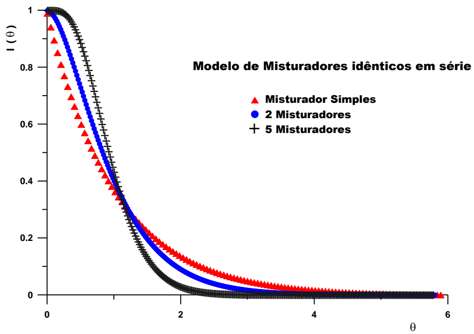
Figura II.10.3 – Função I(\theta) adimensional, para um fluxo com misturadores idênticos em série.
