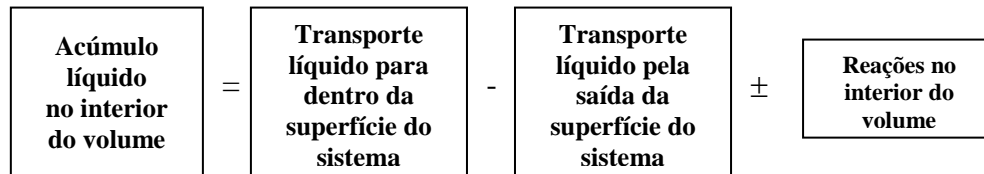
Figura II.3 – Fluxograma de balanço (massa, energia ou quantidade de movimento).
