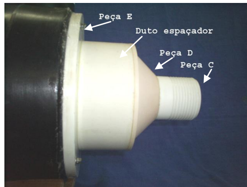
Figura III.8 – Foto da redução usada na conexão do exaustor à mangueira de PVC.
