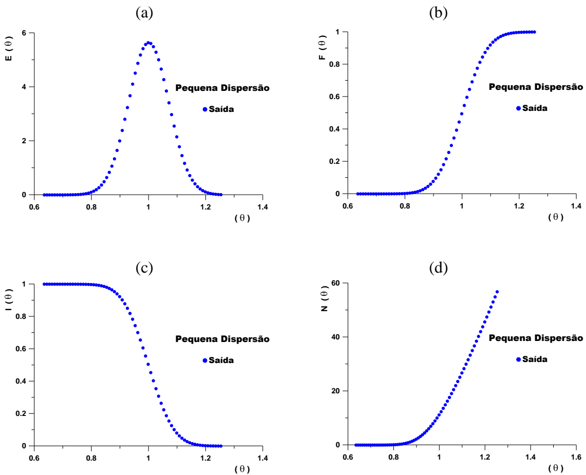
Figura II.8.1 – Funções de DTR adimensionais, para um fluxo dispersivo com pequena dispersão: (a) E(\theta) ; (b) F(\theta) ; (c) I(\theta) ; (d) N(\theta) .
