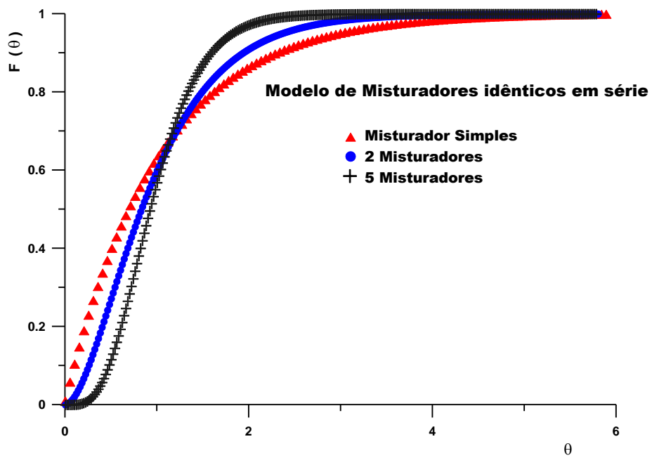
Figura II.10.2 – Função F(\theta) adimensional, para um fluxo com misturadores idênticos em série.
