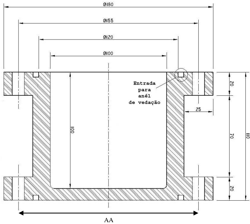
Figura III.4 – Peça A: Cilindro reto que acomoda o meio-poroso.
