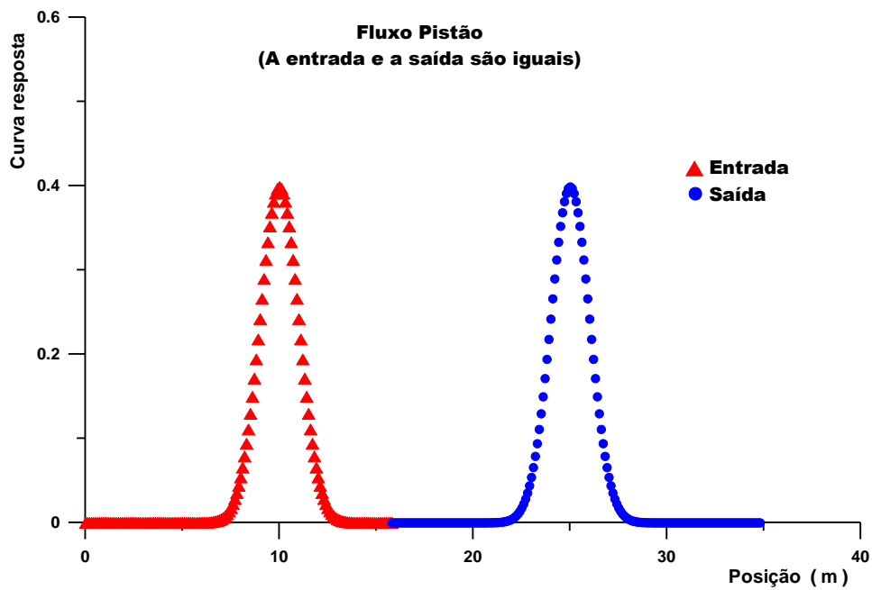
Figura II.7 – Curvas teóricas representando um fluxo pistão.
