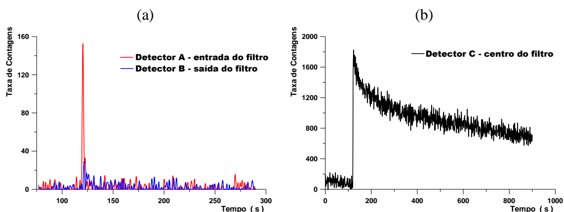
Figura IV.20 – Curva de resposta dos três detectores usados no teste de retenção do \text{CH}_3\text{I} por um filtro com 157 \text{ cm}^3 de carvão ativo: (a) A e B; (b) C.
