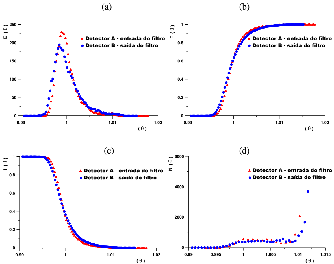
Figura IV.2.1 – Funções de DTR adimensionais, para o filtro contendo 250 g de \text{SiO}_2 : (a) E(\theta) ; (b) F(\theta) ; (c) I(\theta) ; (d) N(\theta) .
