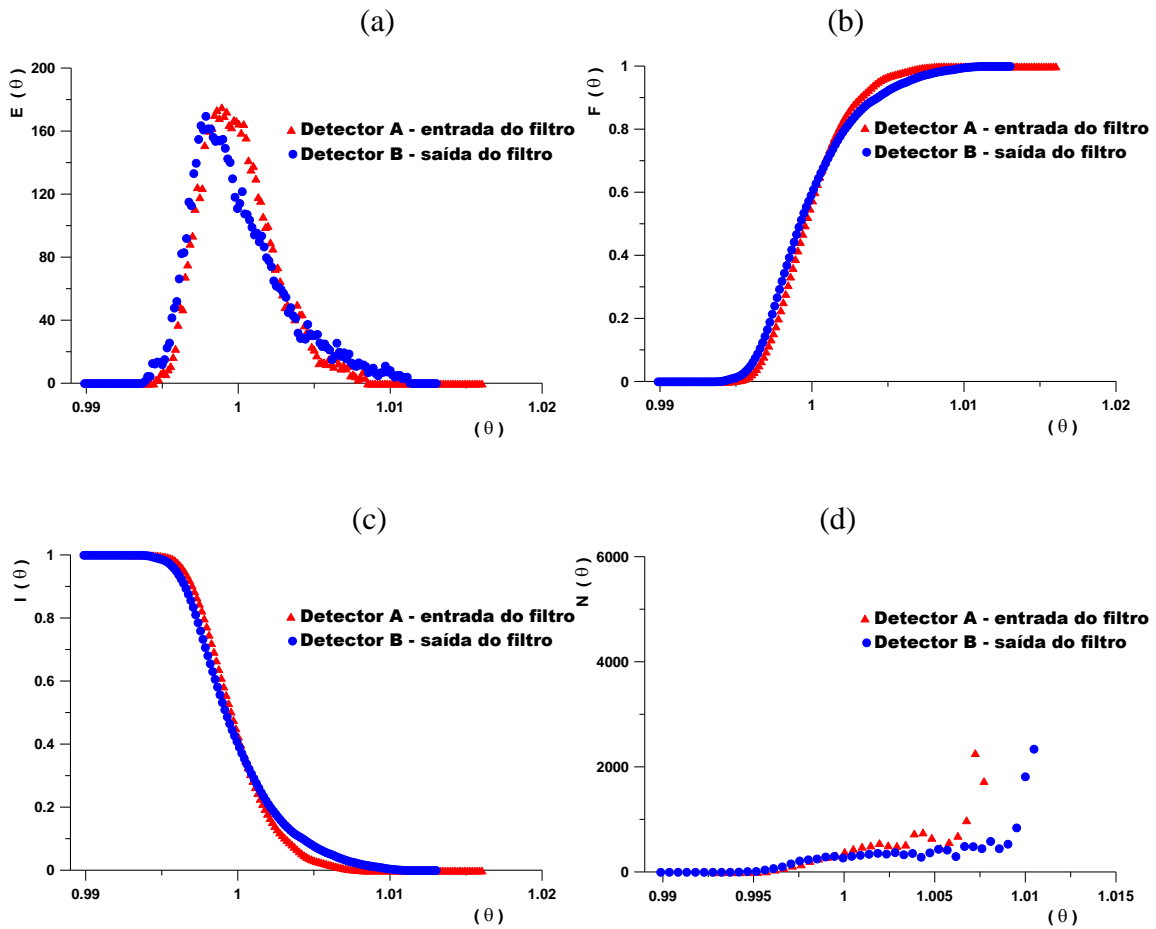
Figura IV.3.1 – Funções de DTR adimensionais, para o filtro contendo 500 g de \text{SiO}_2 : (a) E(\theta) ; (b) F(\theta) ; (c) I(\theta) ; (d) N(\theta) .
