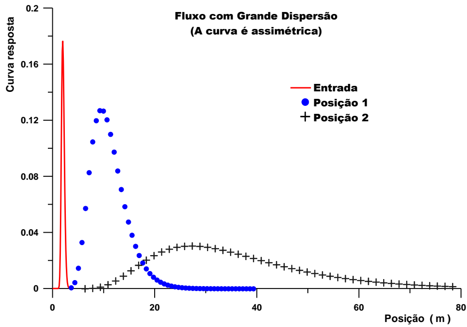
Figura II.9 – Curvas teóricas para um fluxo dispersivo com grande dispersão.
