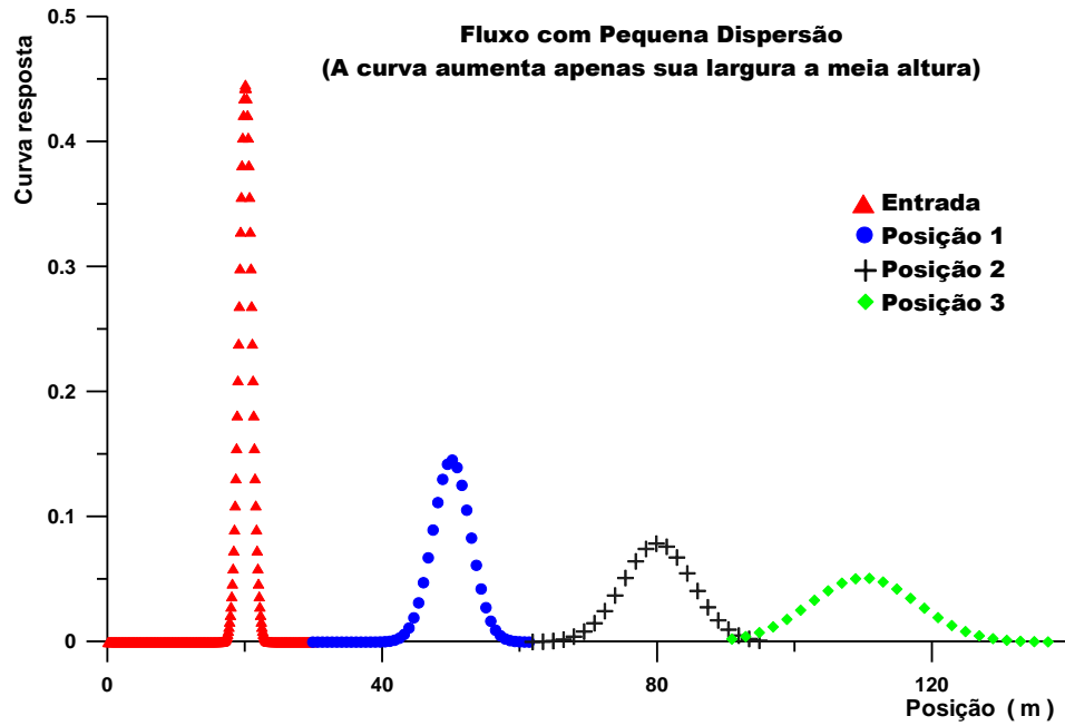
Figura II.8 – Curvas teóricas para um fluxo dispersivo com pequena dispersão.
