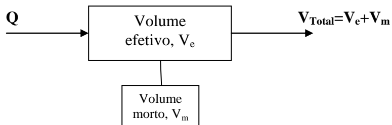
Figura II.11 – Representação esquemática de um fluxo com zona morta.
