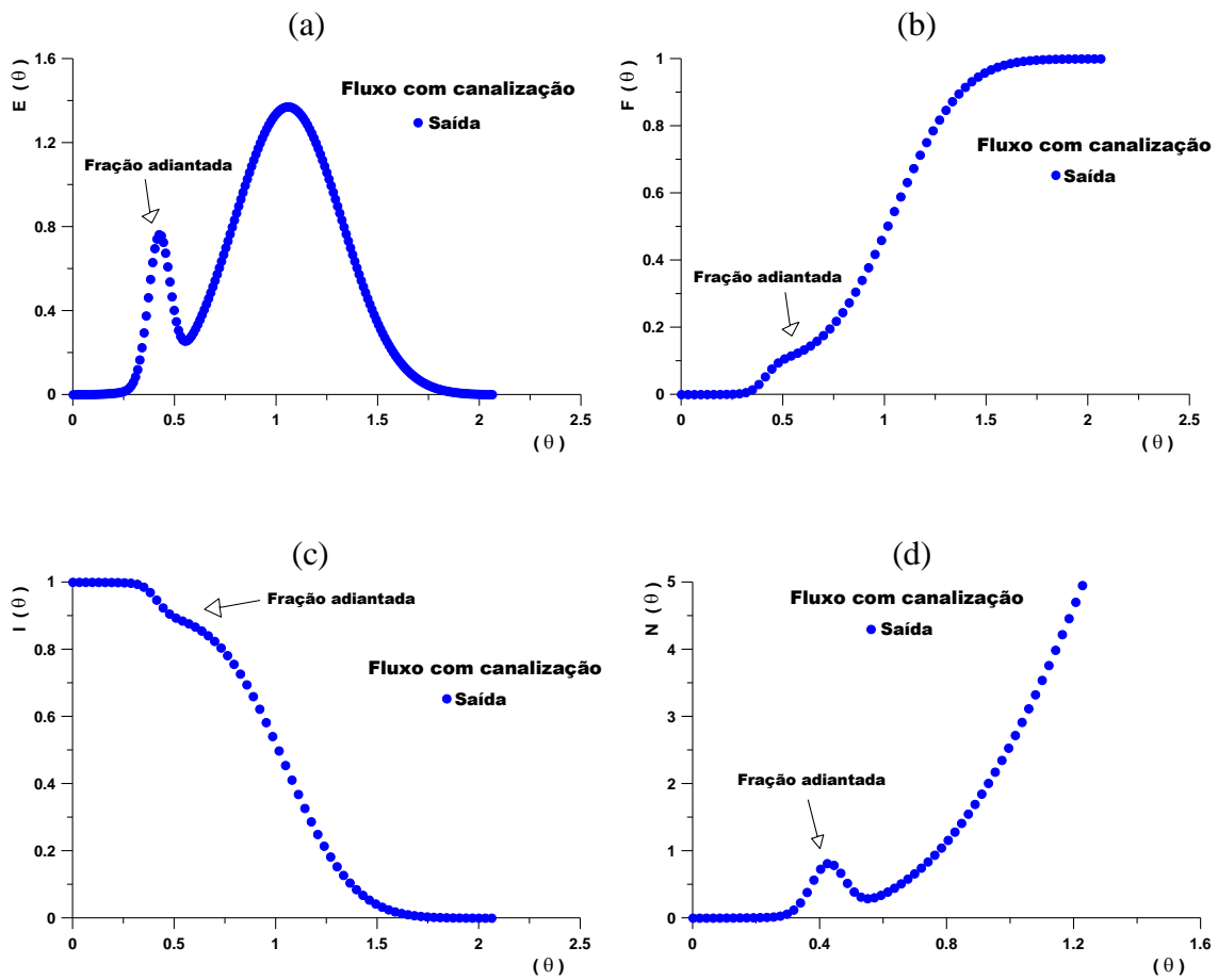
Figura II.14.1 – Funções de DTR adimensionais, para um fluxo com canalização: (a) E(\theta) ; (b) F(\theta) ; (c) I(\theta) ; (d) N(\theta) .
