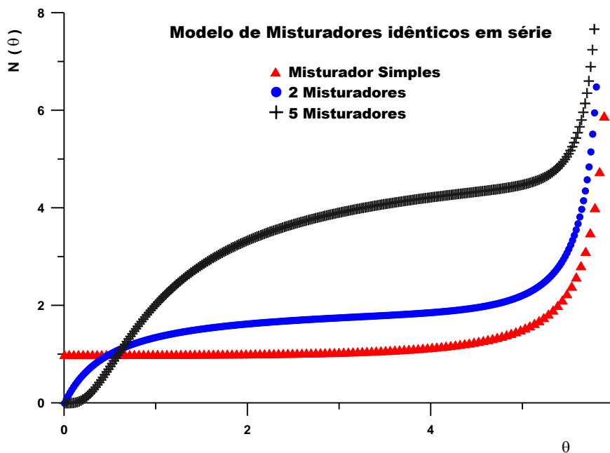
Figura II.10.4 – Função N(\theta) adimensional, para um fluxo com misturadores idênticos em série.
