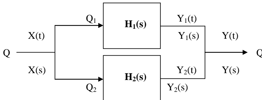
Figura II.20 – Subsistemas em paralelo.
