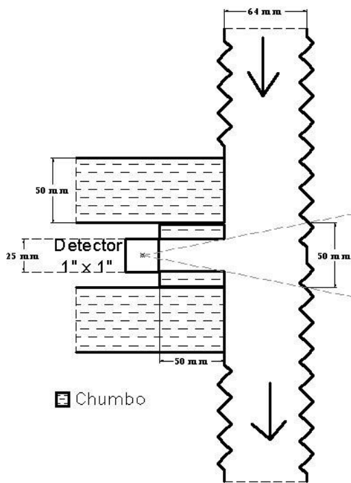
Figura III.17 – Terceira configuração: colimadores com 50 mm de espessura de chumbo e 25 mm de abertura.
