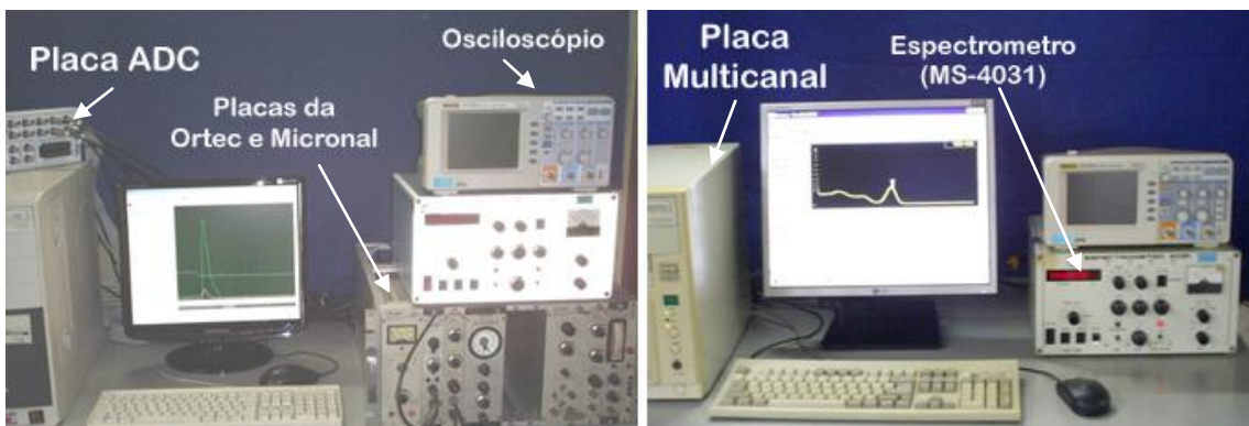
Figura III.2 – Conjunto de aquisição e análise de dados.
