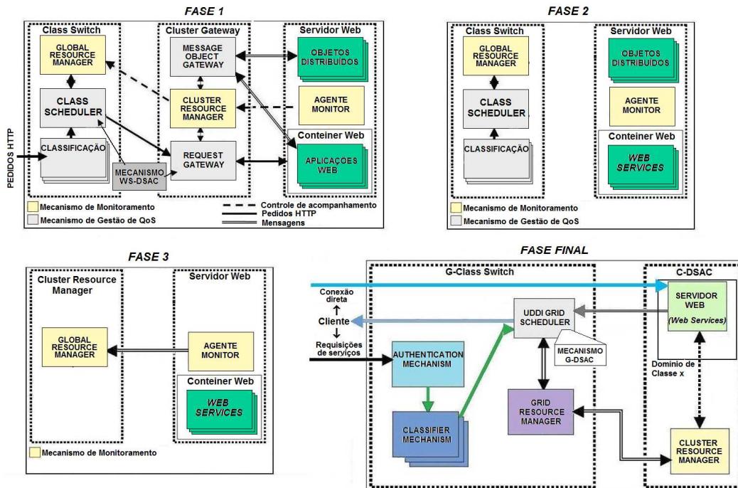
Figura 5.2: Transição da arquitetura WS-DSAC para arquitetura G-DSAC
