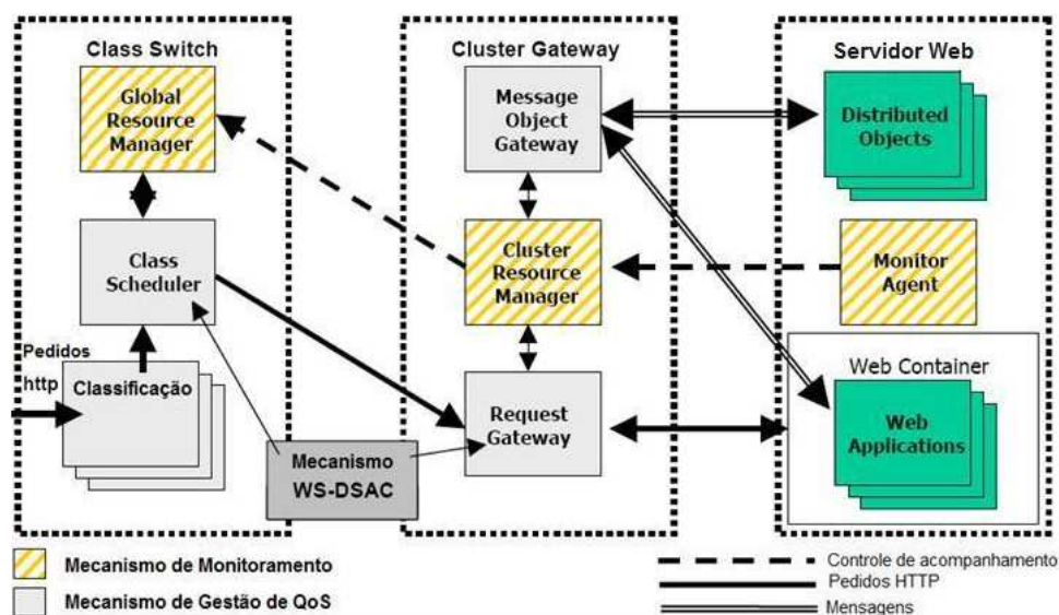
Figura 3.2: Componentes do mecanismo WS-DSAC
