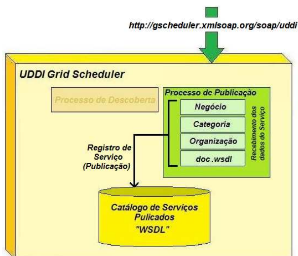
Figura 4.8: Processo de Publicação de Serviços
