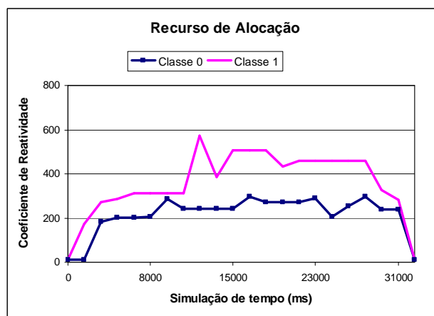
Figura 5.5: Comportamento da carga dos domínios de classes QoS “0” e “1” – Cluster 2
