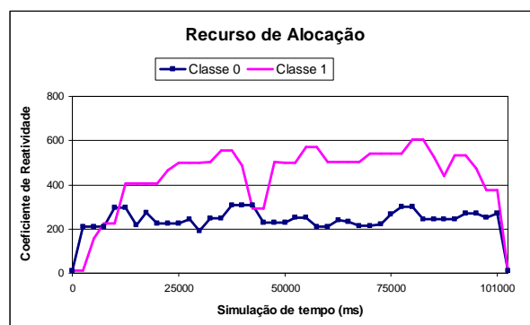
Figura 5.8: Comportamento da carga dos domínios de classes QoS “0” e “1” – Cluster 2
