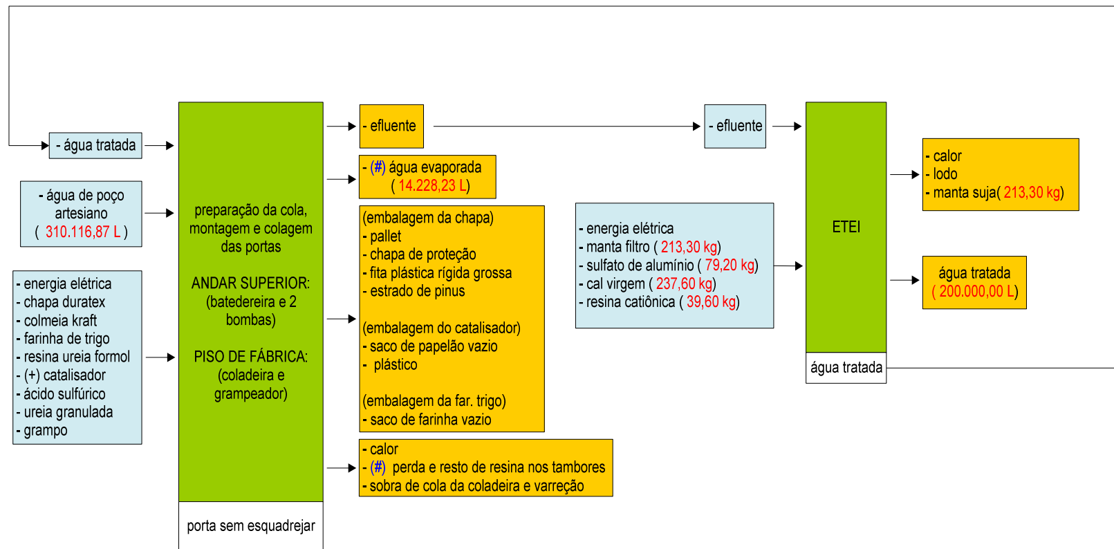
Figura 5.9. Balanço de material da oportunidade de redução da água gasta na painelaria – antes de P+L
