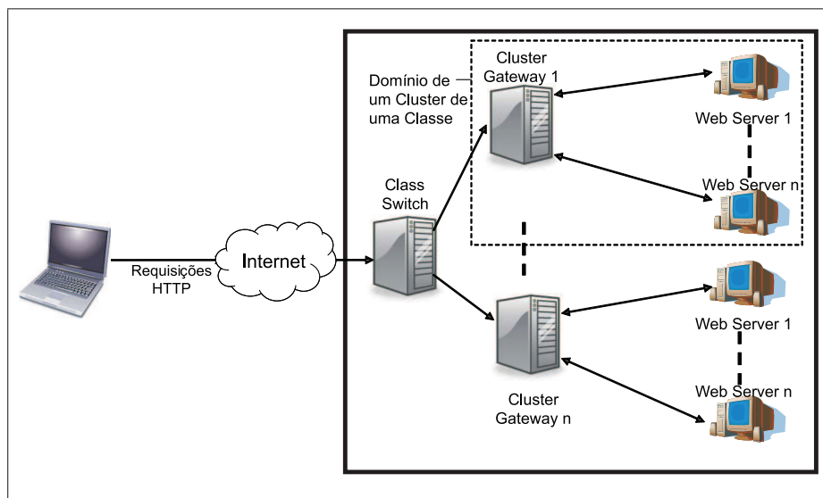
Figura 3.1: Visão geral da plataforma WS-DSAC.
