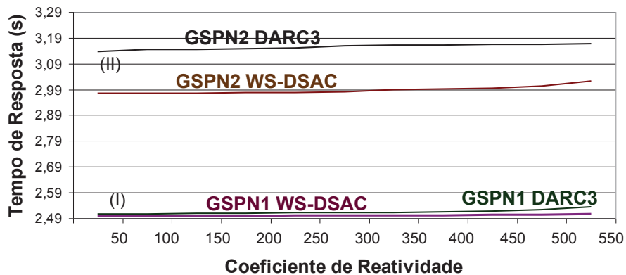
Figura 5.23: Tempo de Resposta: DARC-3 e WS-DSAC.
