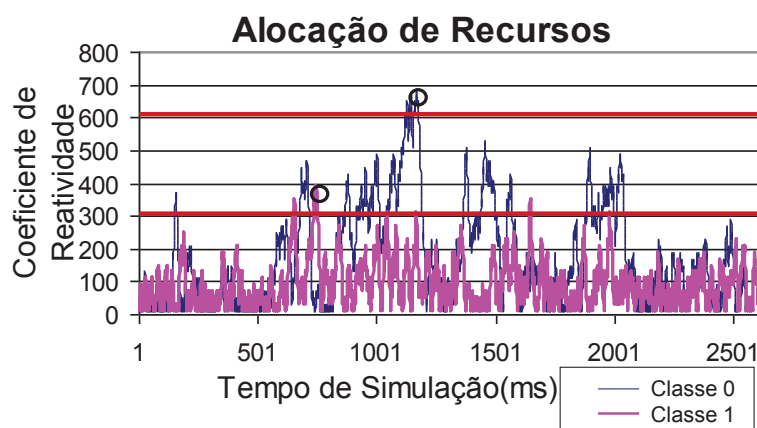
Figura 5.12: Alocação de Recursos com carga nativa da classe 0 com a Arquitetura DARC, com percentual de monitoramento de 85% (DARC3-sim).
