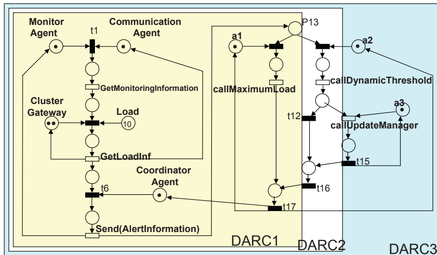
Figura 5.19: GSPN para DARC-1, DARC-2 e DARC-3.
